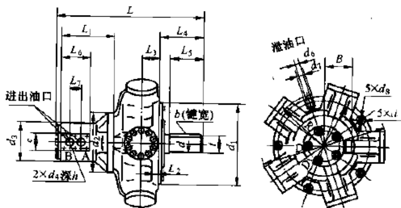
图2 1JMD-63~125型液压马达外形及安装尺寸
