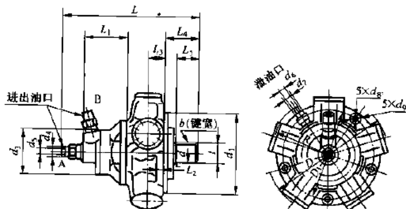
图 1 LJMD-40 型液压马达外形及安装尺寸
