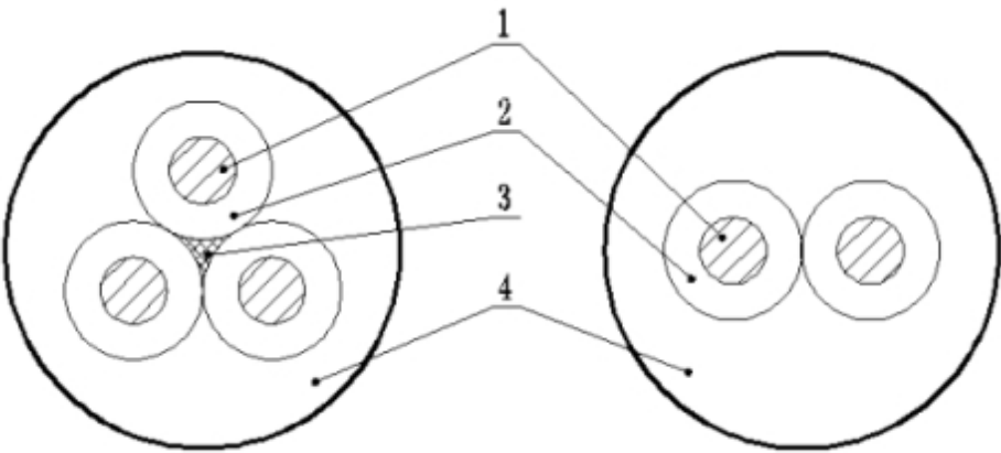
1-导体；2-绝缘；3-填充；4-护套
