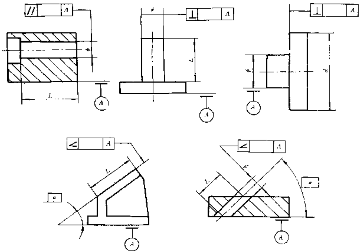
主参数 L, d (D) 图例
