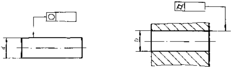
主参数 d(D) 图例
