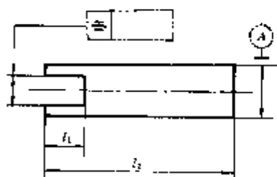
a) 基准:较长要素( l_2 )
