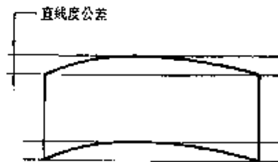
平行度误差 \leq 直线度公差
