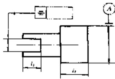
b) 基准:较长要素( l_1 )
