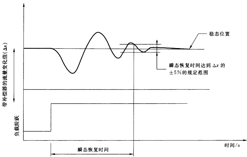
a) 对阶跃输入的瞬态响应
