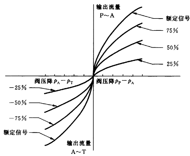
图 8 输出流量-阀压降特性曲线(不带内置式压力补偿)
