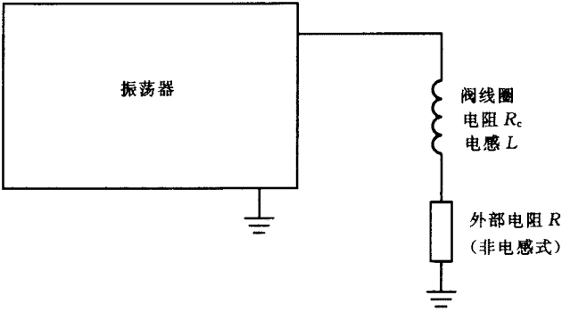
a) 电感试验
