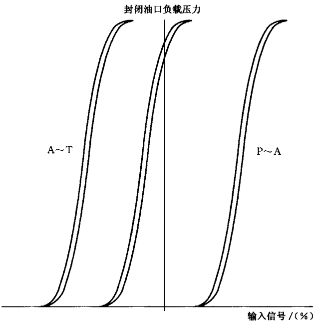
图 12 封闭油口负载压力-输入信号特性曲线
