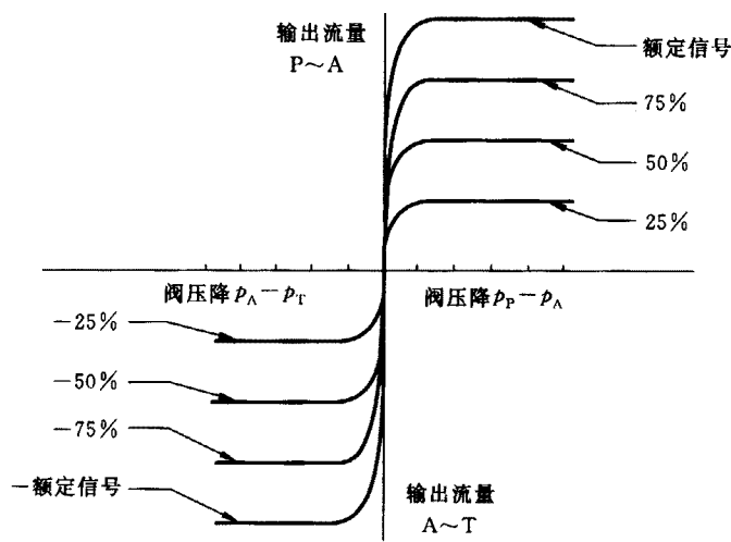
图 9 输出流量-阀压降特性曲线(带内置式压力补偿)
