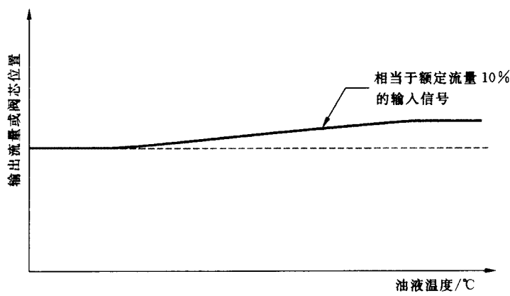
图 11 输出流量-油液温度特性曲线
