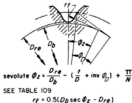
FIG. 36—FILLET FOR FILLET ROOT EXTERNAL SPLINE
