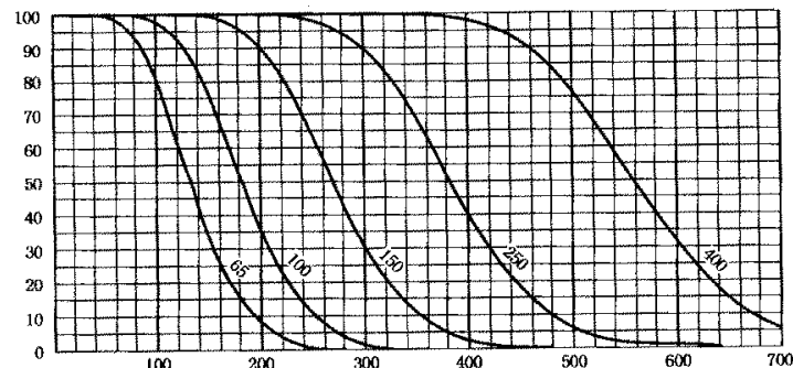
图 D 一次抽样方案的抽检特性曲线 (二次和多次抽样方案的抽检特性曲线尽可能与其紧密匹配)
