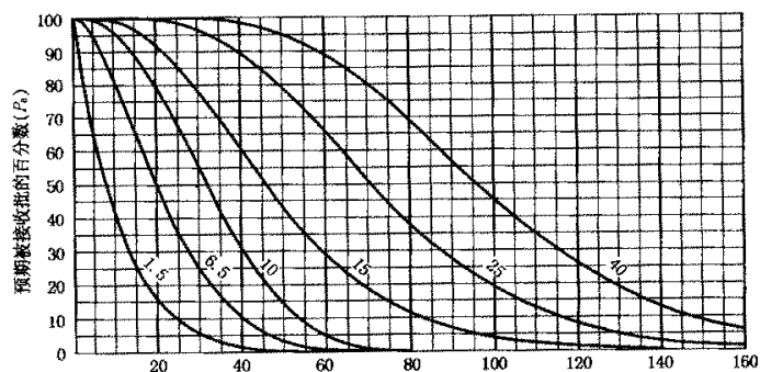
图 D 一次抽样方案的抽检特性曲线 (二次和多次抽样方案的抽检特性曲线尽可能与其紧密匹配)
