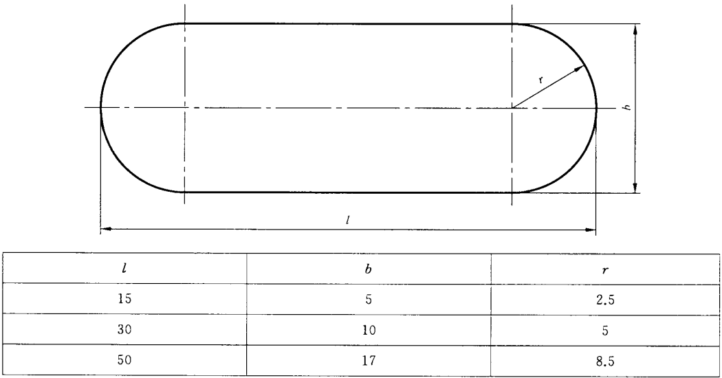
图 2 推荐标牌尺寸
