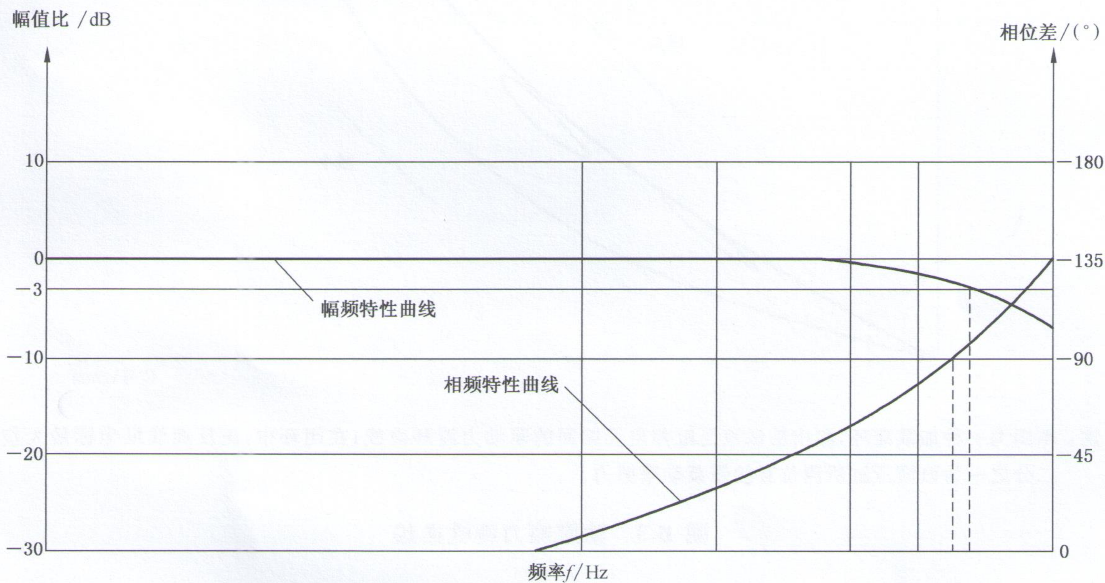
图 B.1 频率响应特性曲线
