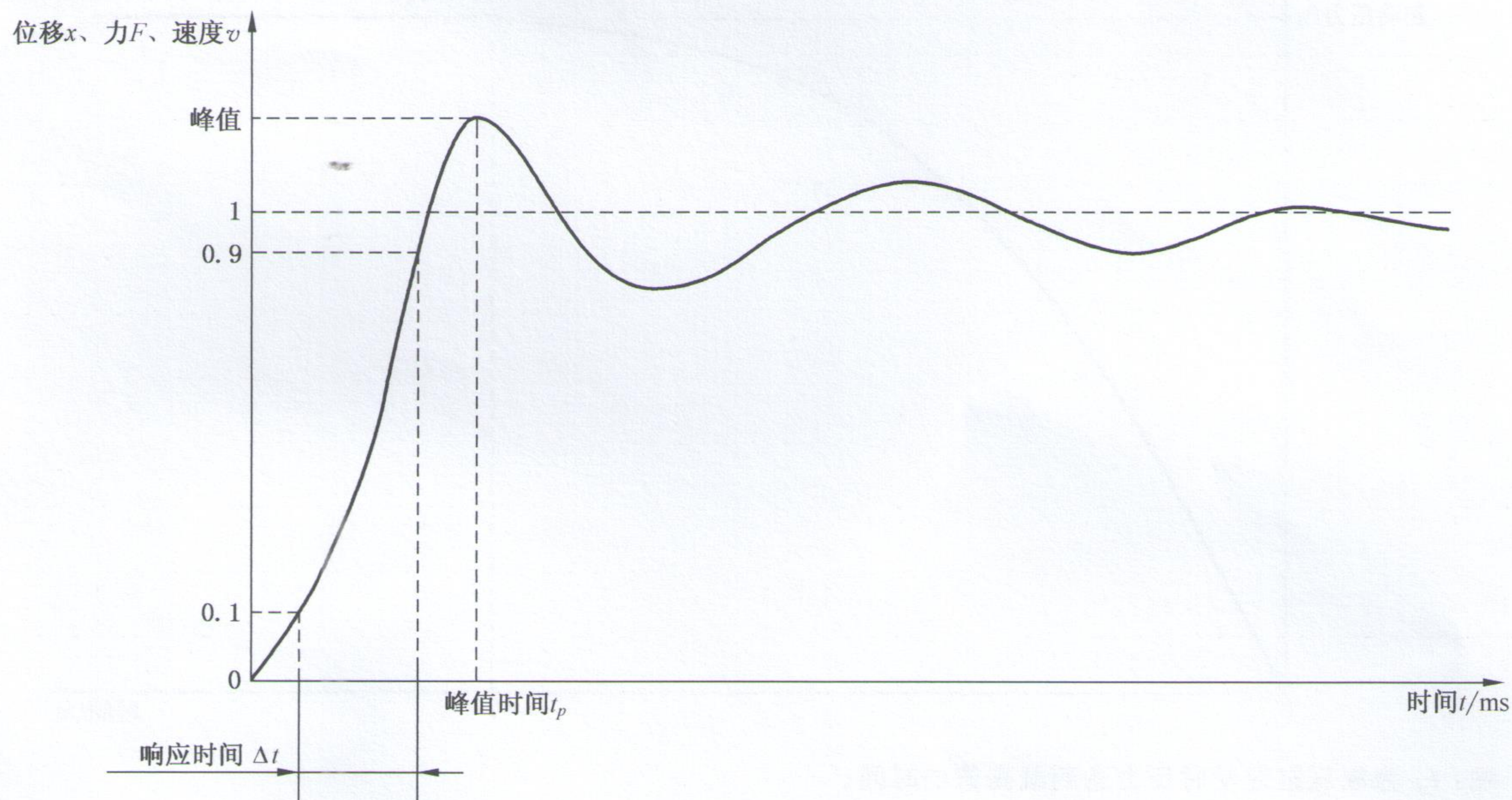
图 B.2 阶跃响应特性曲线
