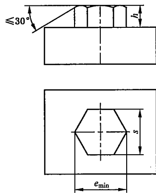
图 4 六角试棒
