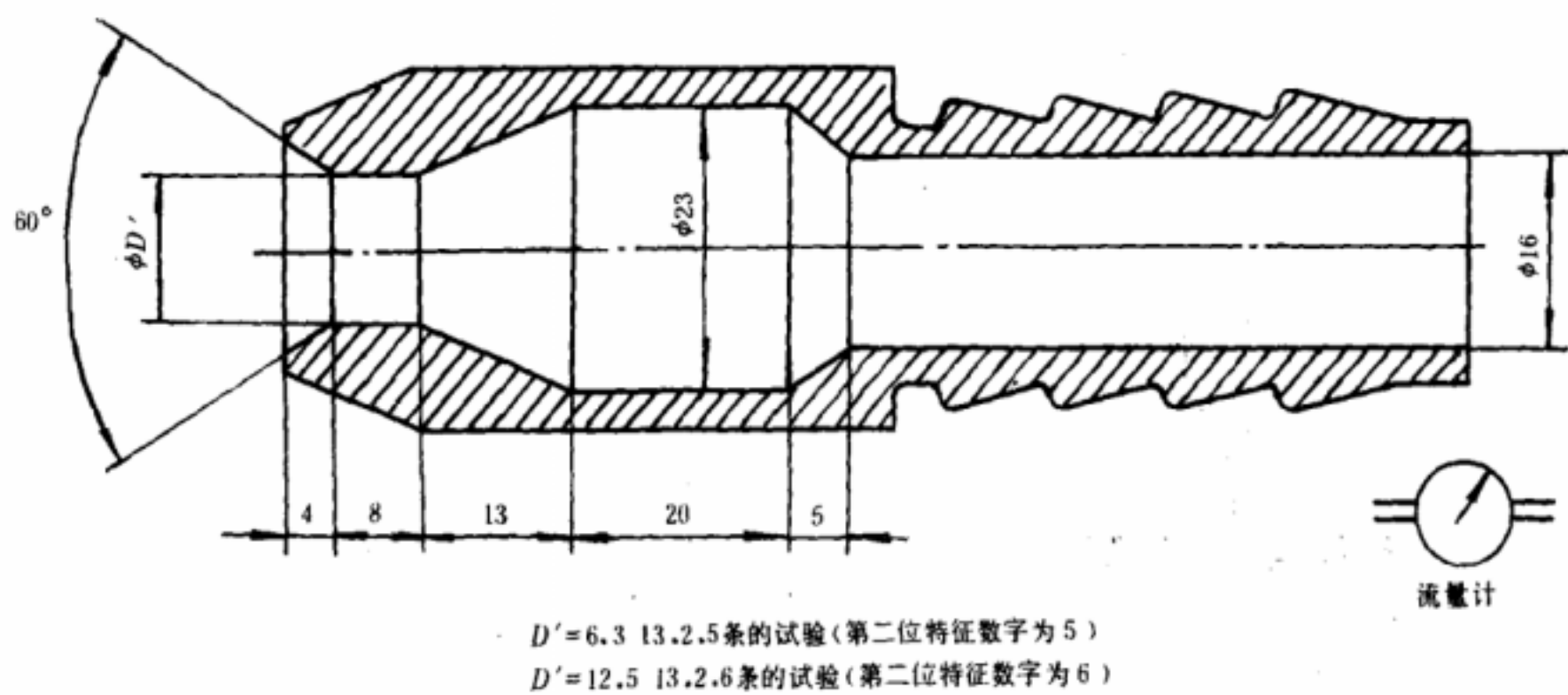
图 6 检验防喷水试验装置(软管喷嘴)
