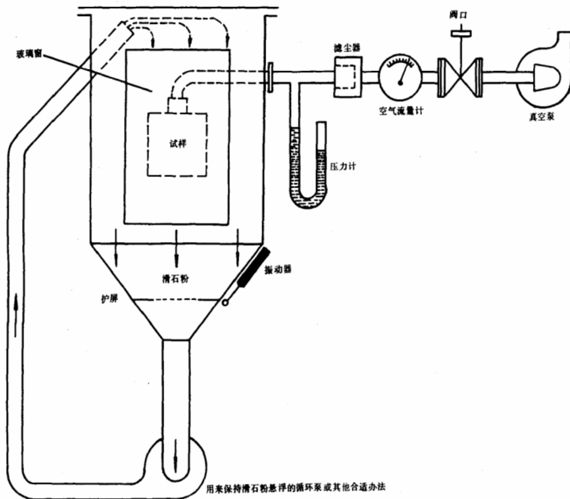
图 2 检验防尘试验装置(防尘箱)
