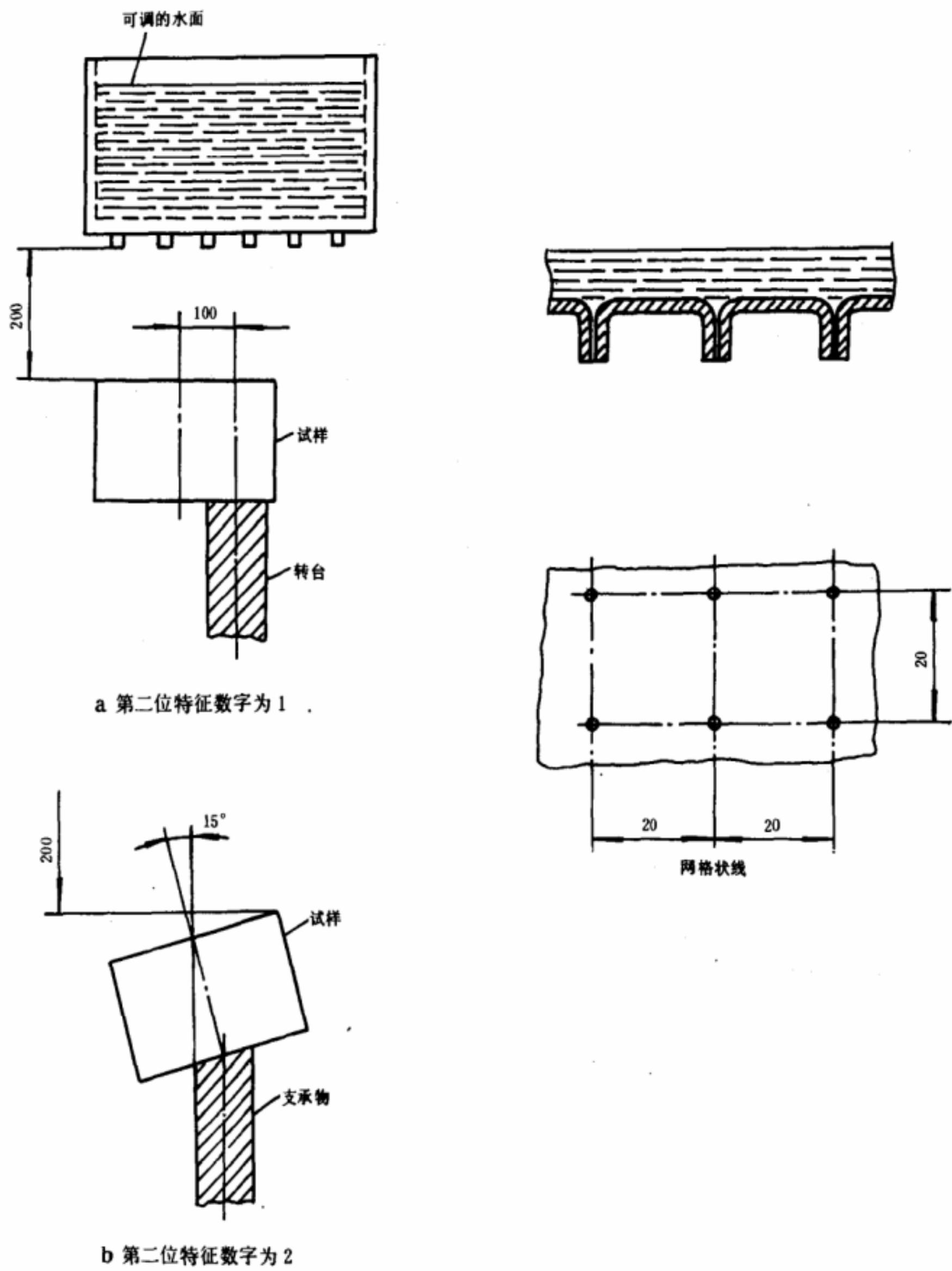
图 3 检验防垂直滴水试验装置(滴水箱)
