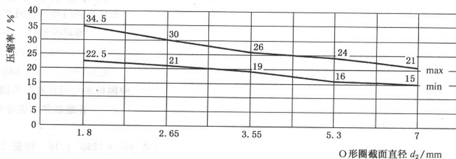
图 A.4 轴向密封
