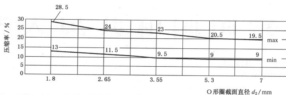
图 A.1 液压动密封
