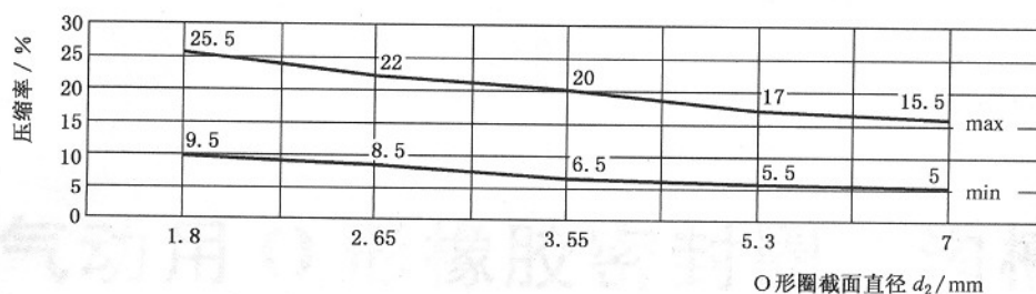
图 A.2 气动动密封
