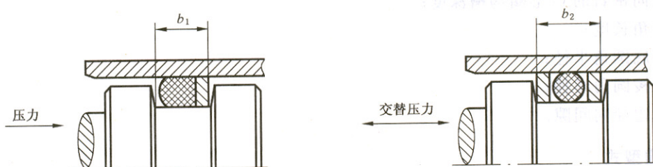
图 3 径向密封带挡圈密封沟槽型式
