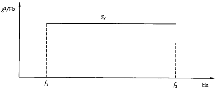
图 4 振动控制仪随机信号的检验谱形设置
