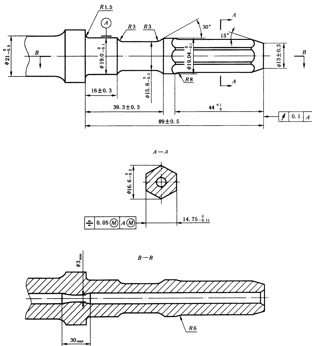
图 13 插孔钻用六角形尾柄
