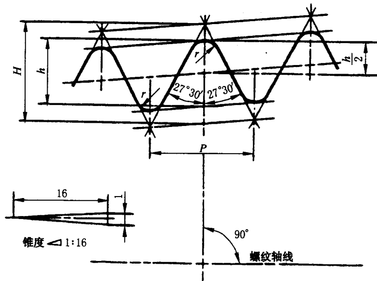
图 1 圆锥螺纹的设计牙型
