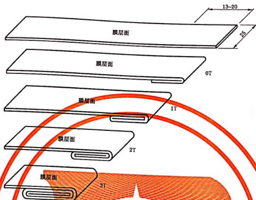
图 1 T弯过程示意图
