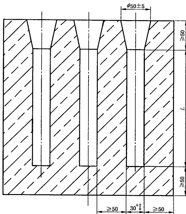
图 1 单铸试棒铸型
