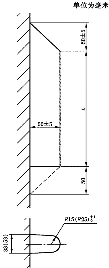
图 3 附铸试块
