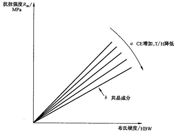
图 B.2 铸铁抗拉强度和硬度比关系(T/H 比)
