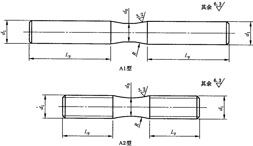
图 5 A 型试样
