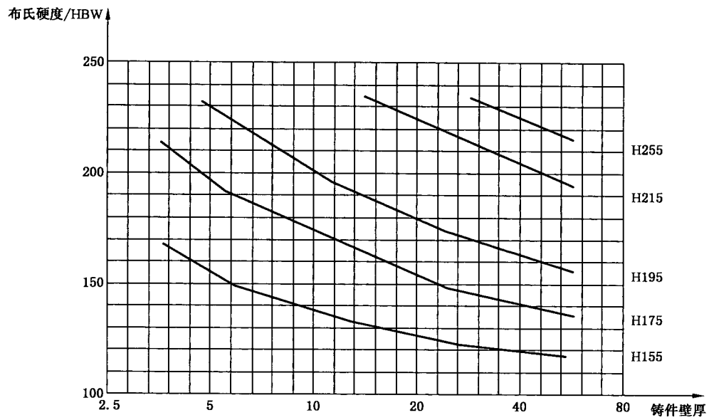
图 C.2 形状简单铸件的平均硬度和主要壁厚之间的关系
