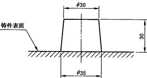
图 4 布氏硬度试块
