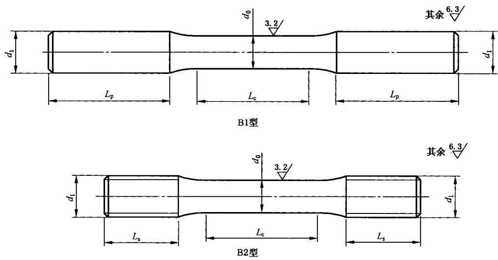
图 6 B 型试样
