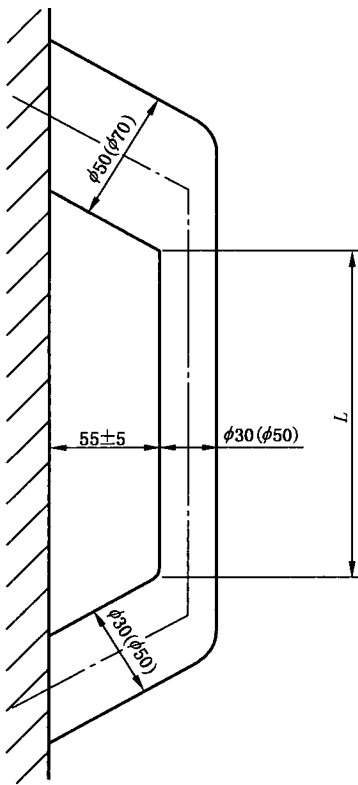
图 2 附铸试棒
