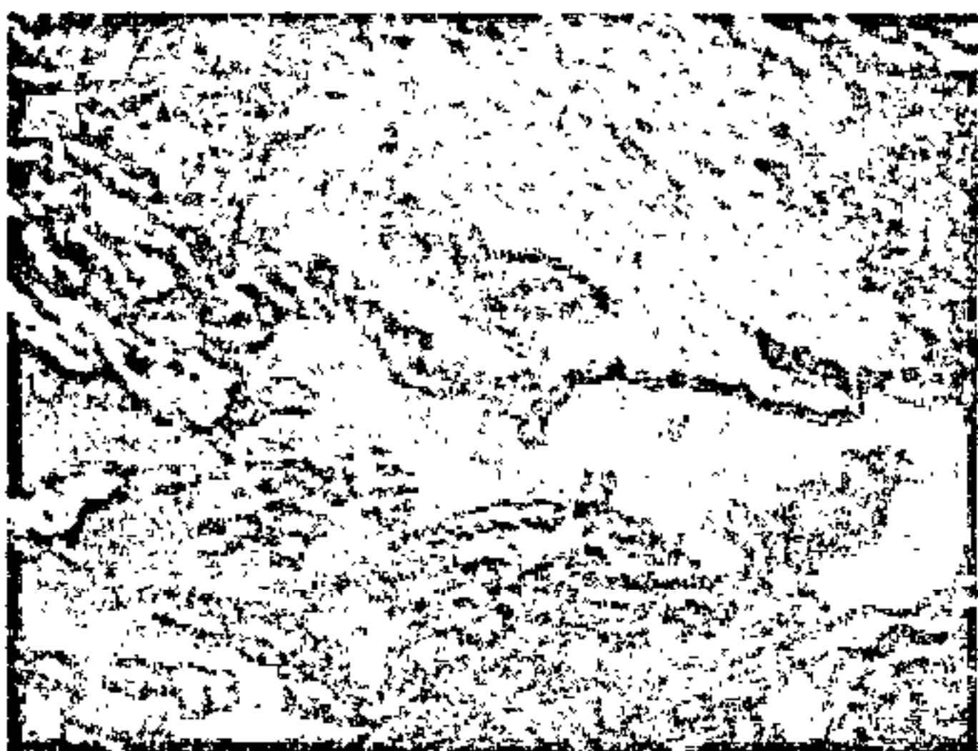
图 12 1060(L2)铝铸轧板横向显微组织 阳极制膜偏光 ×100
