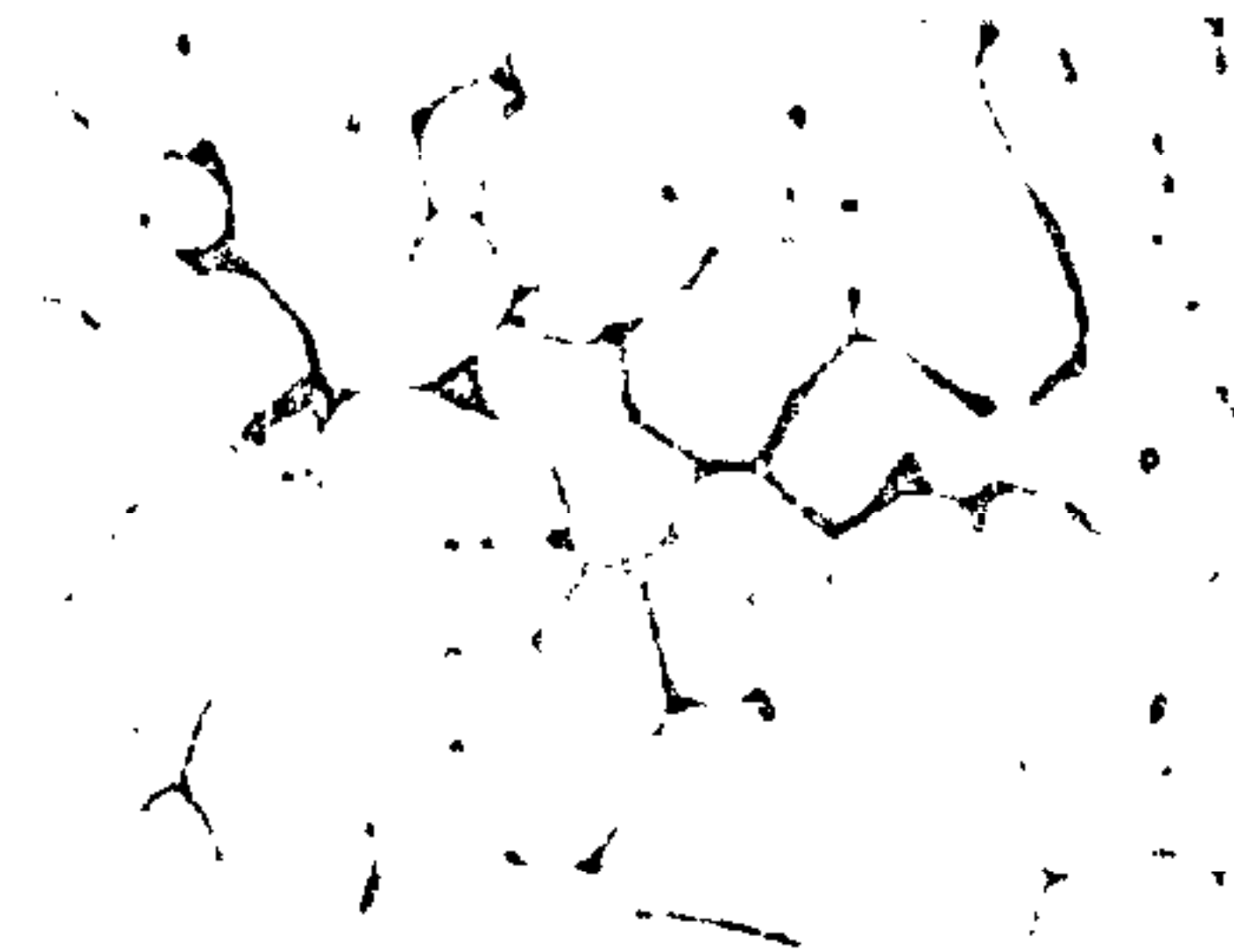
图7 7A04(LC4)合金铸锭枝晶网组织 3号浸蚀剂浸蚀 \times 250
