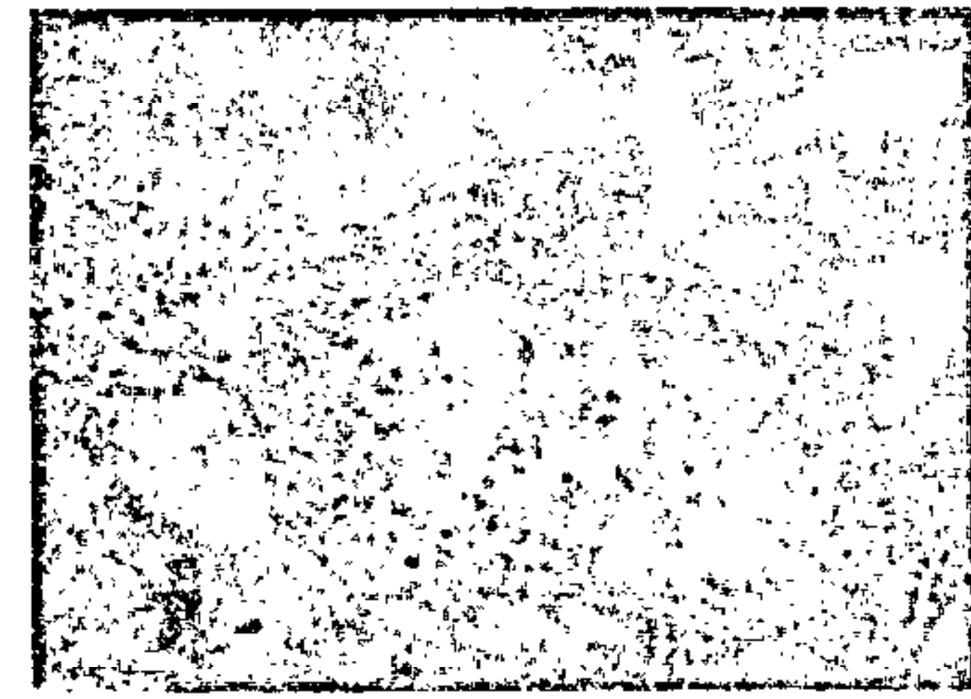
图 21 6063(LD31)合金型材风冷淬火正常组织 3号浸蚀剂浸蚀 ×200
