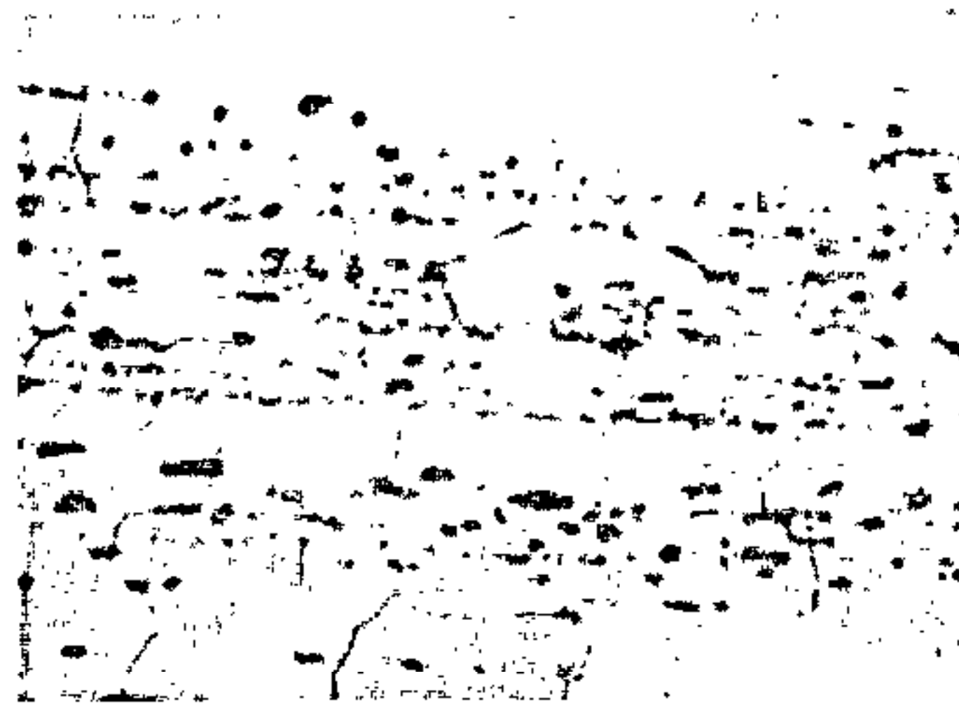
图 20 2A70(LD7)合金锻件淬火过烧组织 3号浸蚀剂浸蚀 ×200
