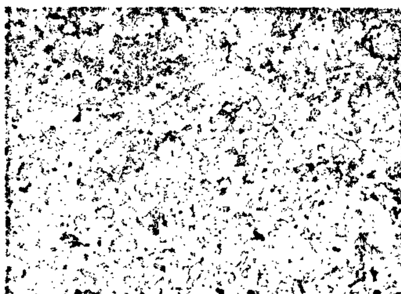
图 15 2A12(LY12)合金棒材淬火正常显微组织 3号浸蚀剂浸蚀 ×250
