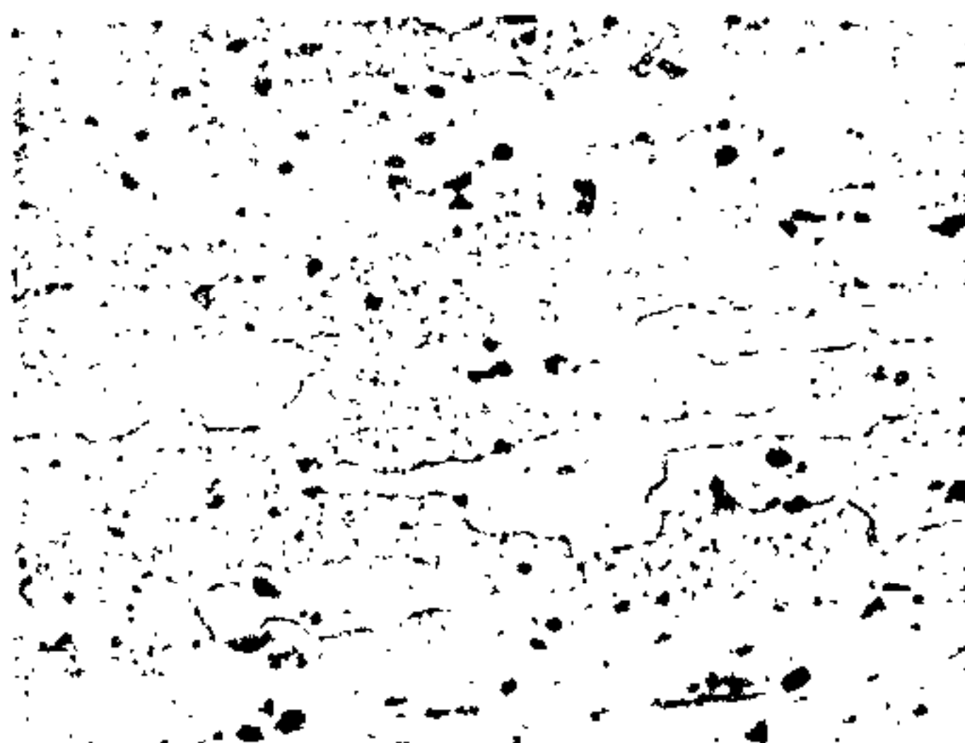
图 13 2A12(LY12)合金板淬火正常组织 3号浸蚀剂浸蚀 ×200
