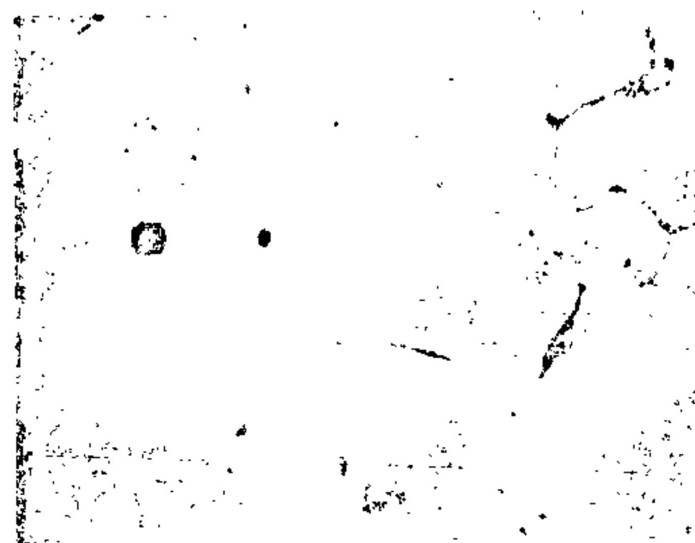
图8 7A04(LC4)合金铸锭均匀化处理过烧 3号浸蚀剂浸蚀 \times 250
