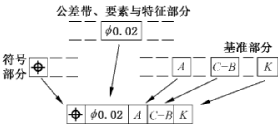
图 12 公差框格的三个部分
