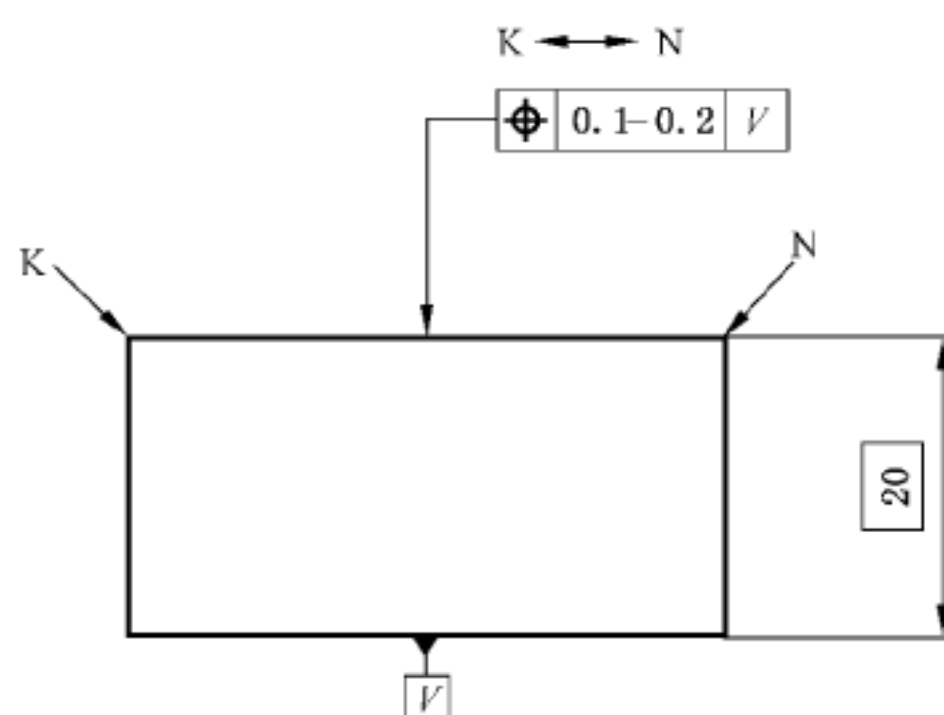
图 14 线性变化的公差带规范
