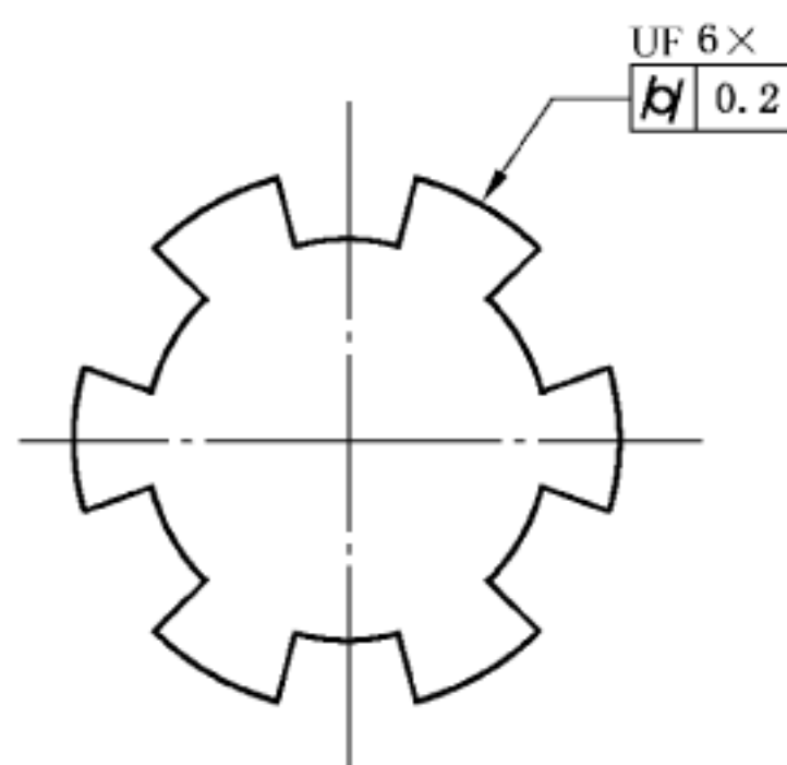
图 48 应用于联合要素的规范标注
