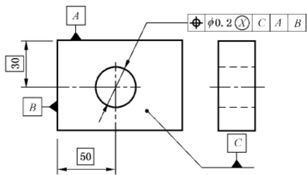
图 33 最大内切拟合被测要素——图样标注
