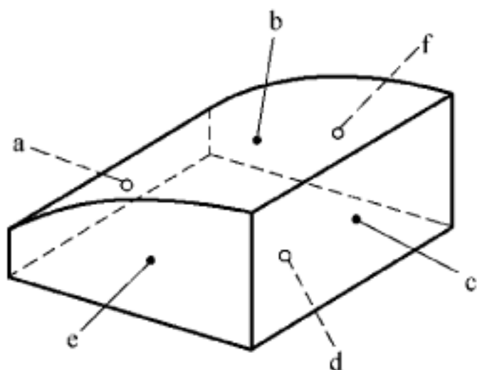
说明：图样上所标注的要求作为单独要求适用于四个面要素 a、b、c 与 d。 注：全周符号不包括面要素 e 与 f。
