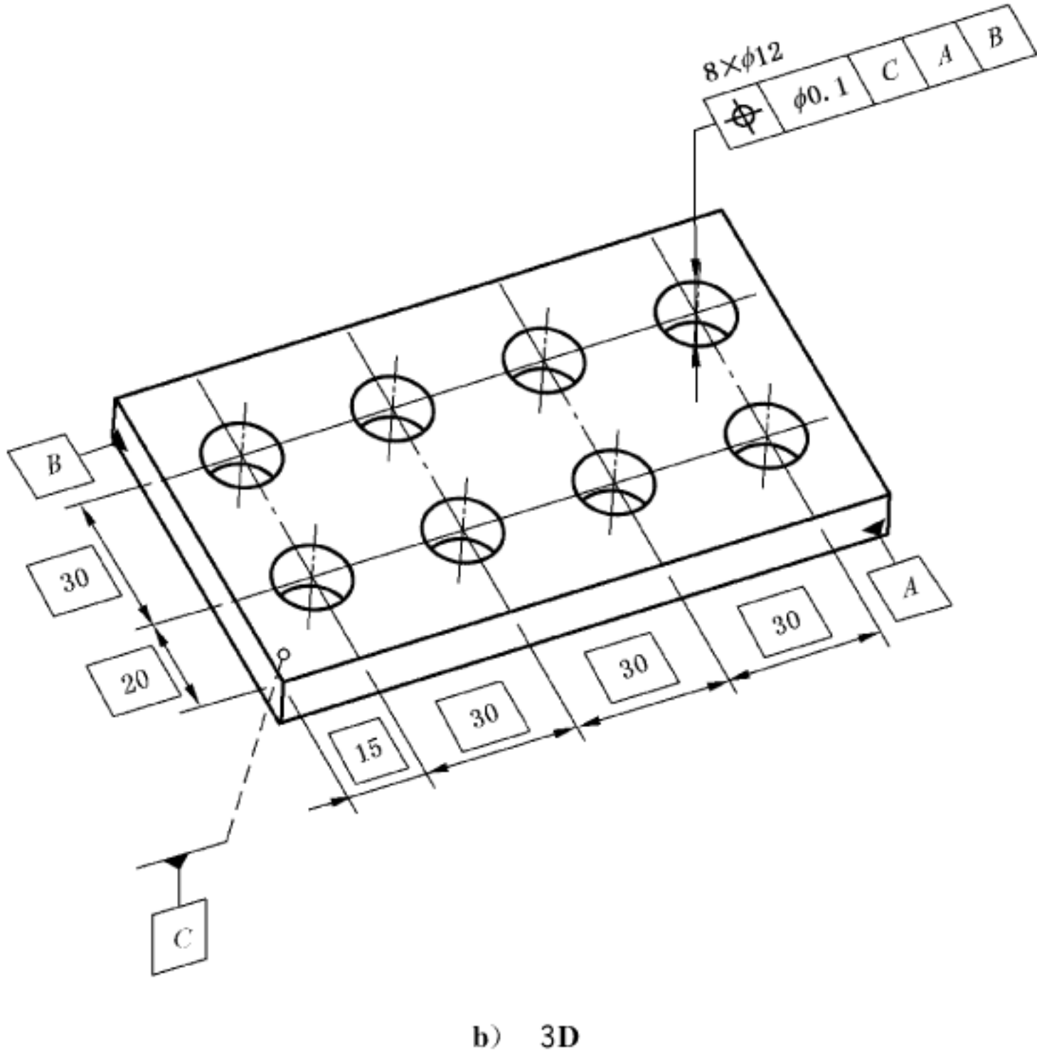
图 155 位置度标注
