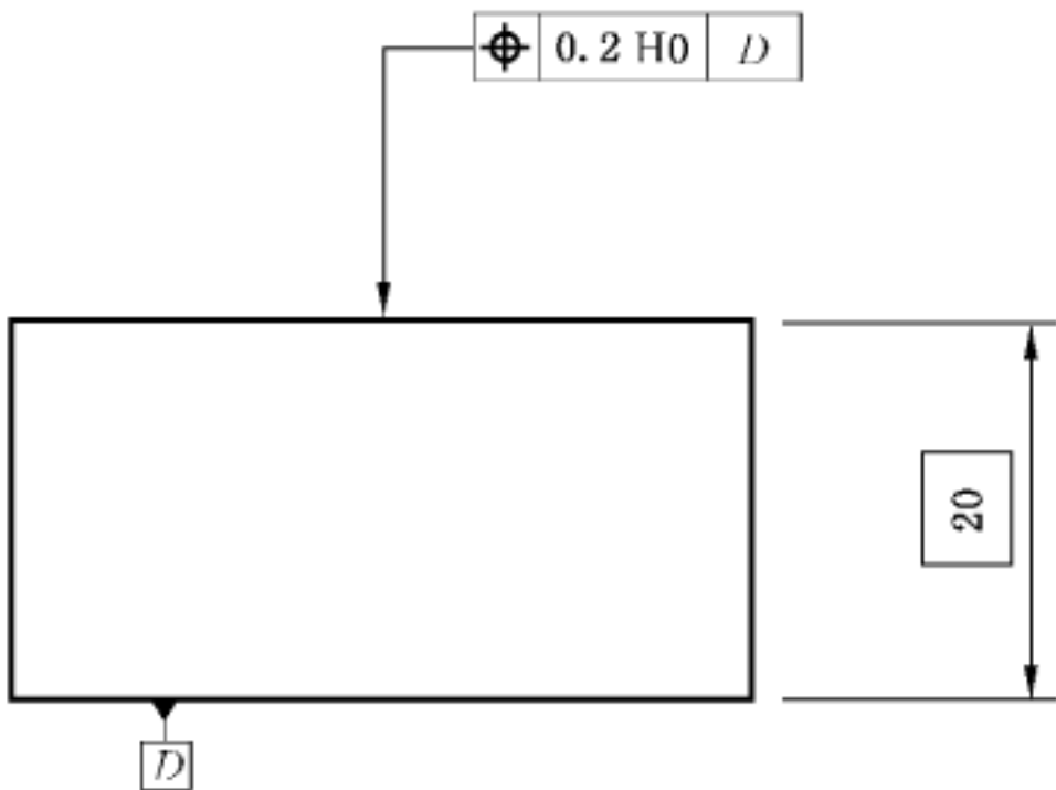
图 E.18 位置度公差示例
