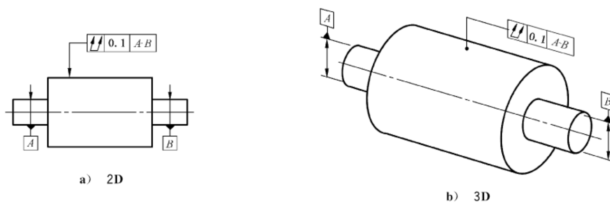
图 184 全跳动标注
