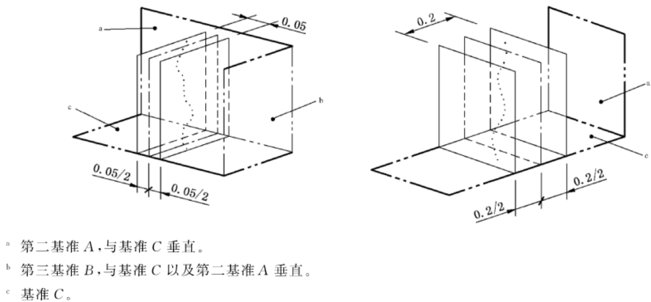
图 153 位置度公差带的定义
