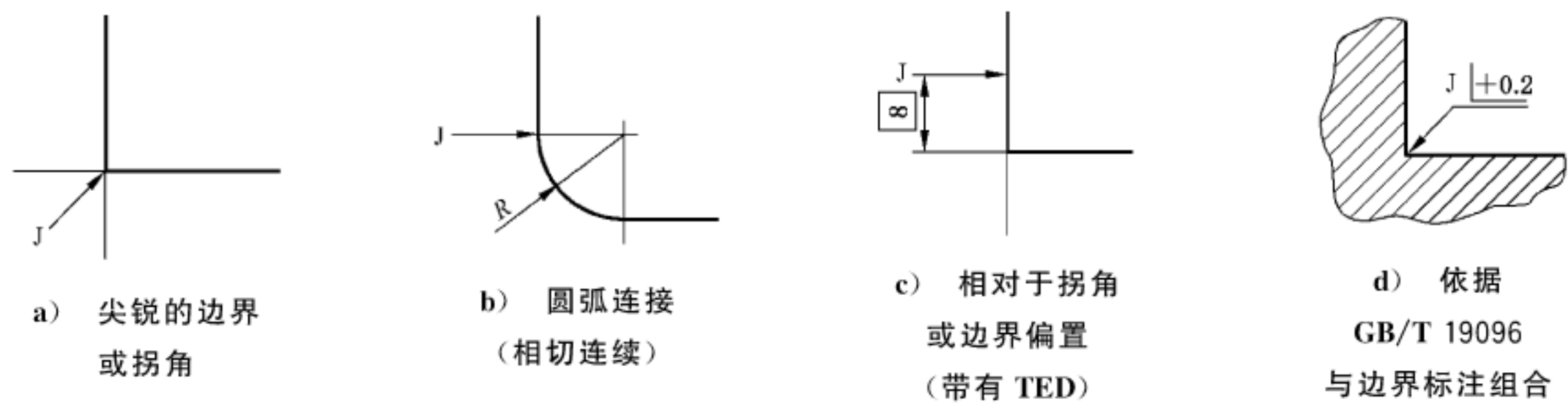
图 62 要素界限的标注
