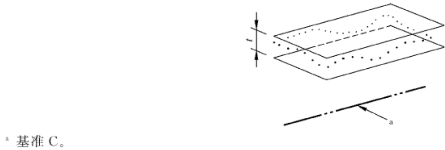
图 125 平行度公差带的定义
