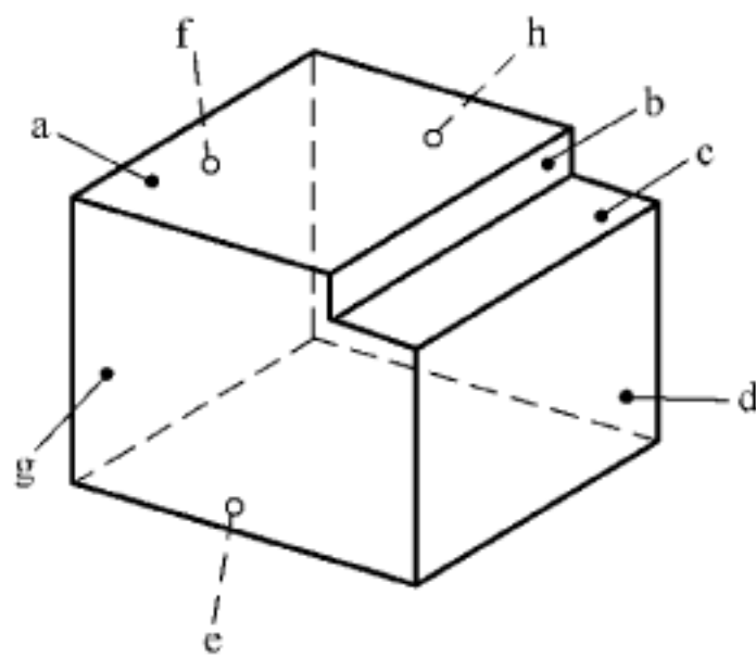
说明：该要求适用于所有的面要素 a、b、c、d、e、f、g、h，并将其视为一个联合要素。
