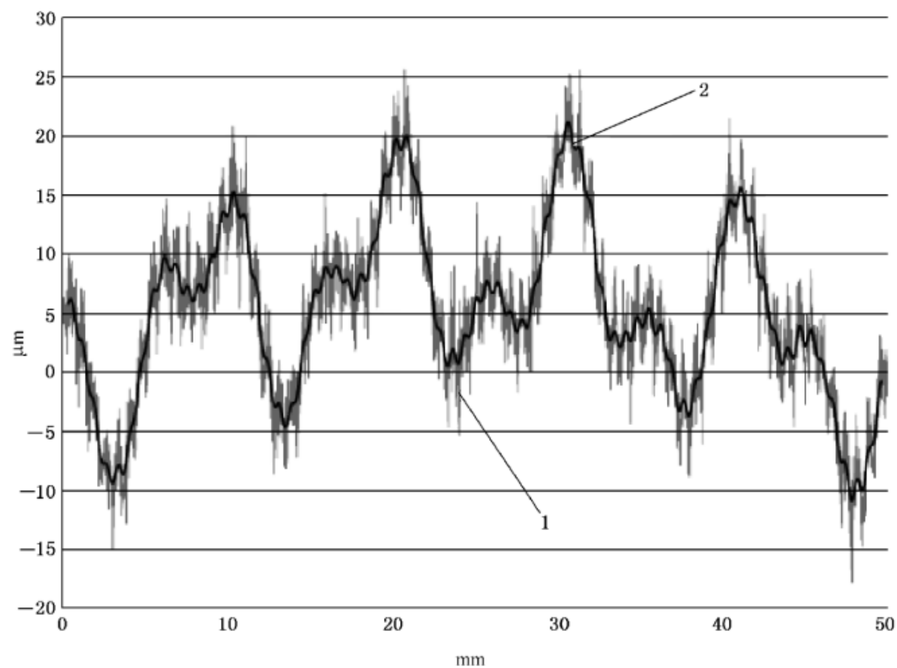
a) 0.8 mm 的长波通高斯滤波器
