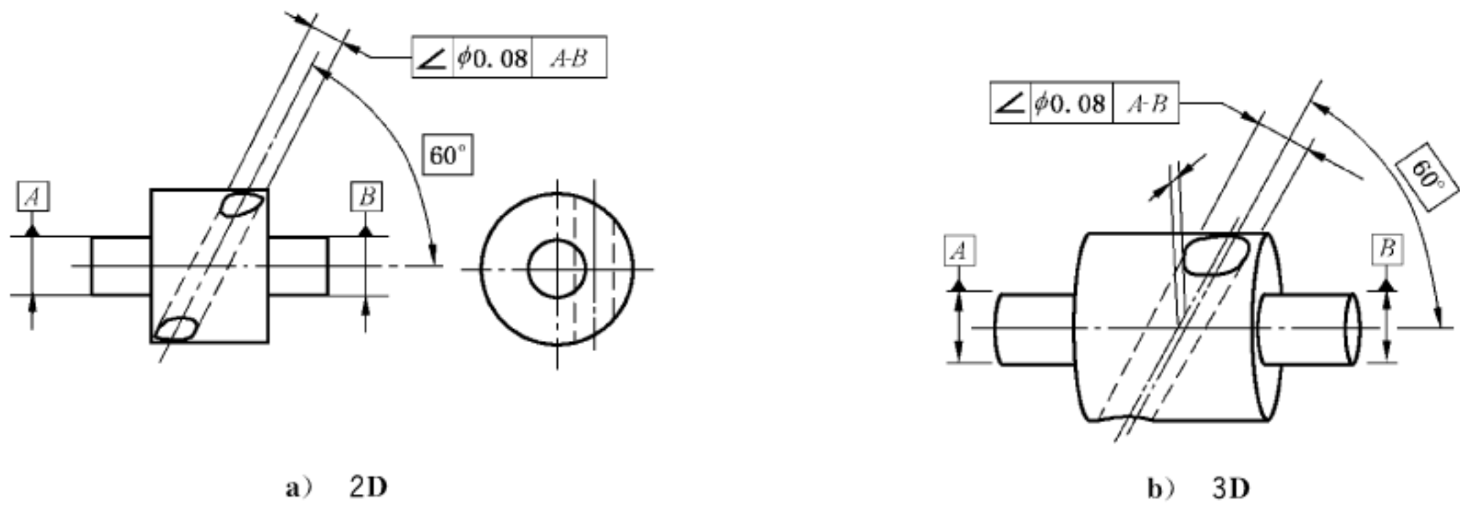
图 140 倾斜度标注
