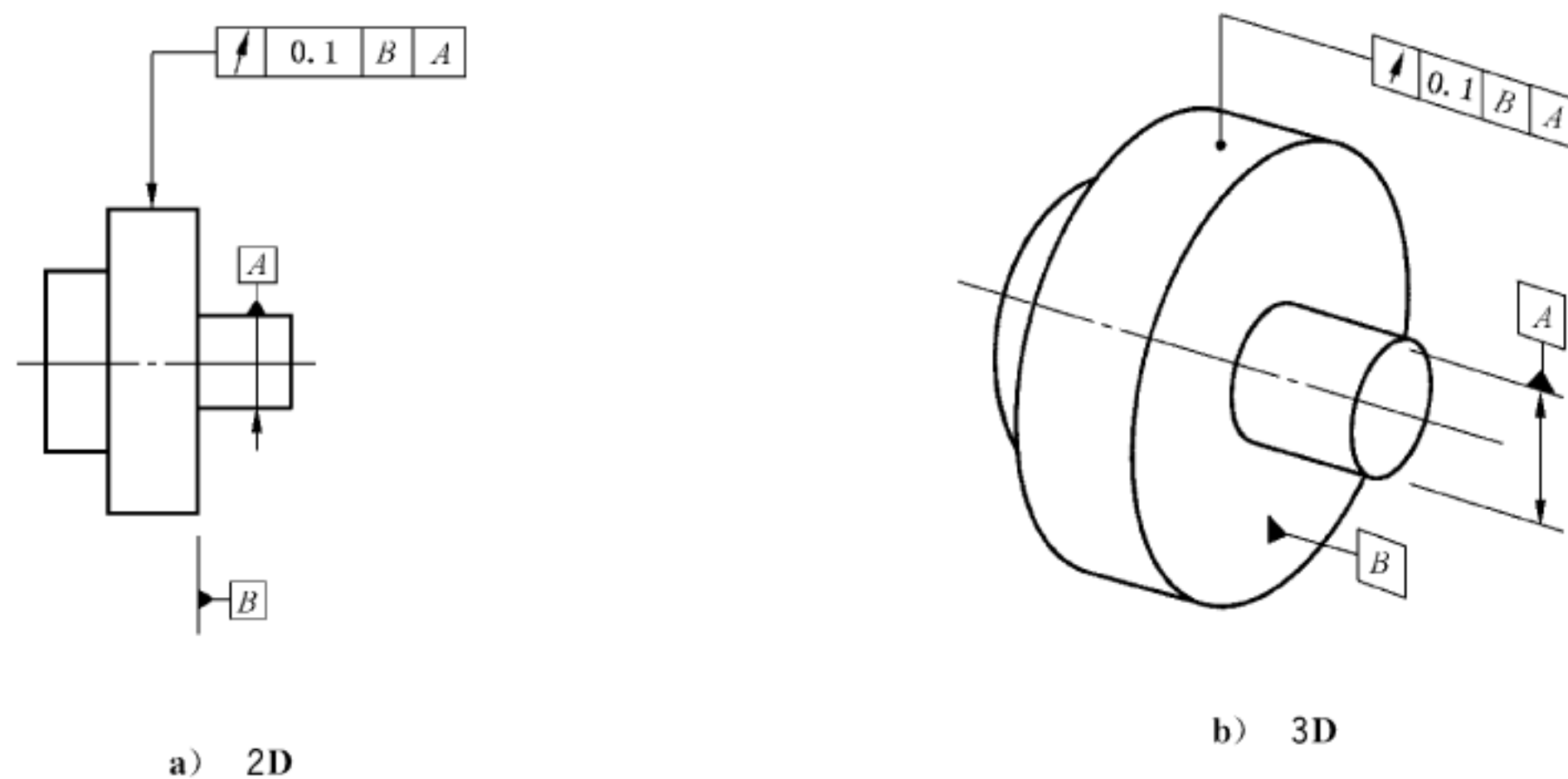
图 173 圆跳动标注
