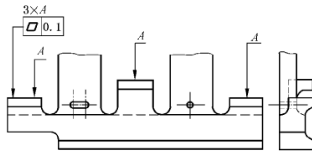
图 18 适用于多个单独要素的规范
