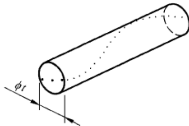
图 95 直线度公差带的定义
