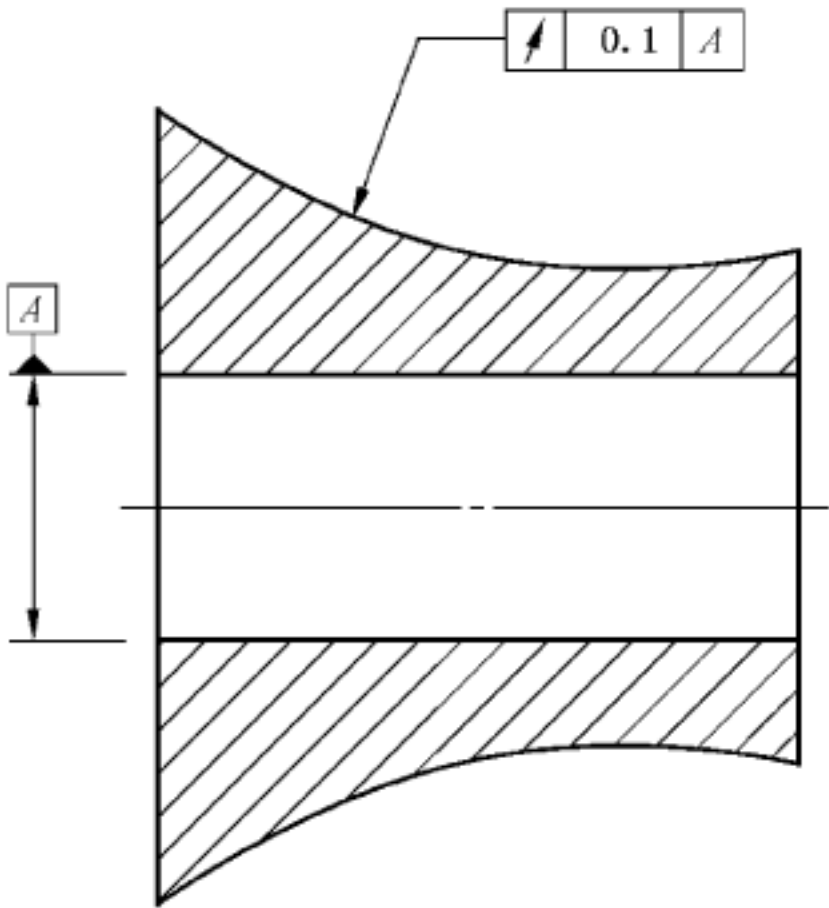
图8 图样标注
