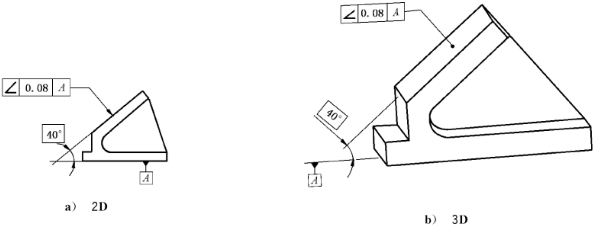
图 148 倾斜度标注
