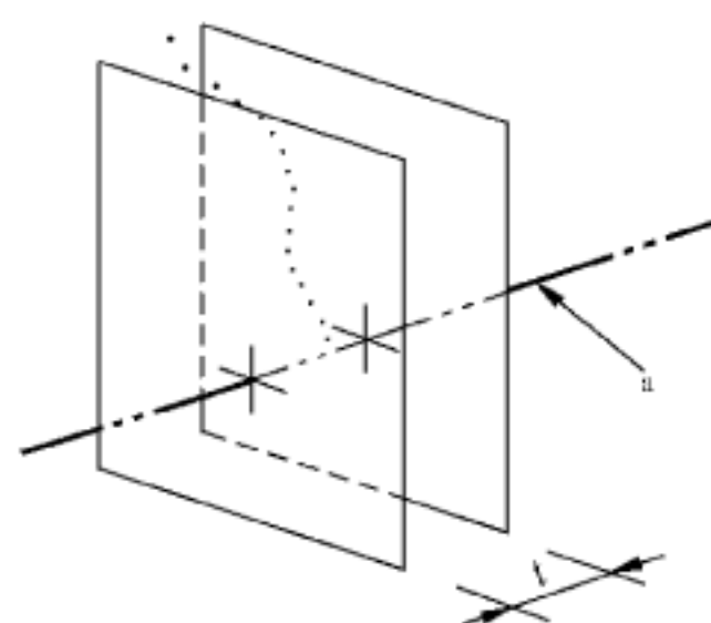
图 129 垂直度公差带的定义
