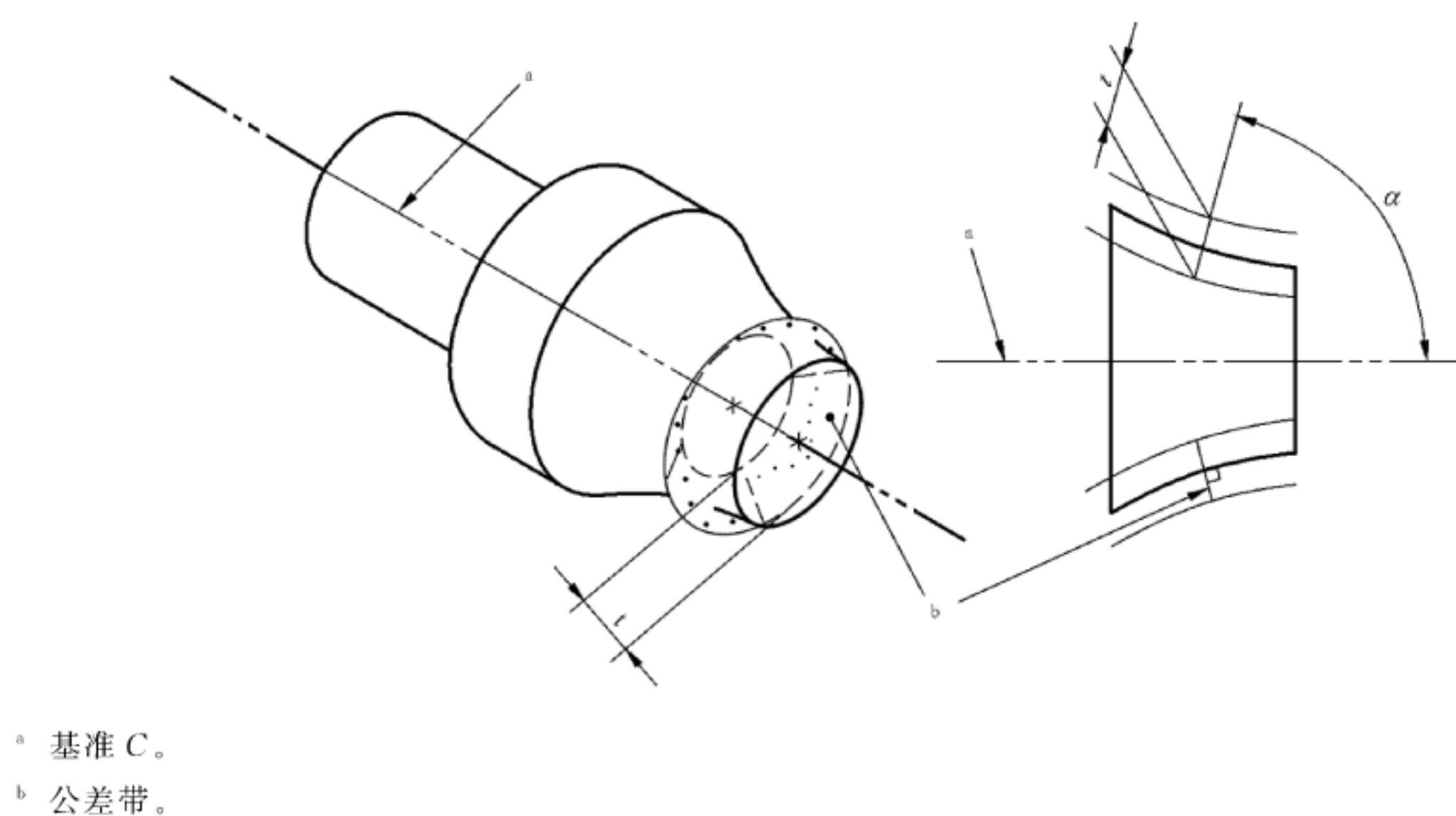
图 183 圆跳动公差带的定义
