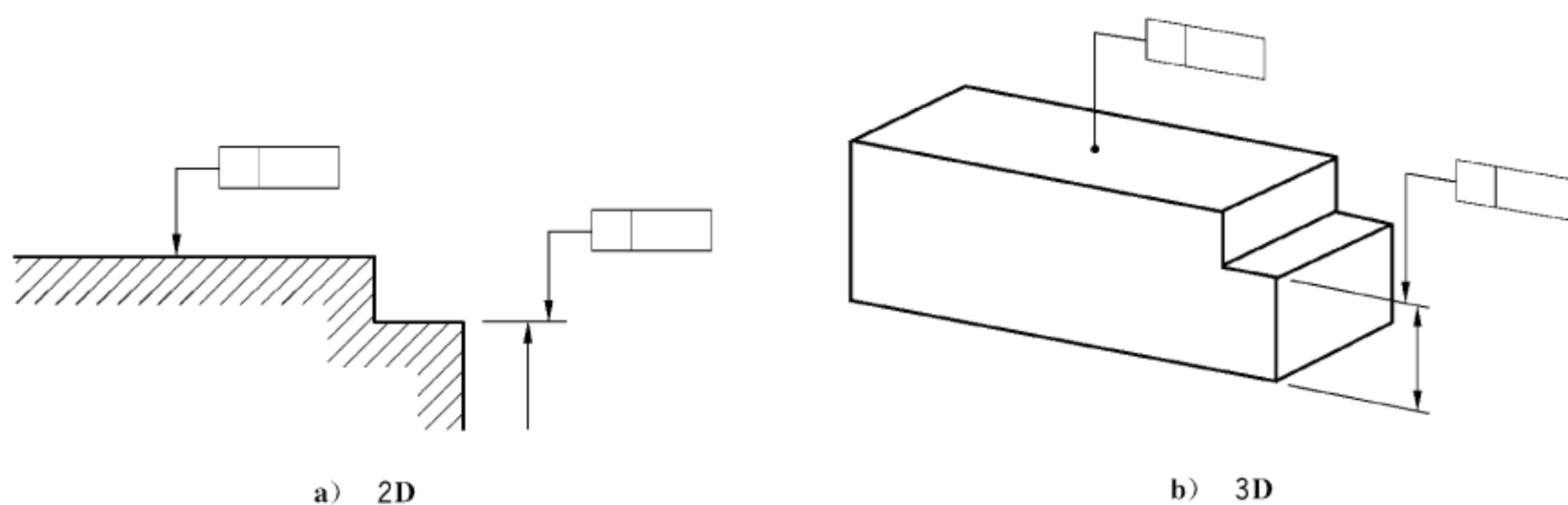
图1 组成要素的标注
