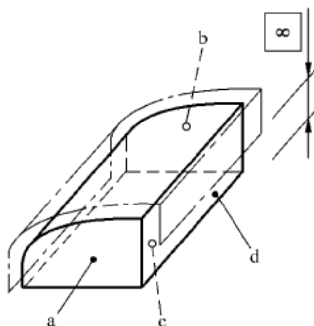
图 61 说明:长点划线勾勒出被测要素的轮廓——面要素 a、b、c 与 d 的下部不在规范的范围
