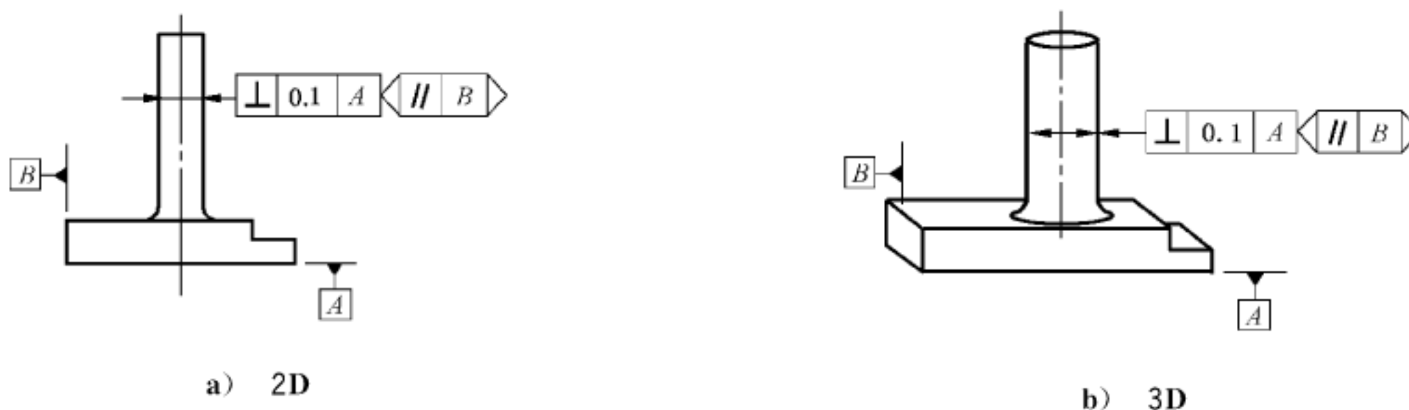
图 130 垂直度标注
