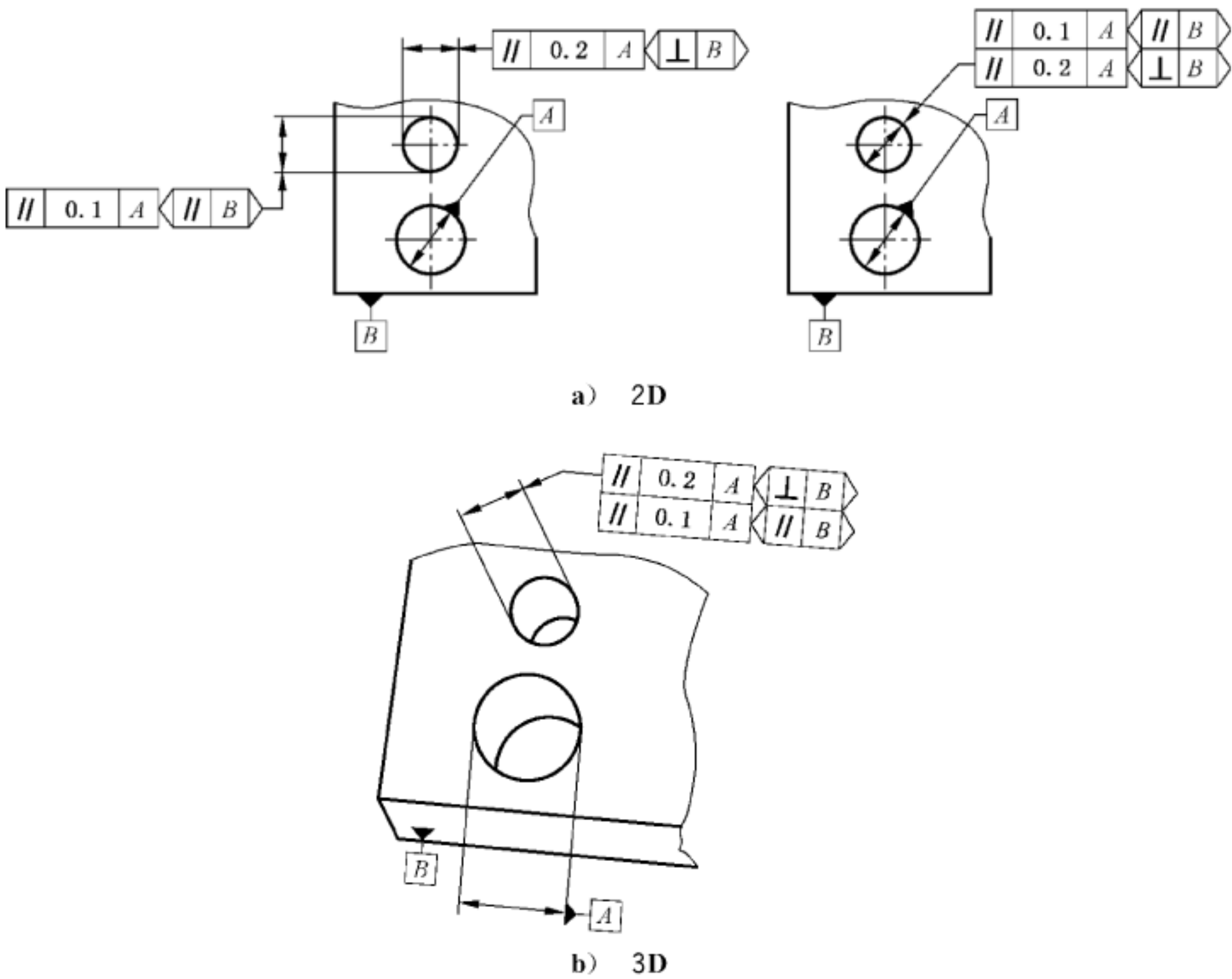
图 116 平行度标注
