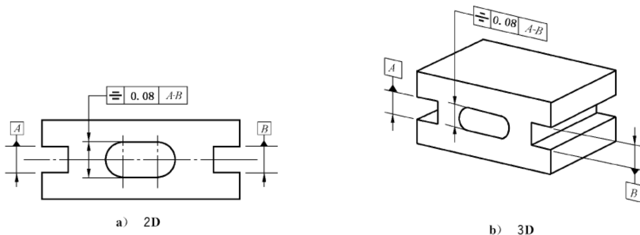
图 170 对称度标注
