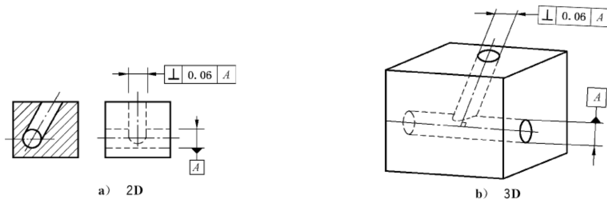
图 128 垂直度标注
