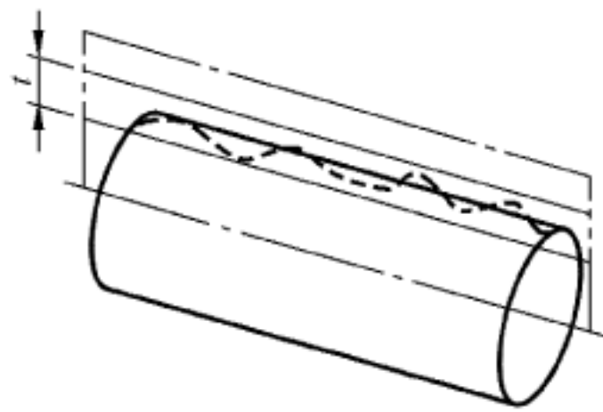
图 93 直线度公差带的定义
