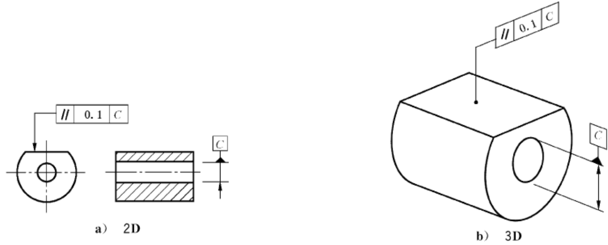
图 124 平行度标注
