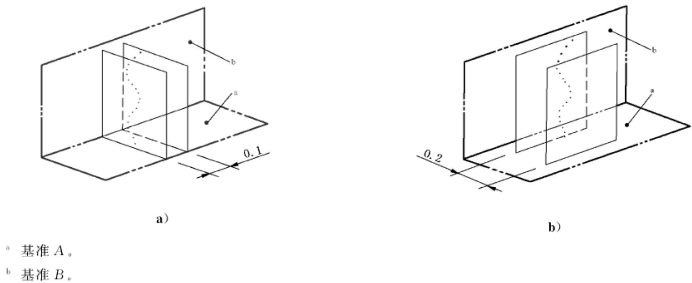
图 133 垂直度公差带的定义
