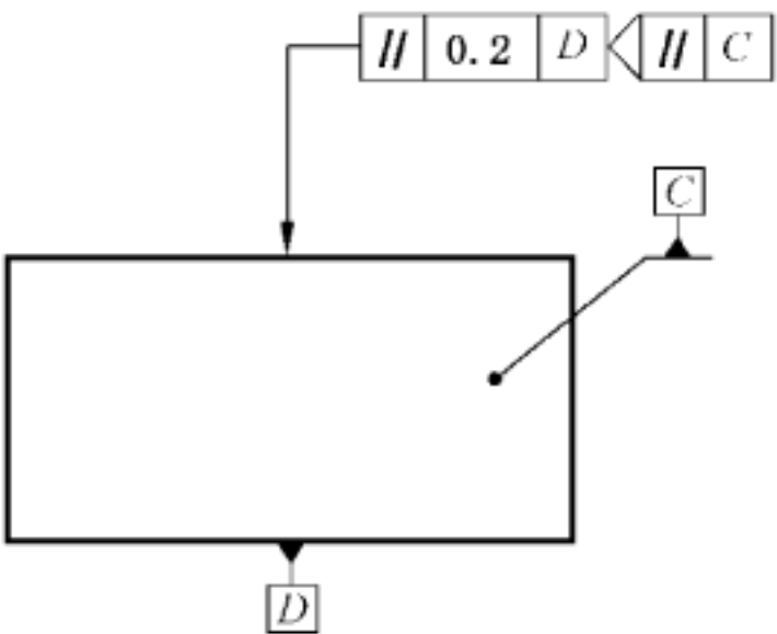
图 77 使用相交平面框格的规范
