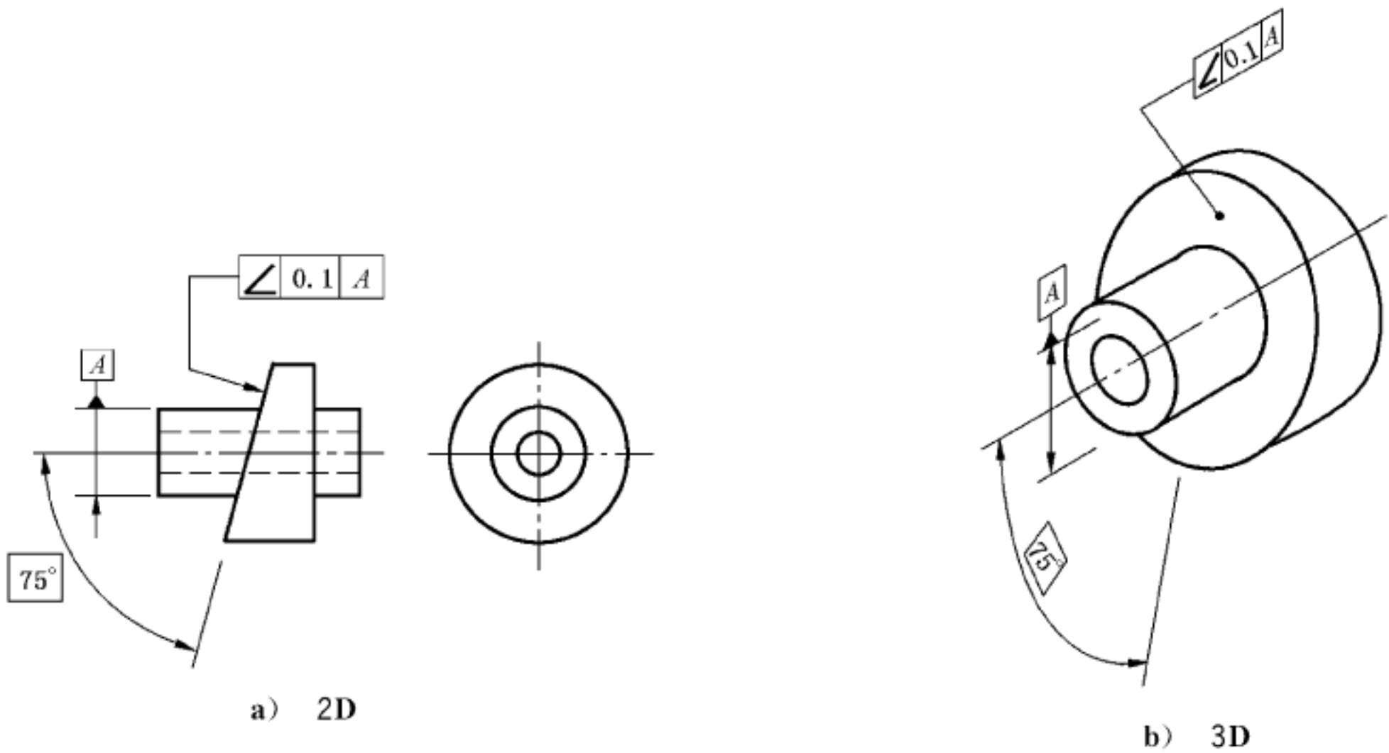
图 146 倾斜度标注
