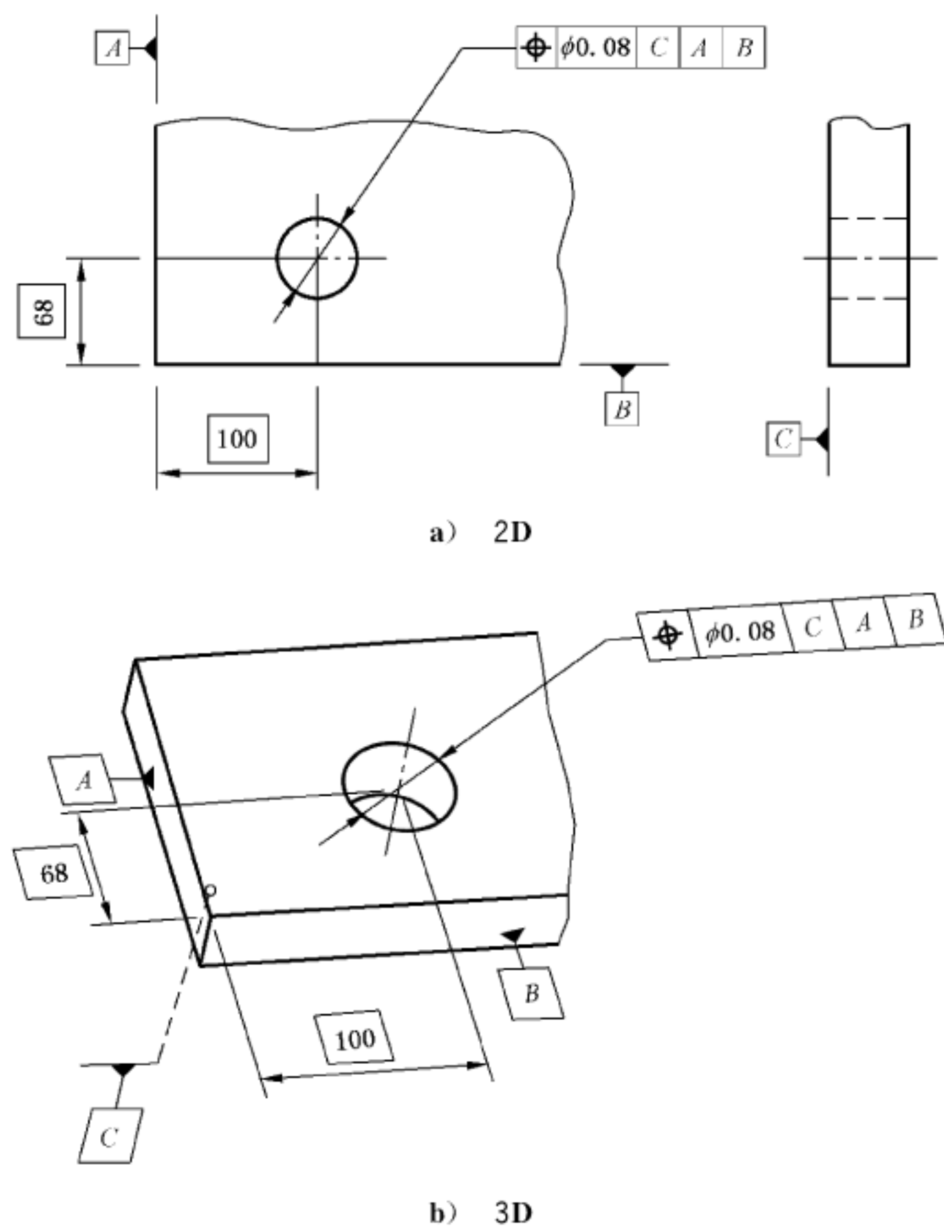
图 154 位置度标注
