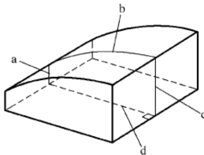
图 51 全周图样标注
