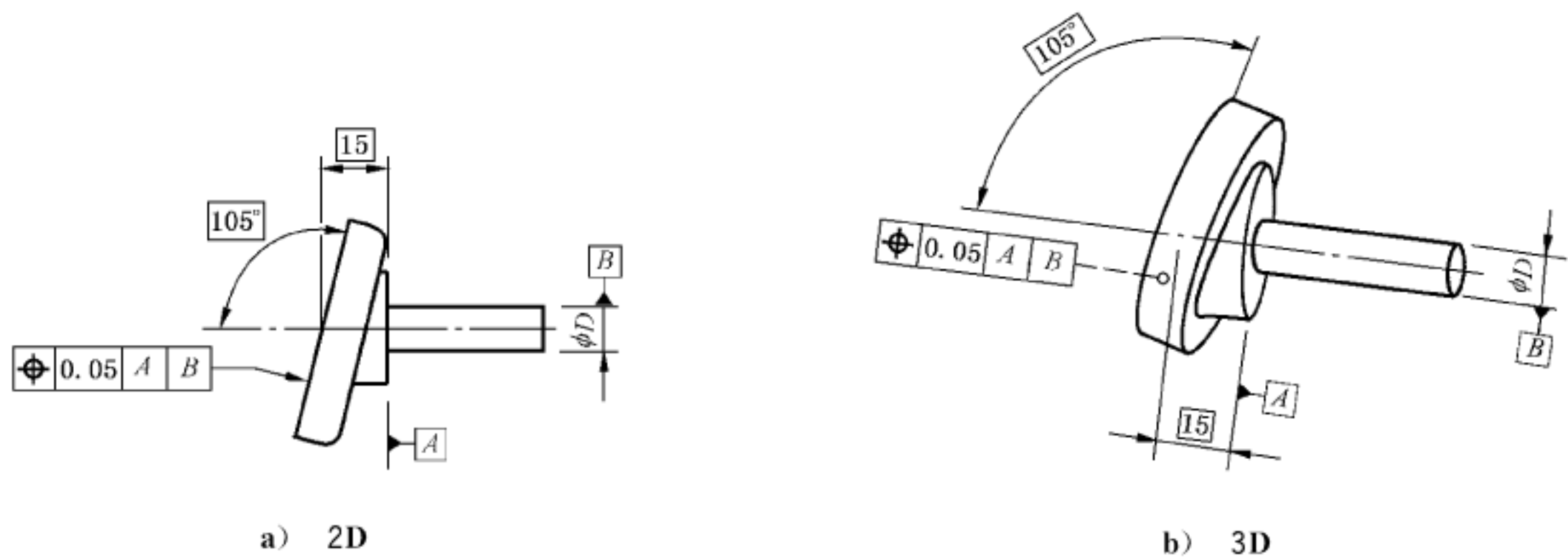
图 161 位置度标注
