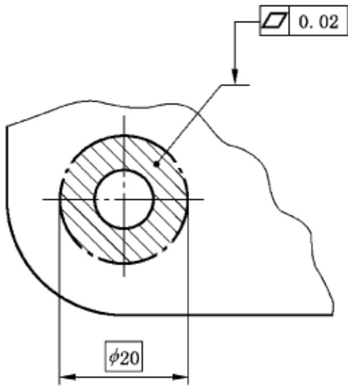
图 59 局部区域标注
