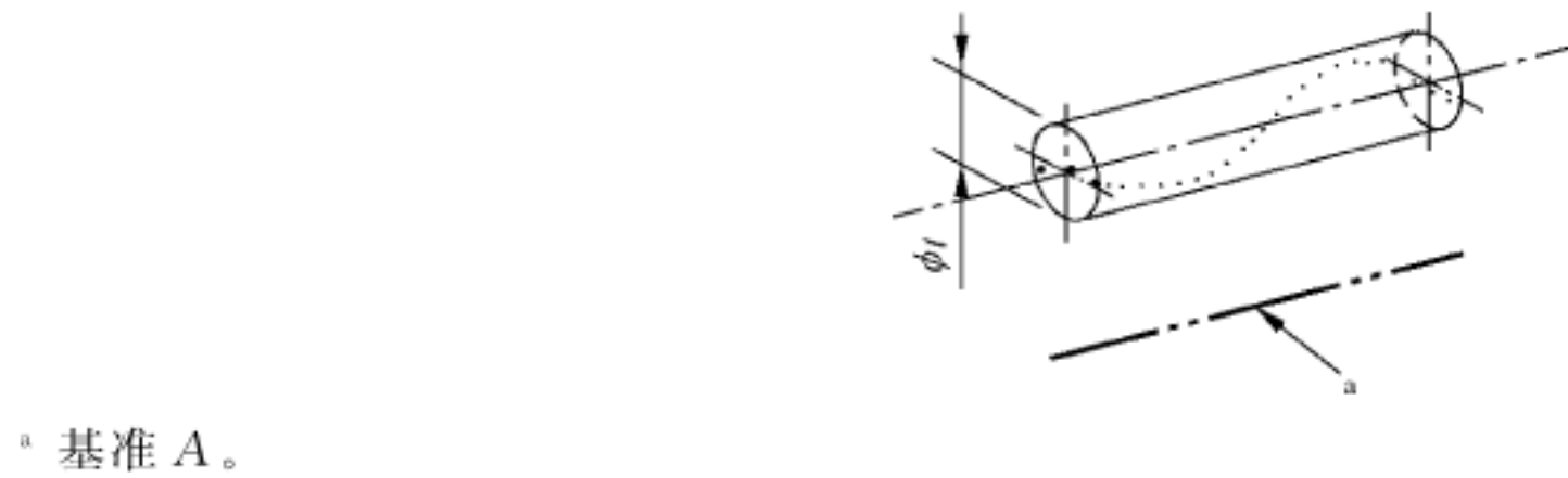
图 119 平行度公差带的定义
