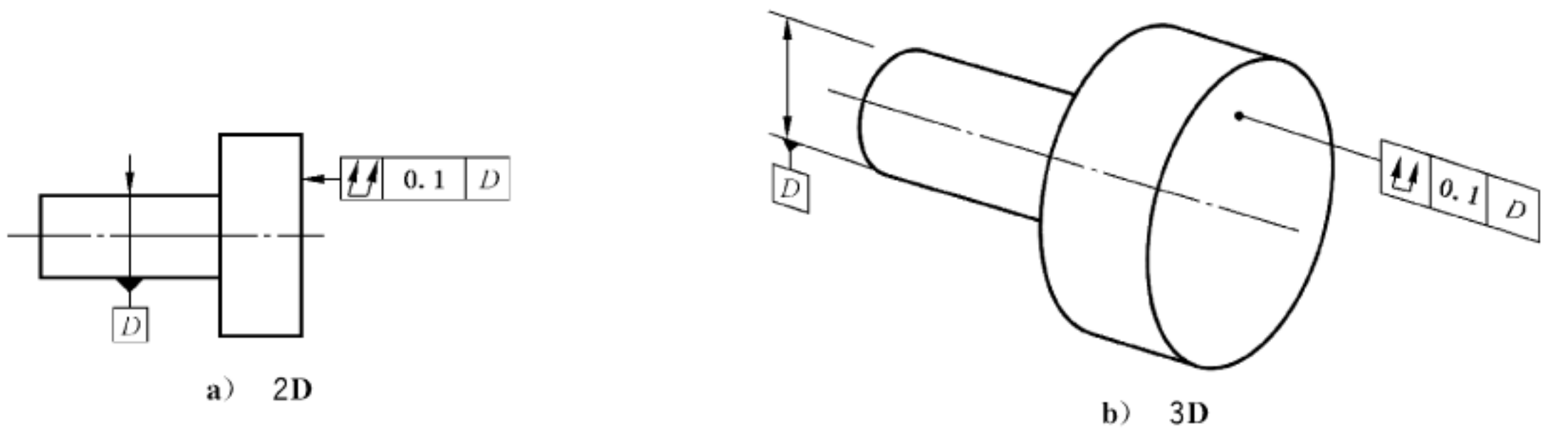
图 186 全跳动标注
