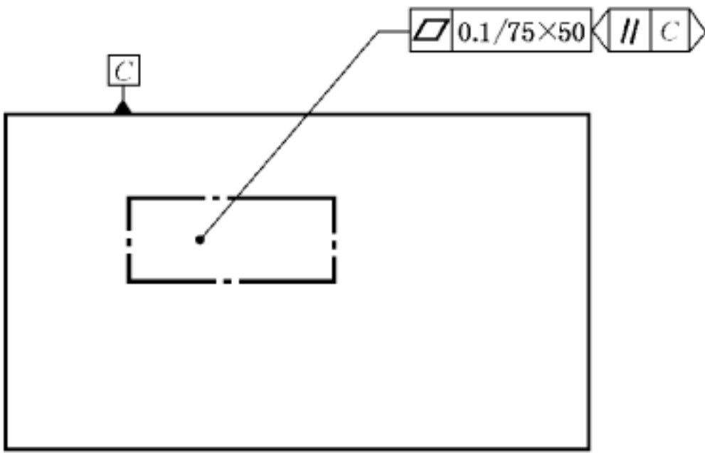
图 67 区域局部规范的标注
