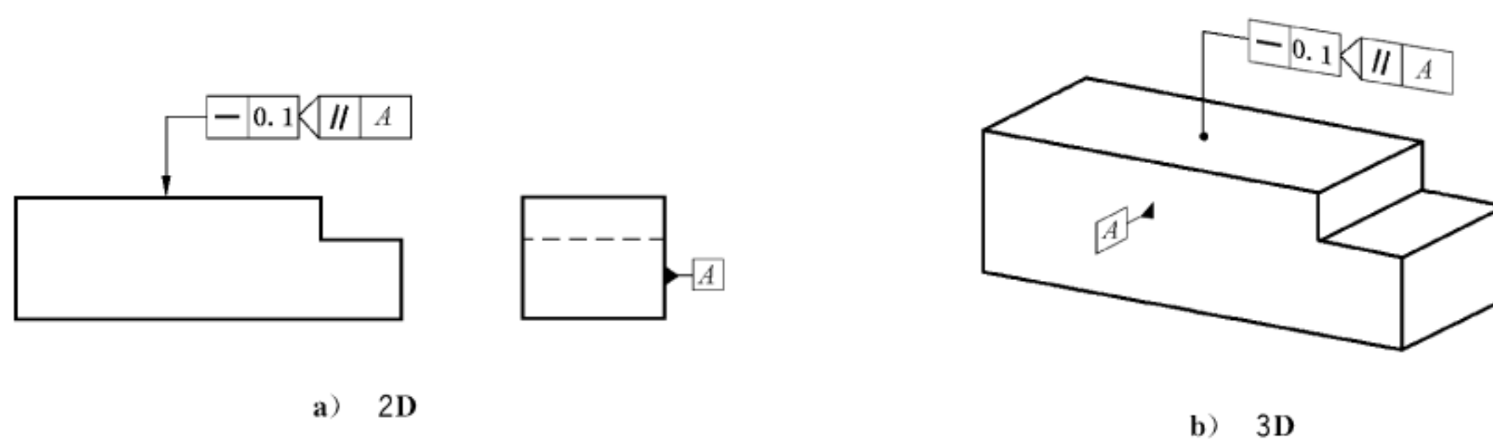
图 90 直线度标注
