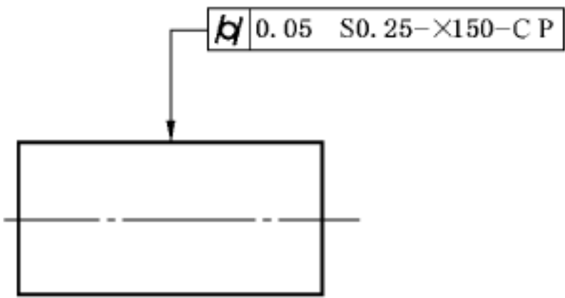
图 45 滤波规范,参照要素与特征规范元素
