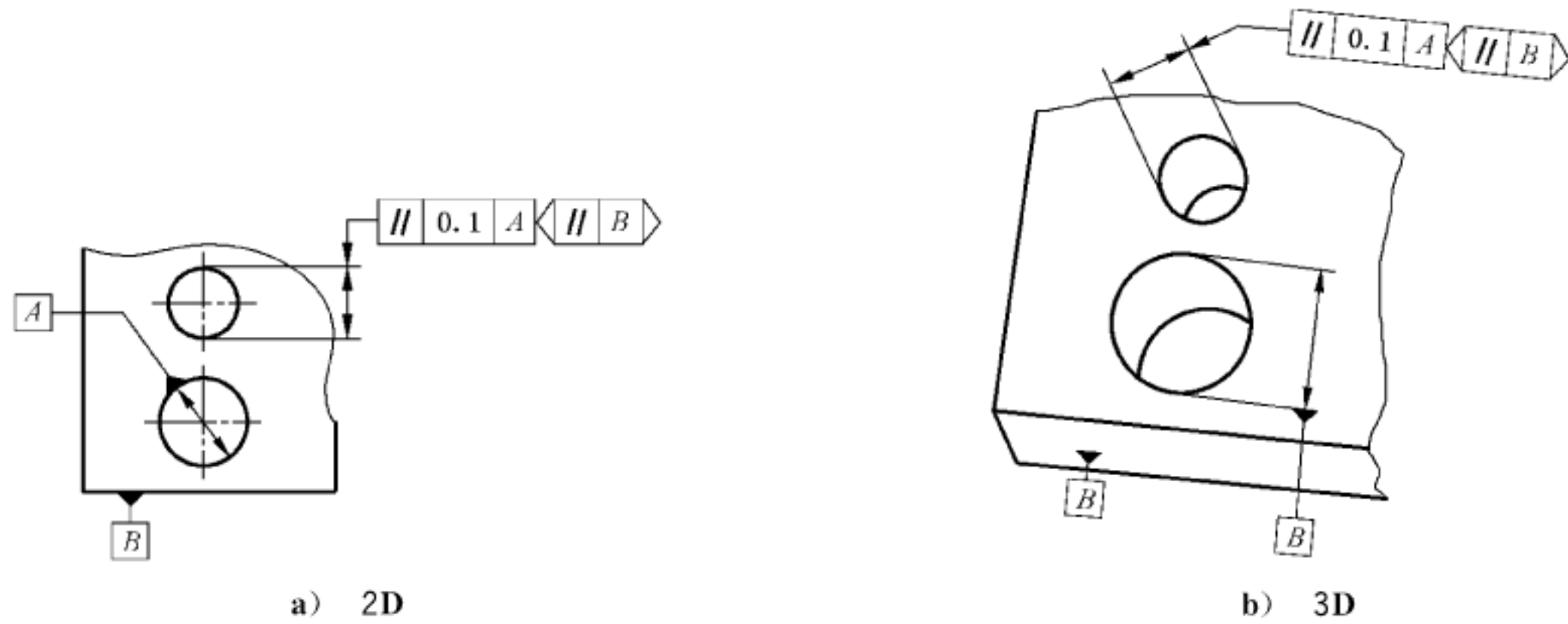
图 112 平行度标注
