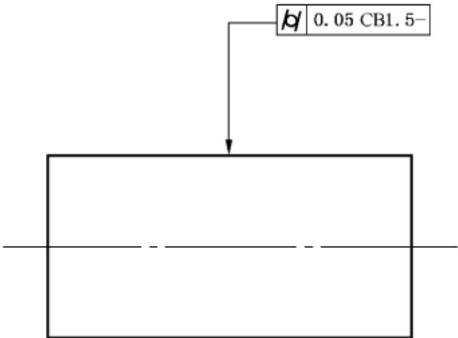
图 E.14 圆度公差示例——封闭球滤波器
