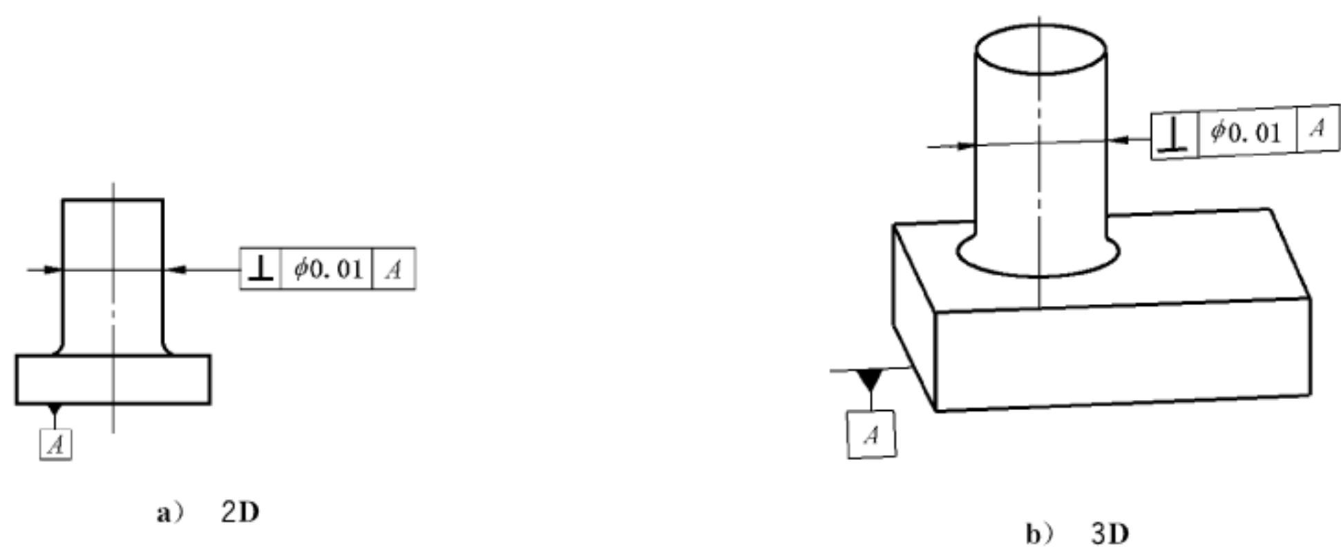
图 134 垂直度标注
