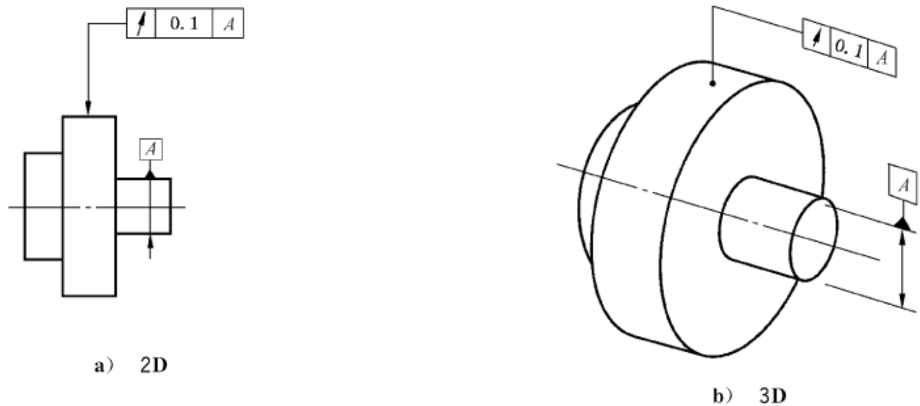
图 172 圆跳动标注
