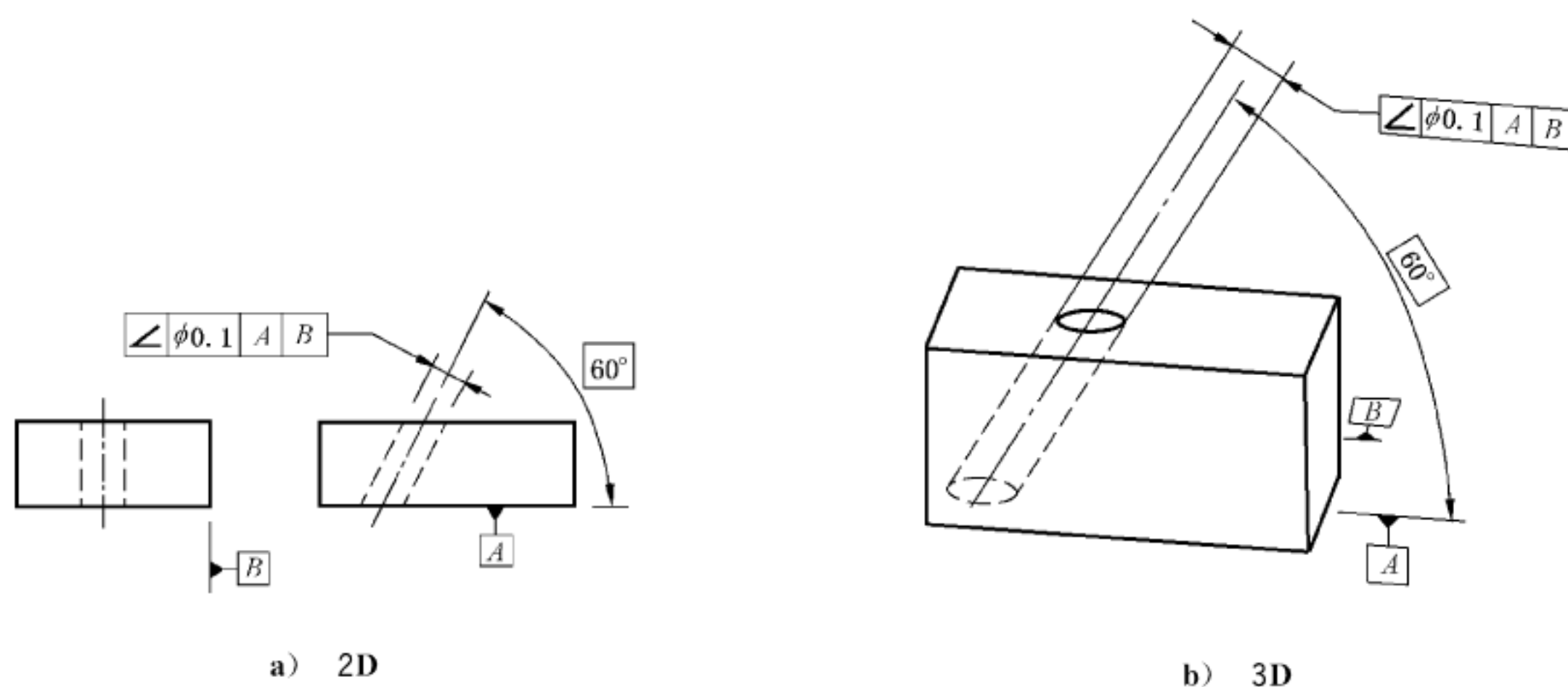
图 144 倾斜度标注
