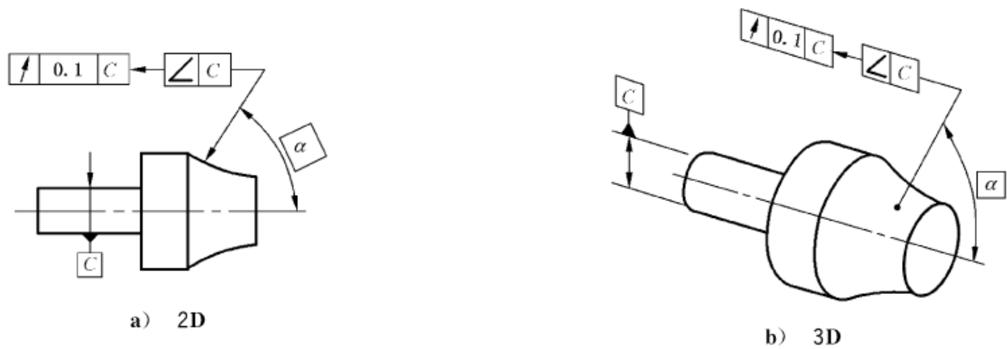
图 182 圆跳动标注
