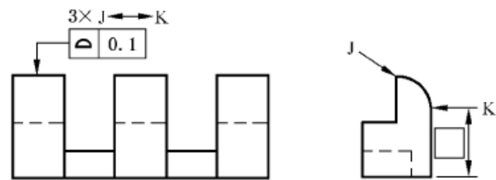
图 63 多个组合被测要素的标注
