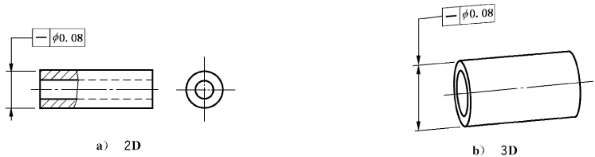
图 94 直线度标注
