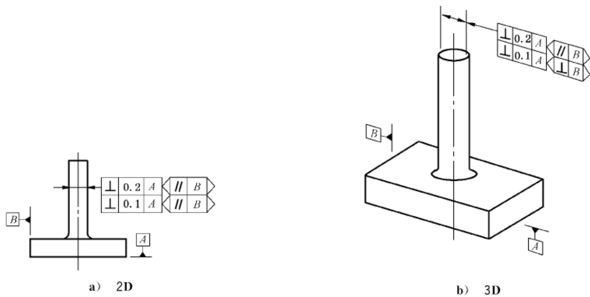
图 132 垂直度标注
