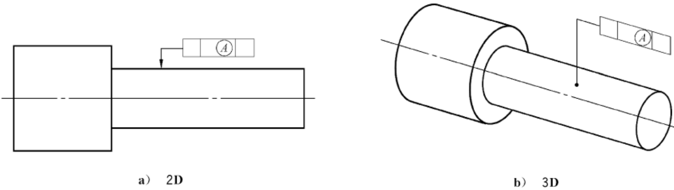
图7 中心要素的标注
