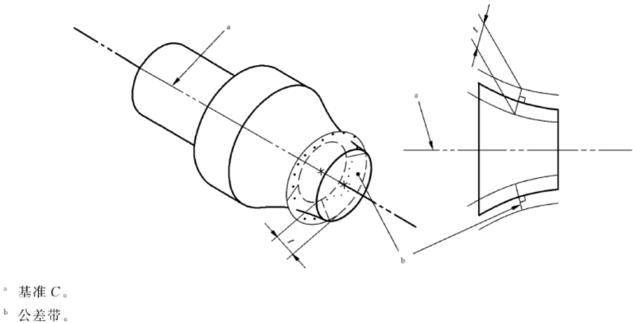
图 181 圆跳动公差带的定义
