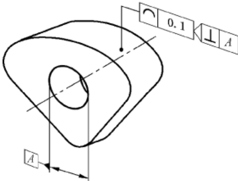
图 79 使用垂直于基准的相交平面规范
