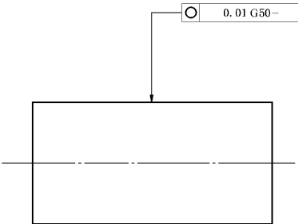
图 E.13 圆度公差示例——高斯滤波器
