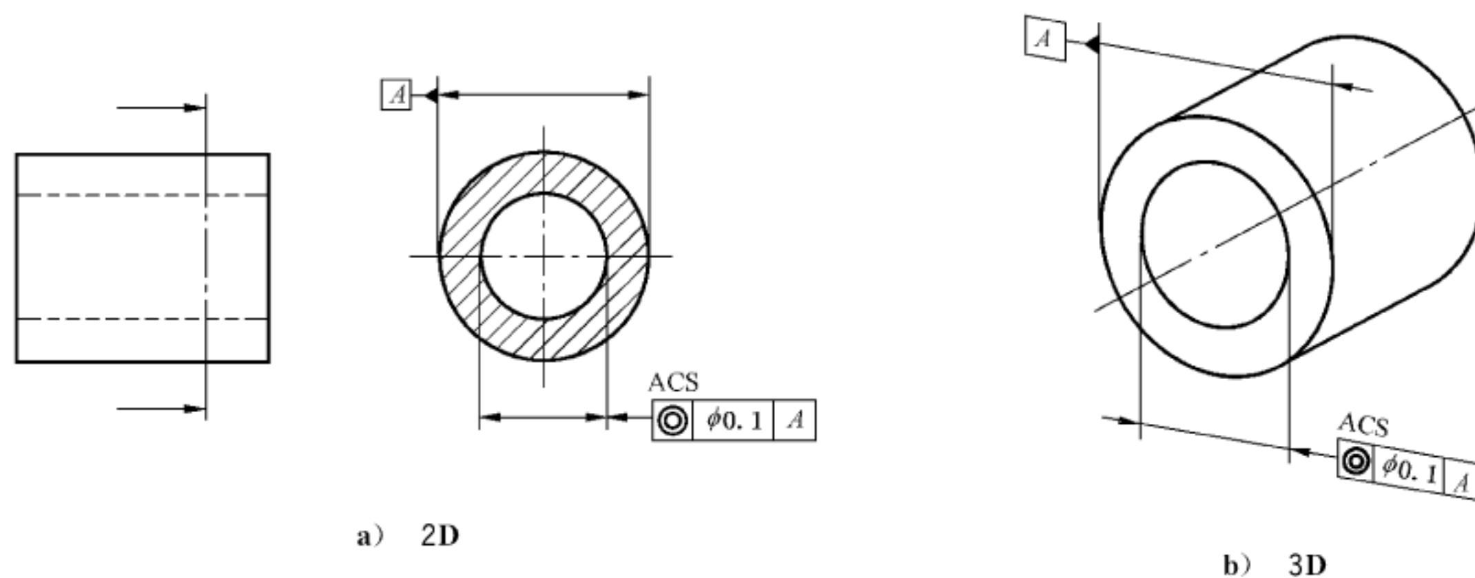
图 163 同心度标注
