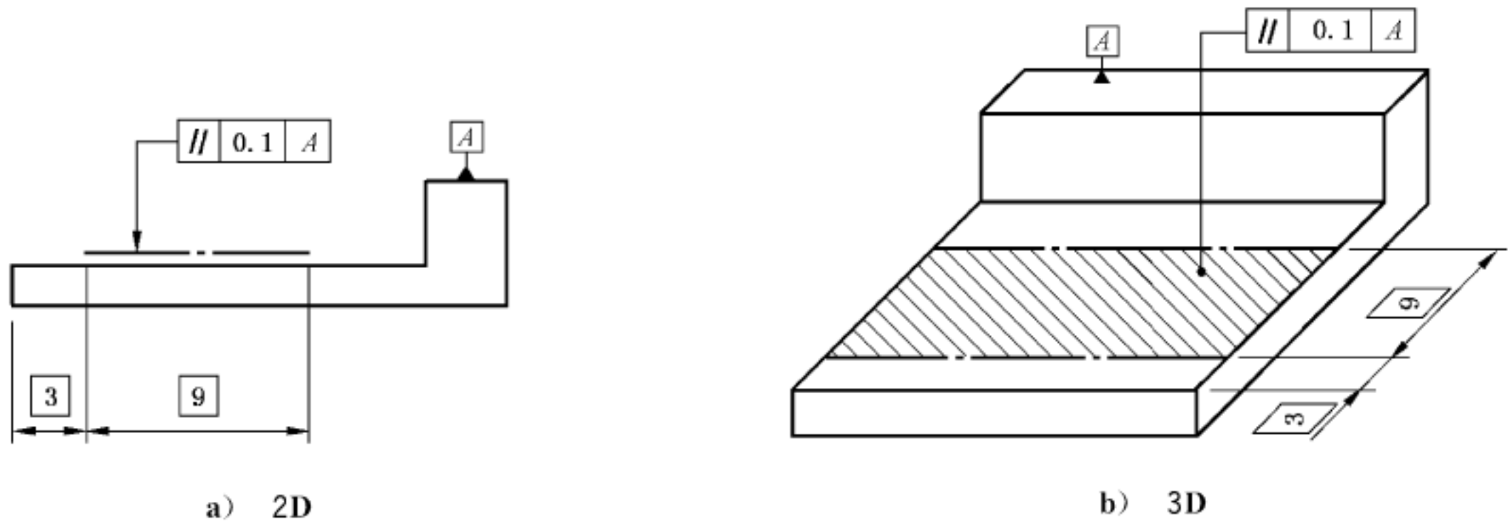
图 58 局部区域标注
