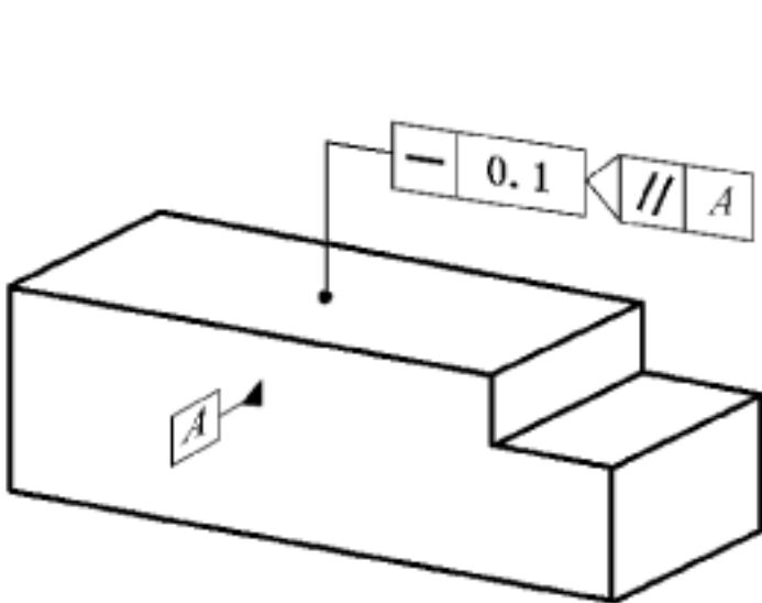
图 78 使用平行于基准的相交平面的规范
