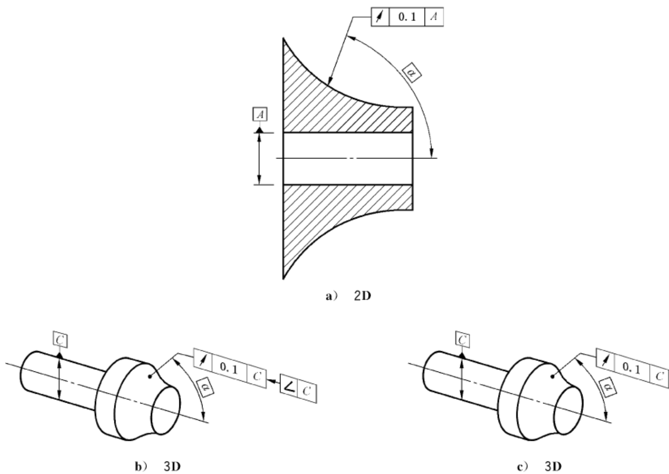
图 85 图样标注
