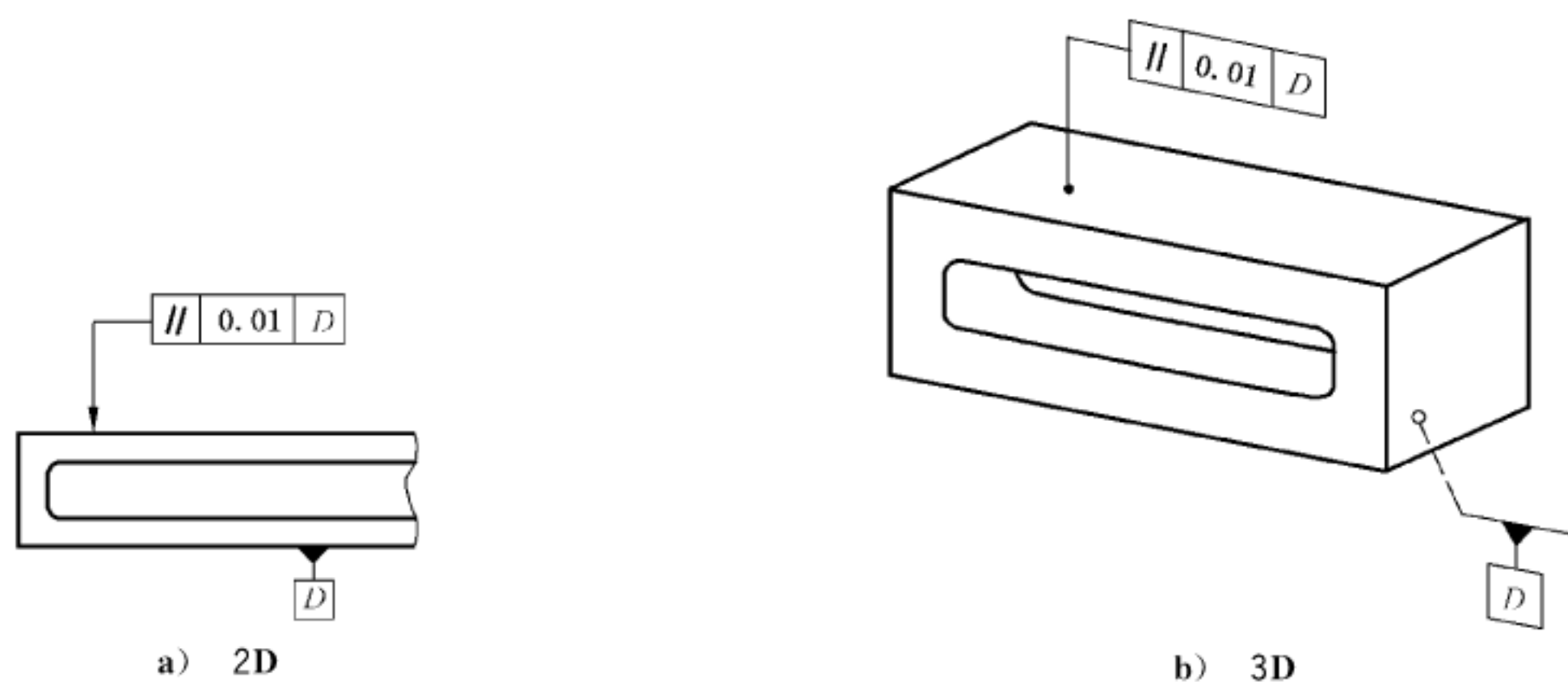
图 126 平行度标注
