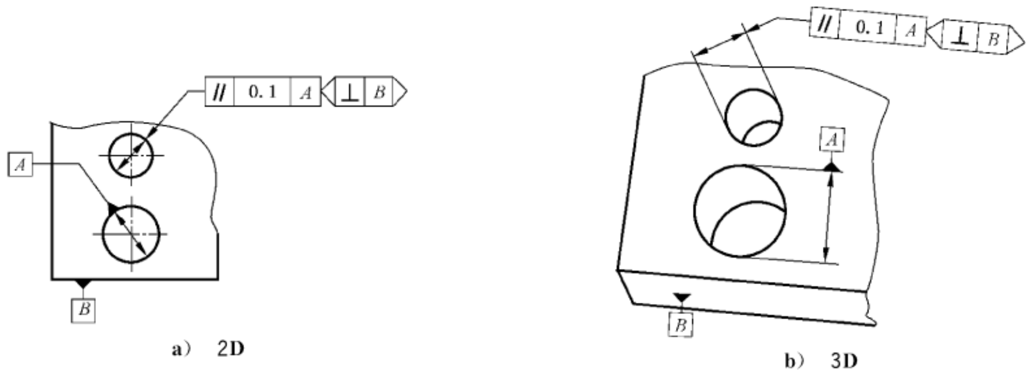
图 114 平行度标注
