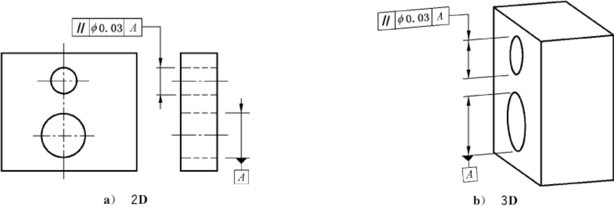
图 118 平行度标注
