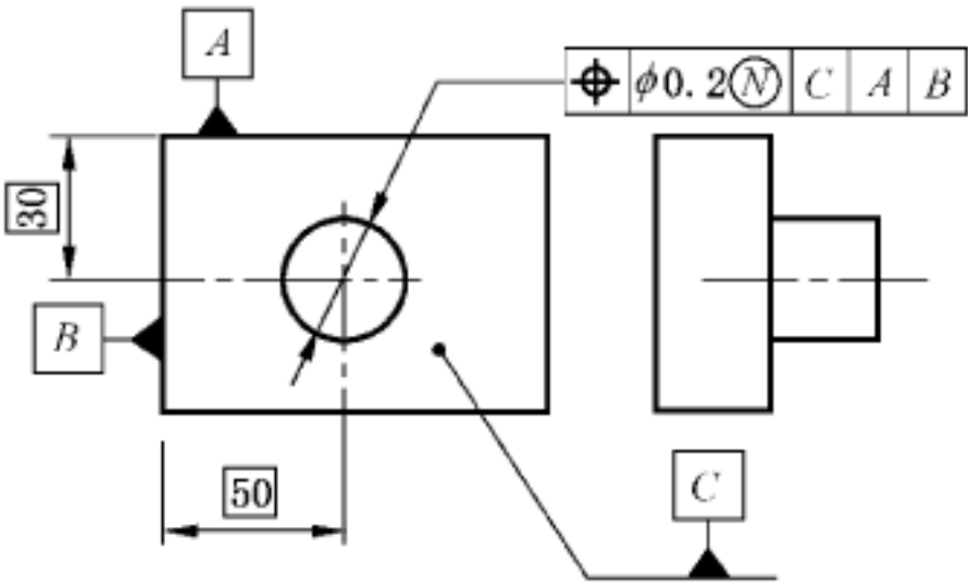
图 29 最小外接拟合被测要素——图样标注
