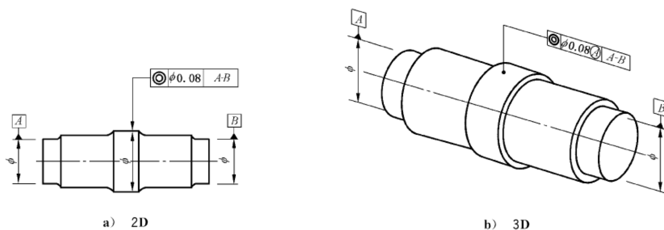
图 165 同轴度标注
