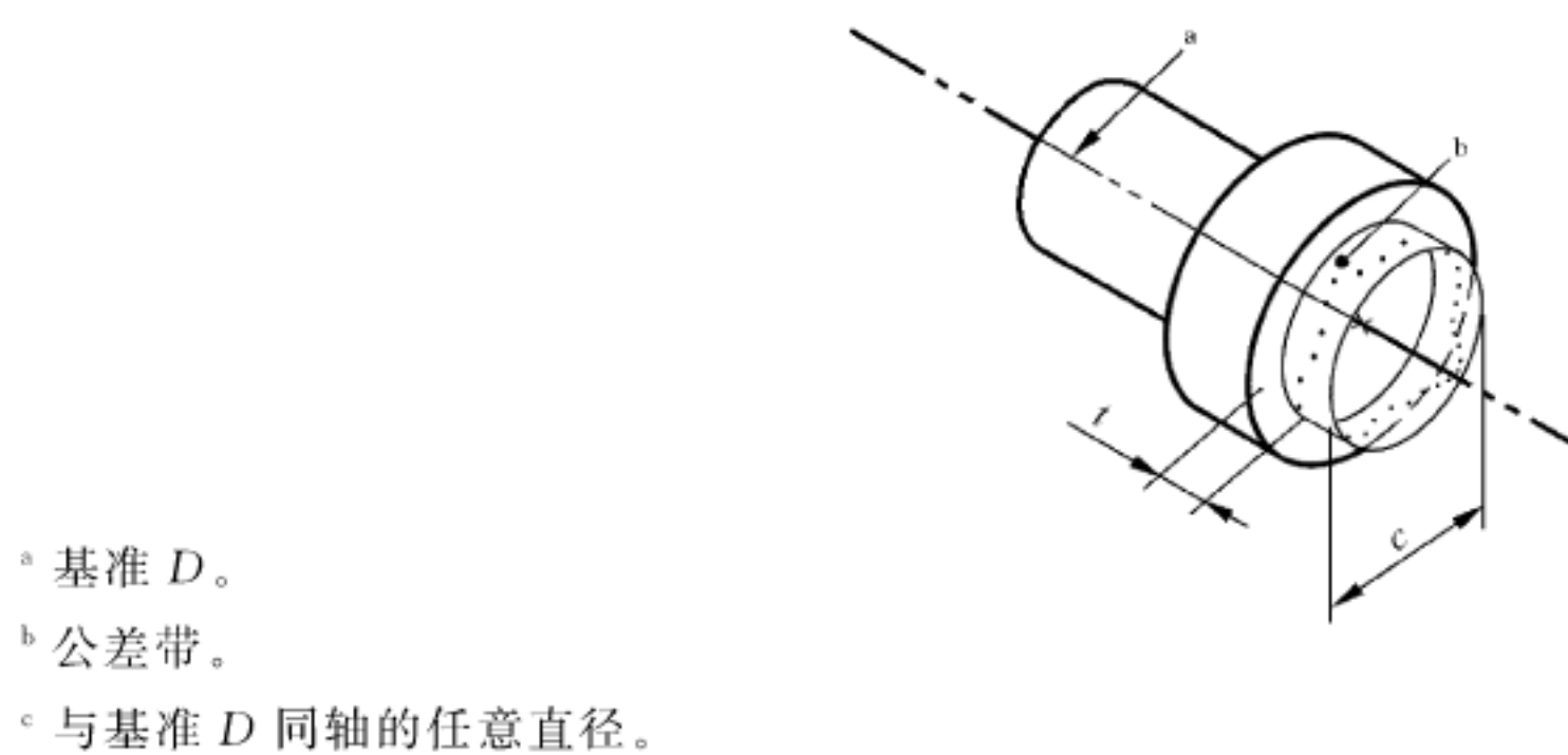
图 178 圆跳动公差带的定义
