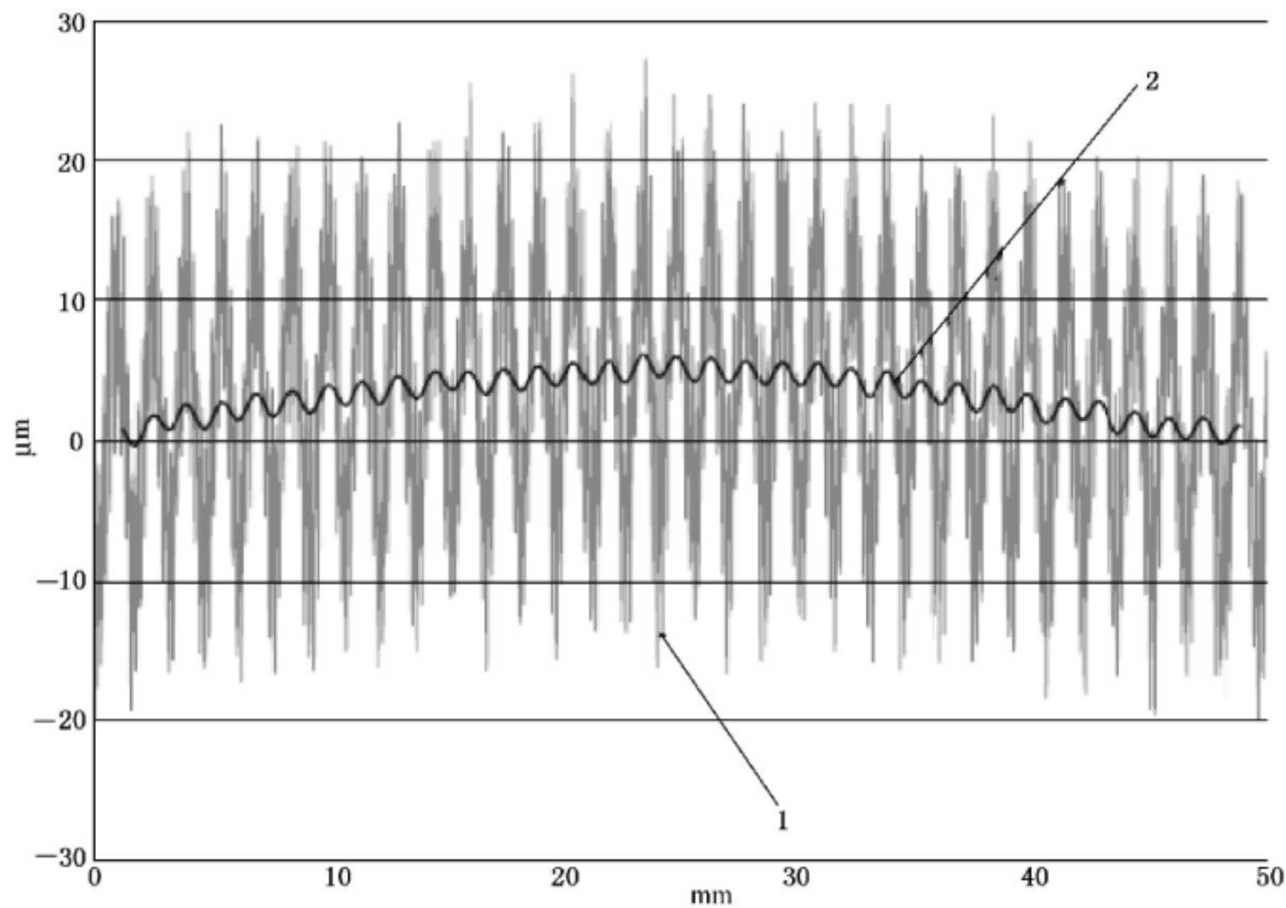
b) 2.5 mm 的长波通高斯滤波器
