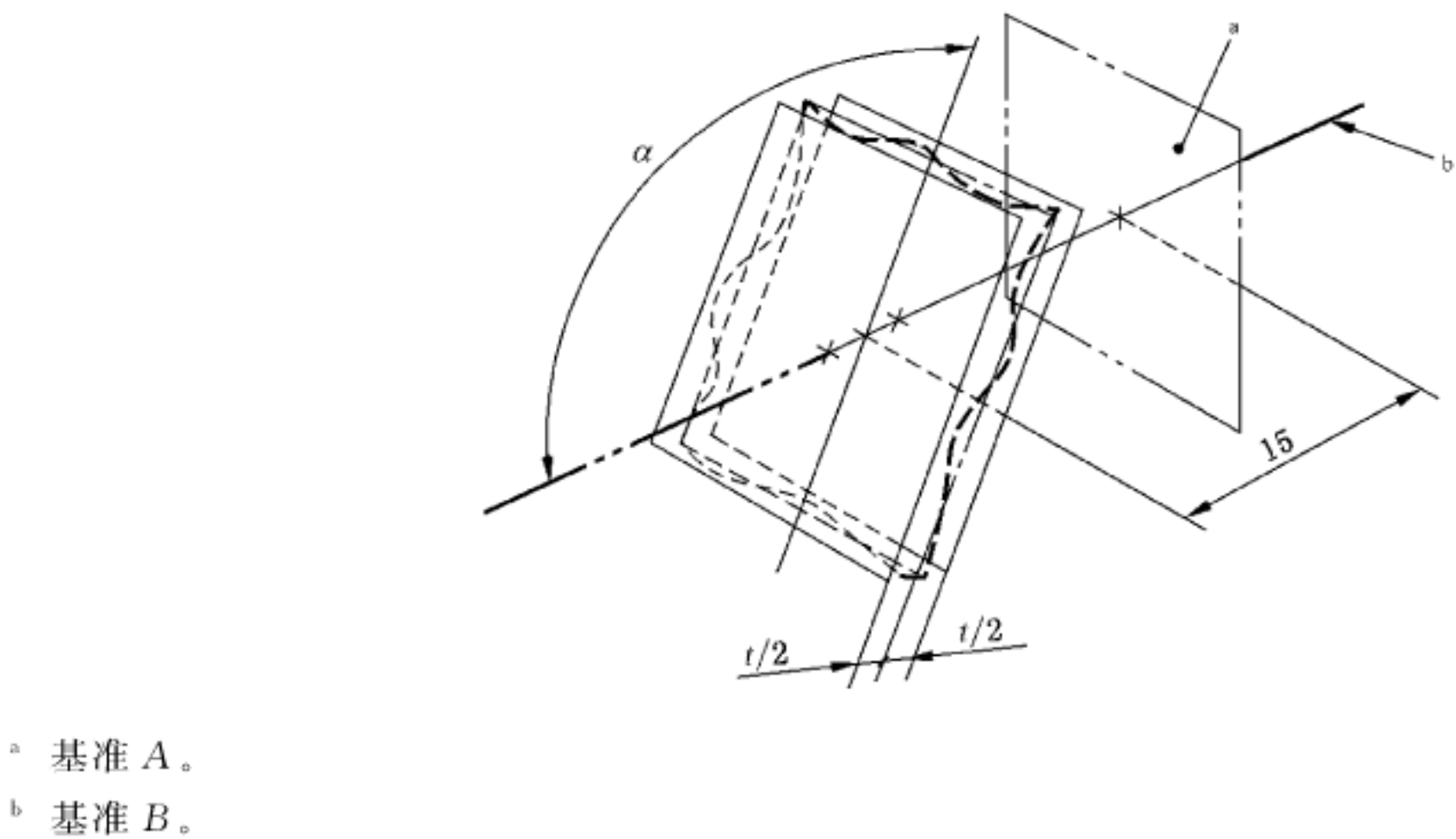
图 162 位置度公差的定义
