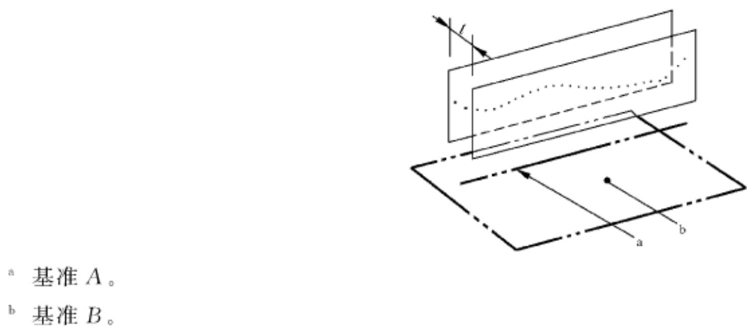
图 115 平行度公差带的定义
