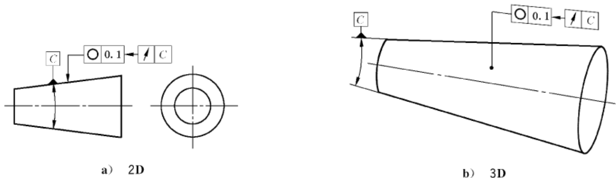
图 100 圆度标注
