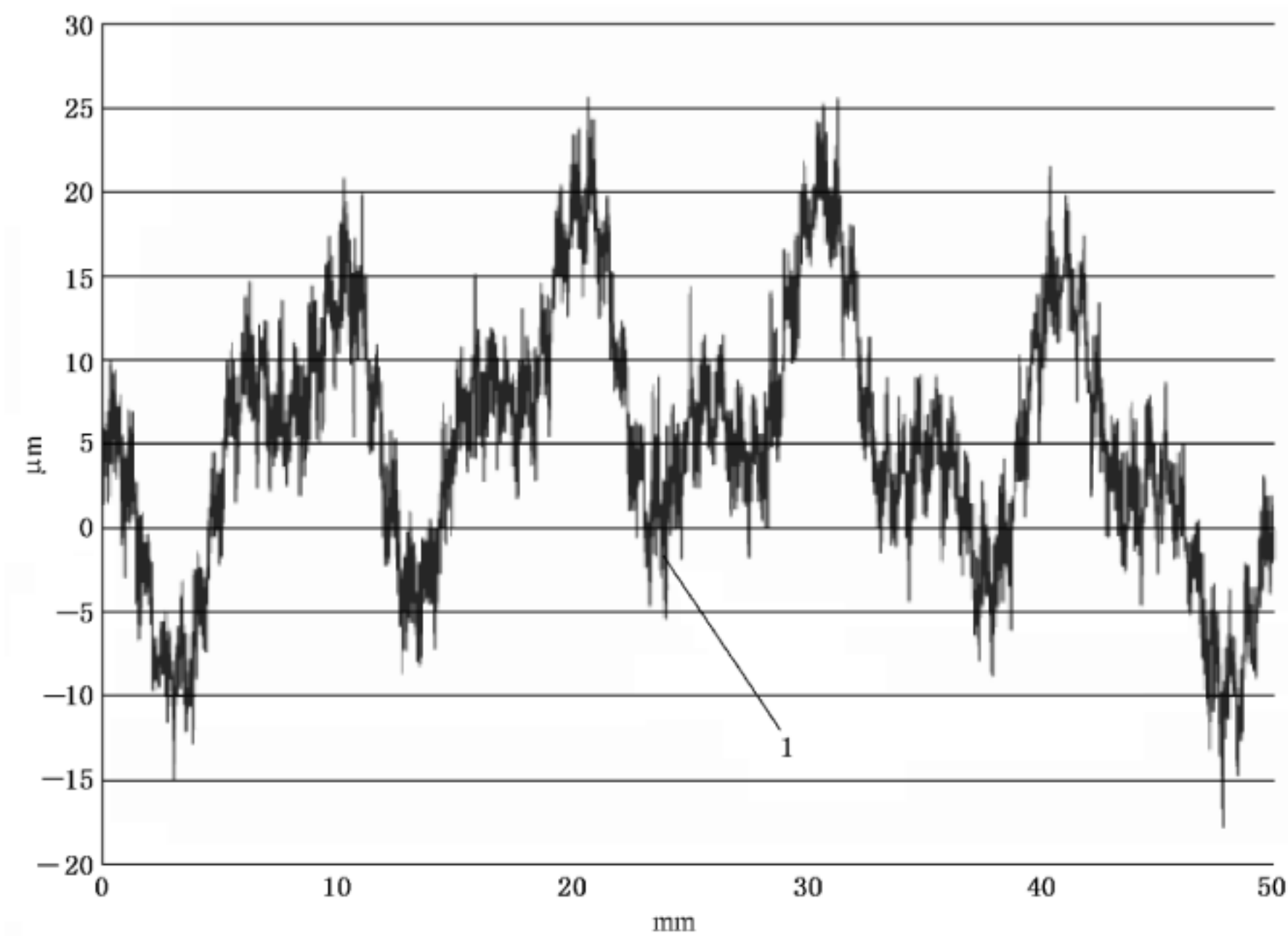
说明： 1——未经滤波的轮廓。
