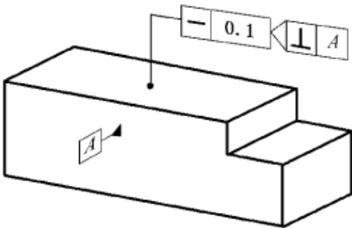
图 80 使用垂直于基准的相交平面规范
