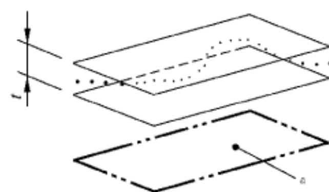
图 121 平行度公差带的定义
