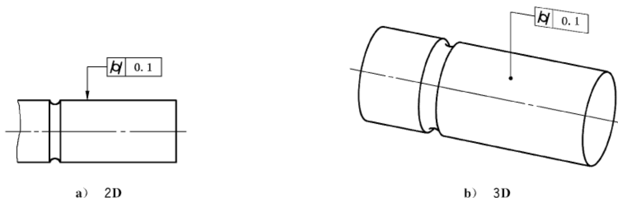
图 102 圆柱度标注
