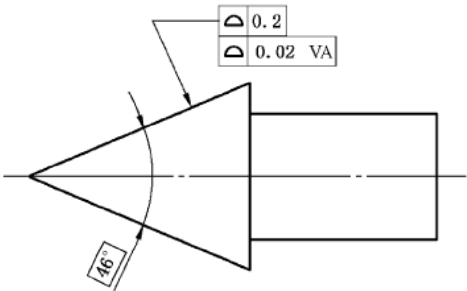
图 24 可变角度,VA,修饰符
