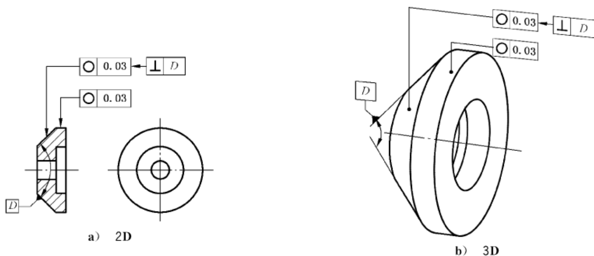
图 98 圆度标注
