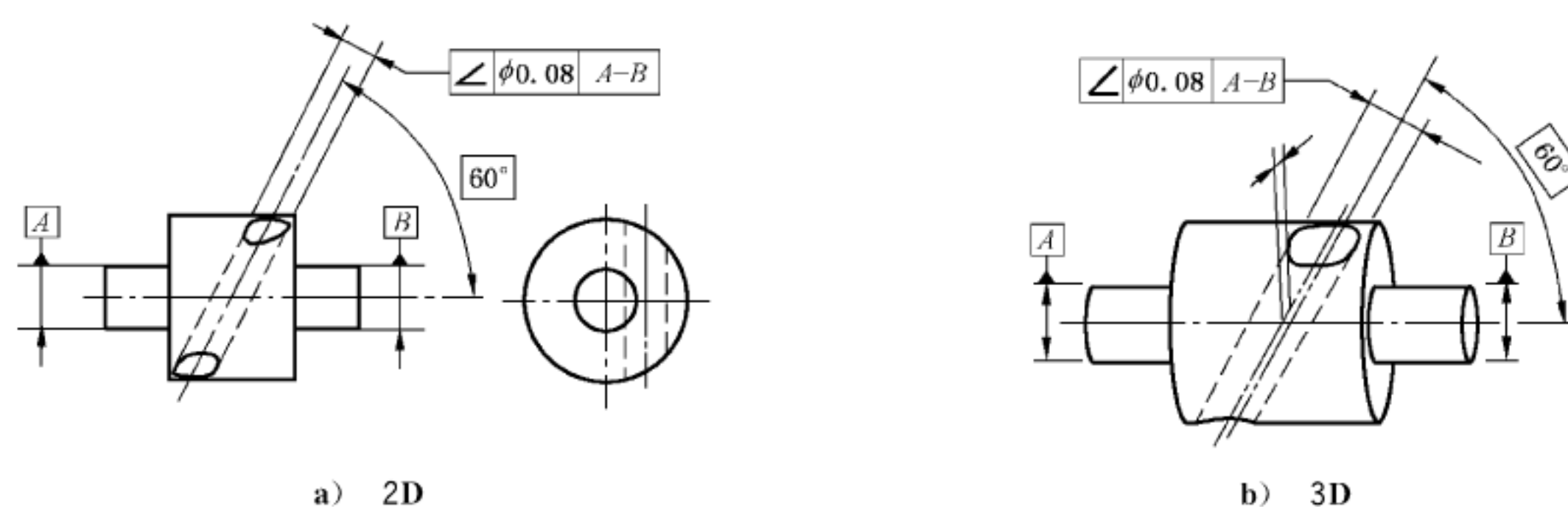
图 142 倾斜度
