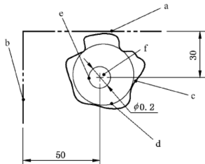
图 33 最大内切拟合被测要素——图样标注
