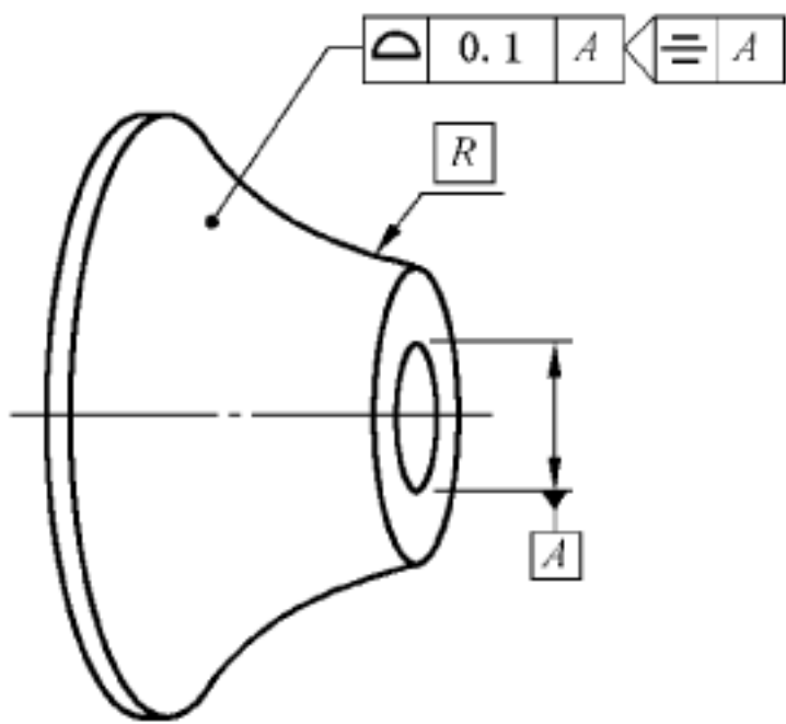
图 81 使用对称于(包含)基准的相交平面规范
