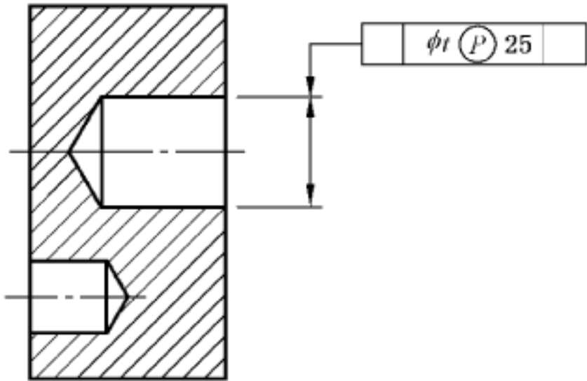
图 70 带延伸公差修饰符的几何公差规范标注,在公差框格中使用延伸被测要素长度来间接标注
