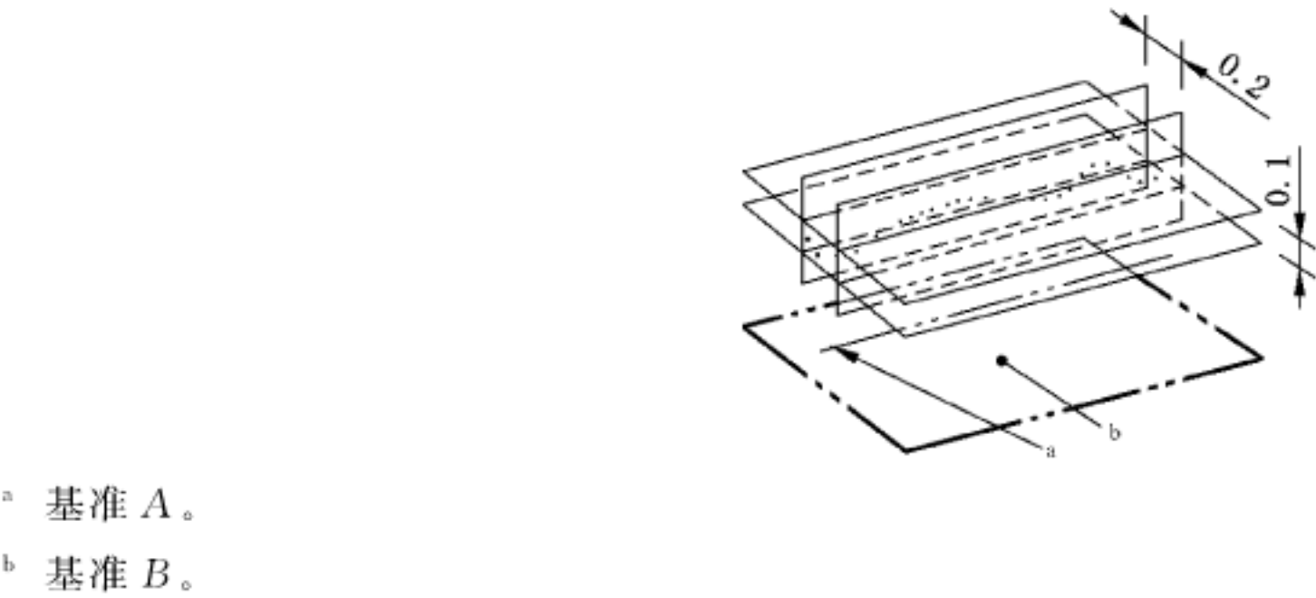
图 117 平行度公差带的定义
