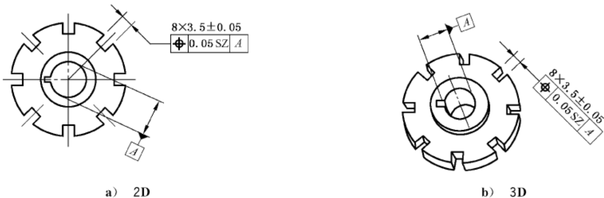
图 159 位置度标注
