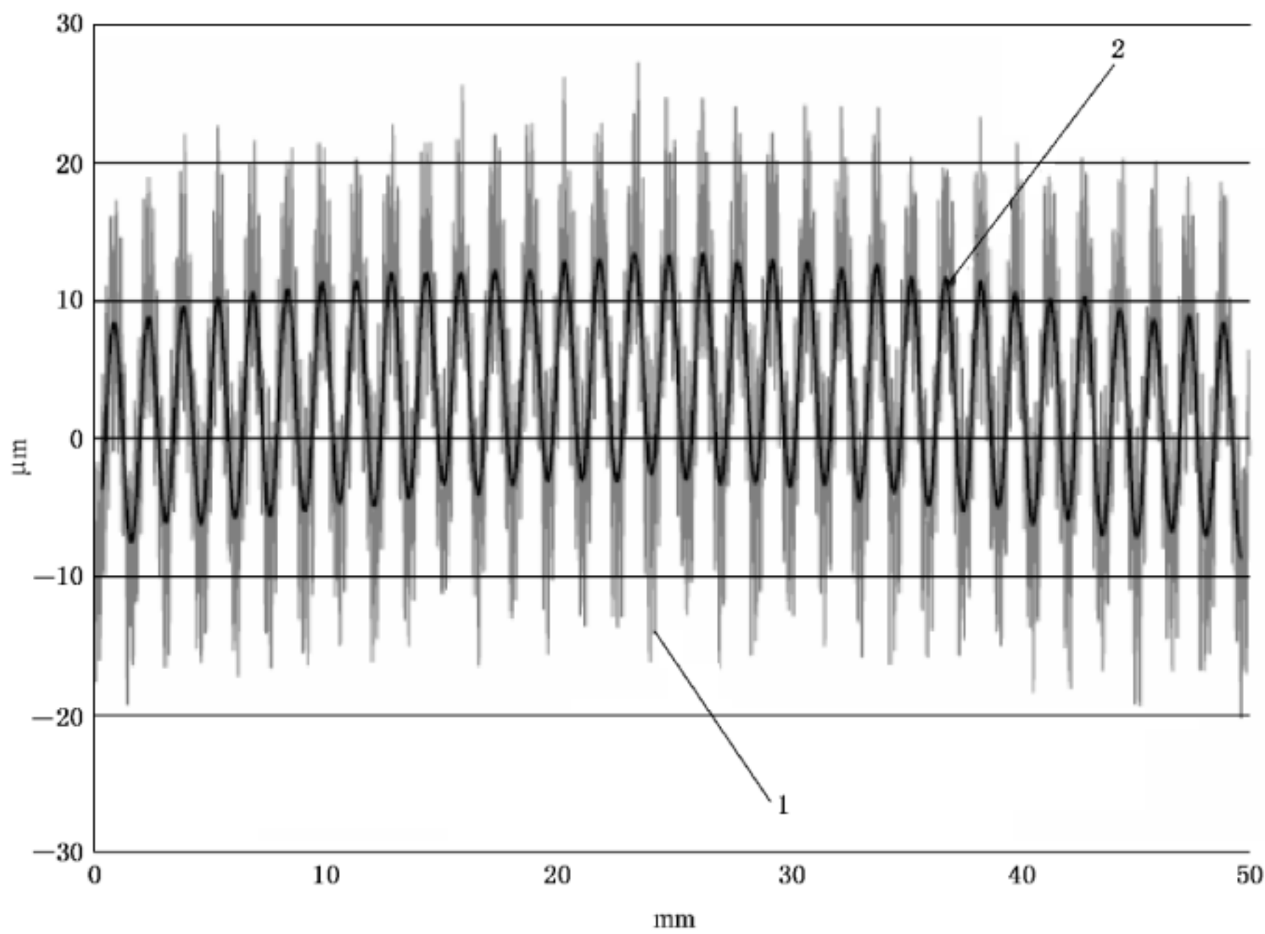
a) 0.8 mm 的长波通高斯滤波器 图 E.6 经高斯滤波器滤波后的表面轮廓
