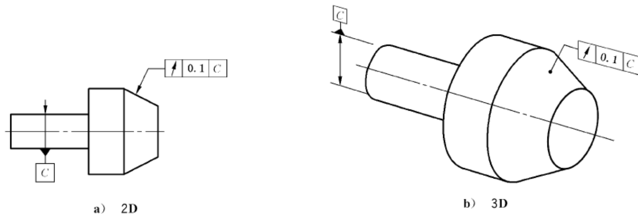
图 179 圆跳动标注
