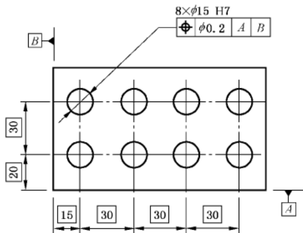
图 64 线性 TED 的标注
