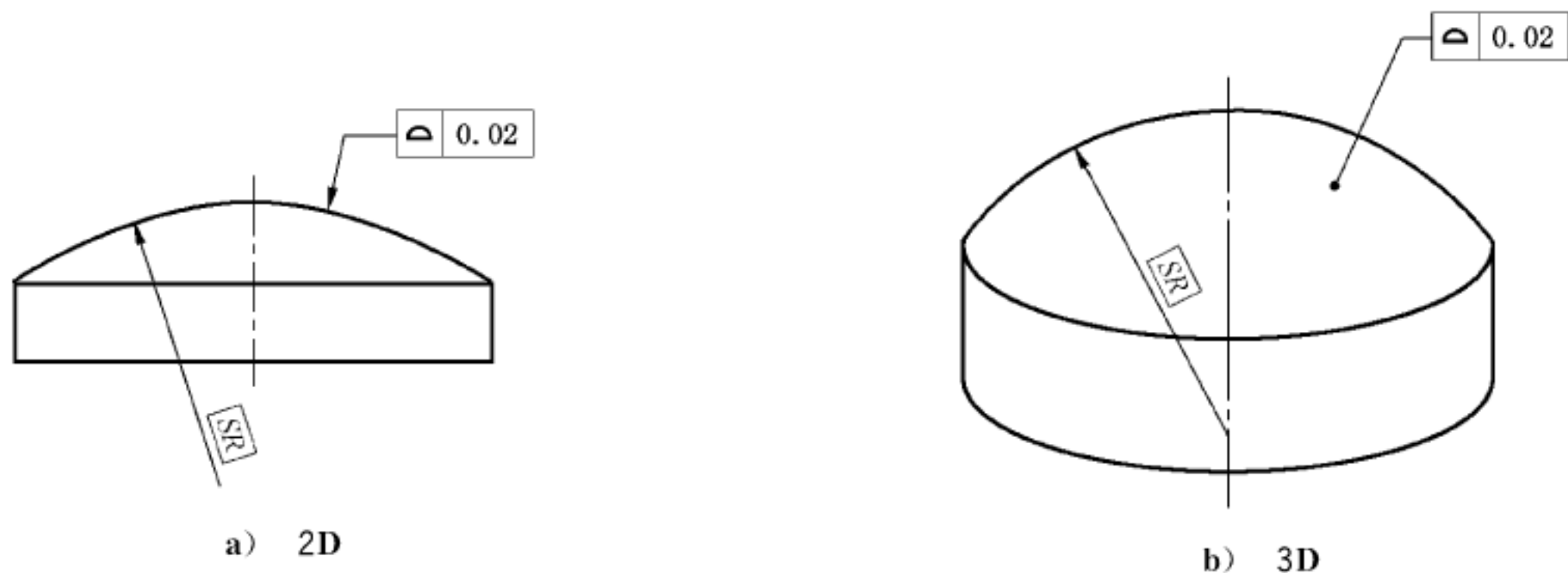
图 108 面轮廓度标注
