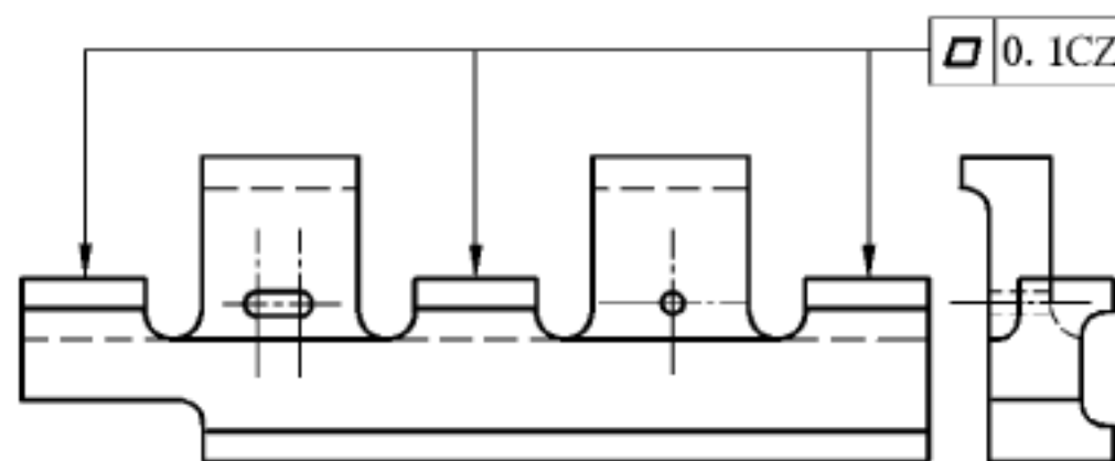
图 19 适用于多个要素的组合公差带规范
