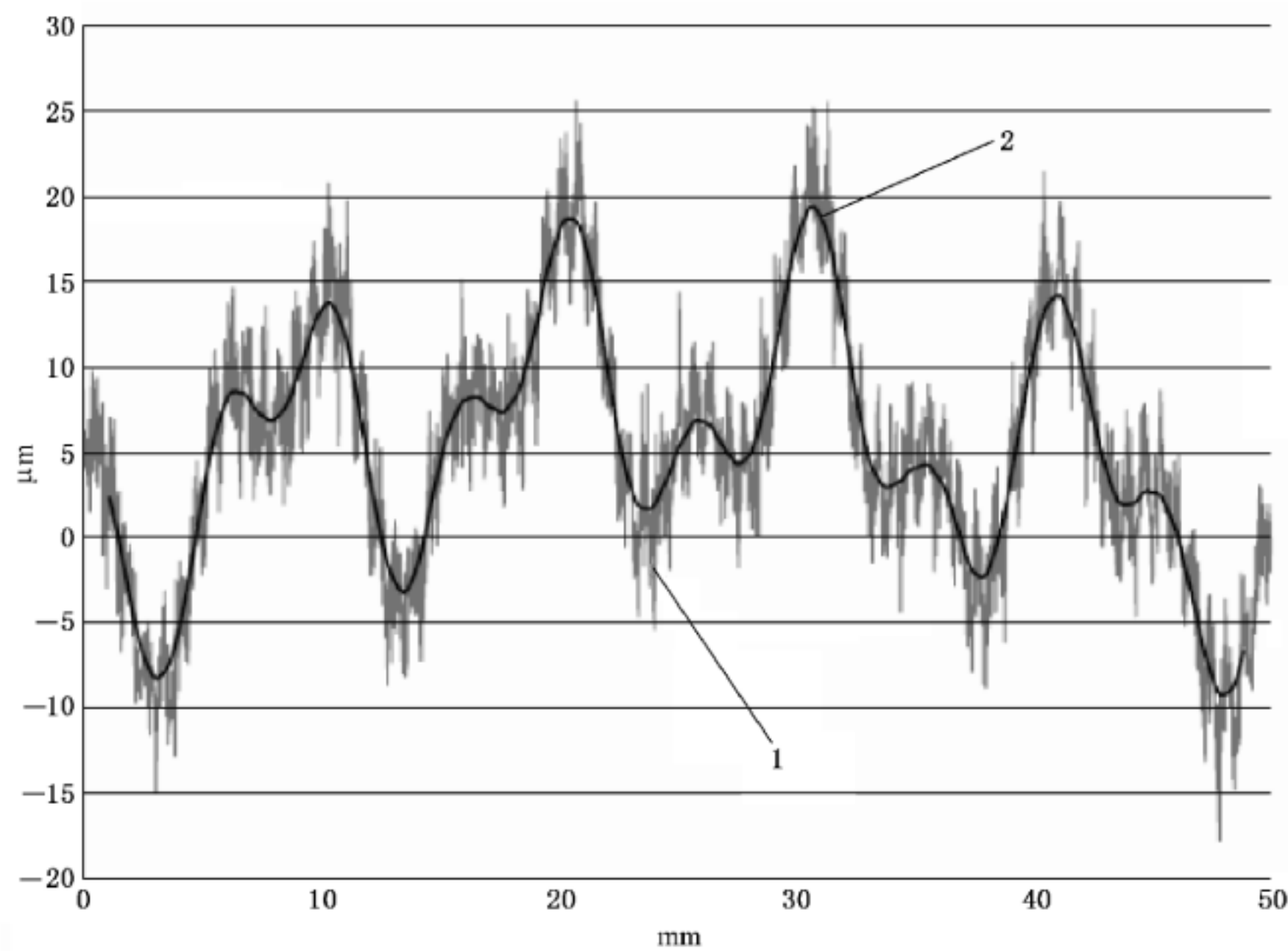
b) 2.5 mm 的长波通高斯滤波器
