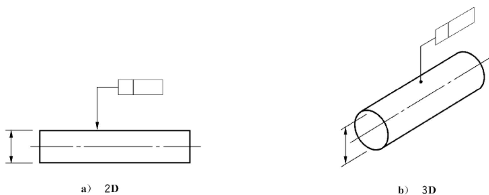
图2 组成要素的标注
