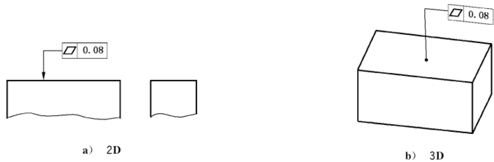
图 96 平面度标注
