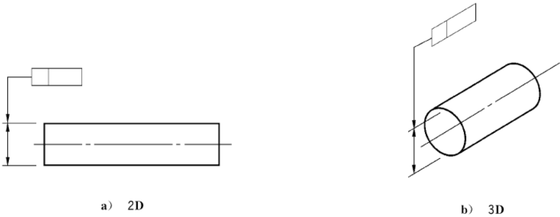
图 4 导出要素的标注
