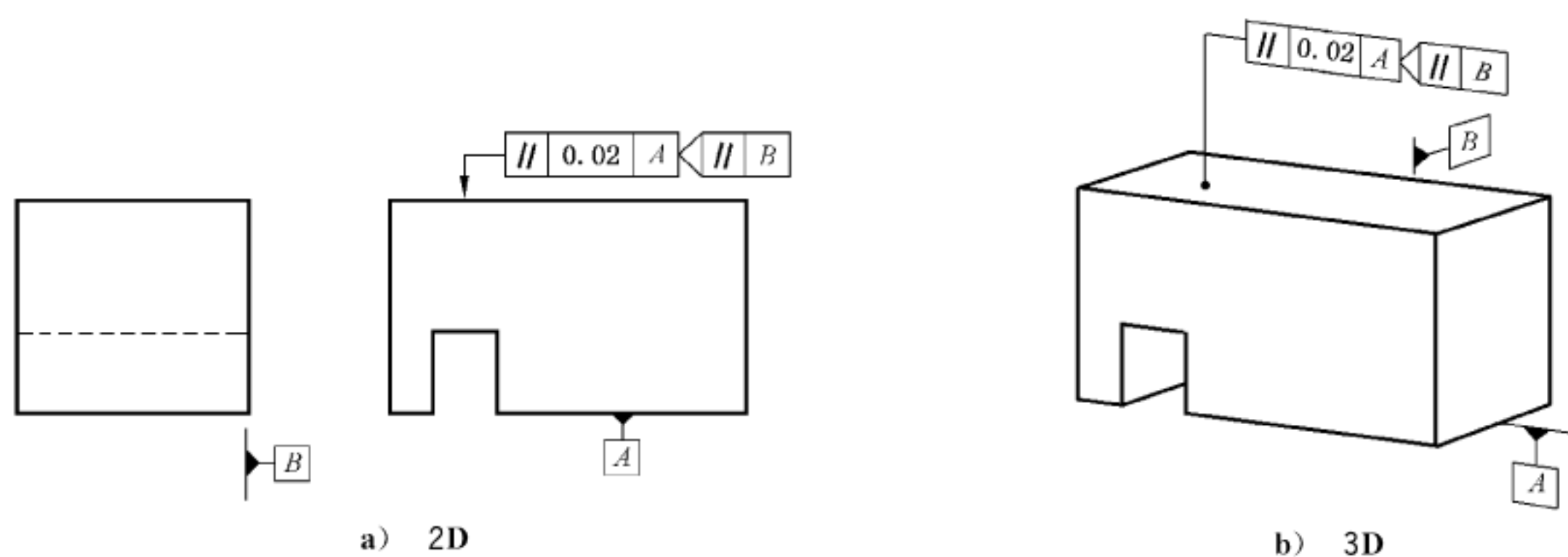
图 122 平行度标注
