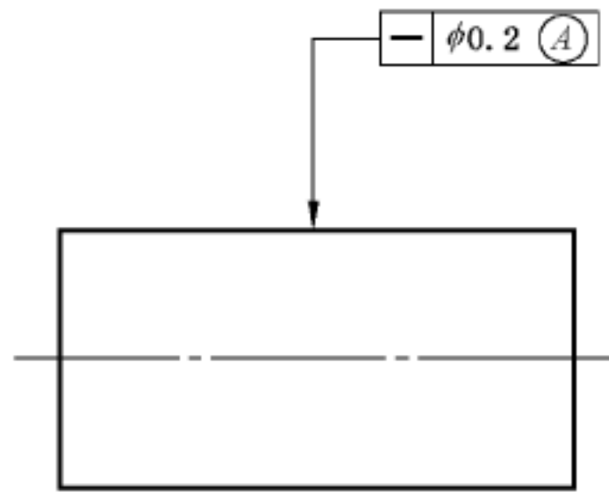
图 37 适用于中心要素的规范
