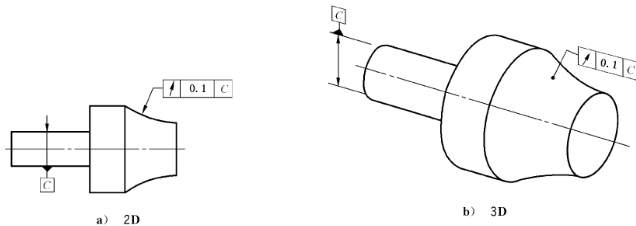
图 180 圆跳动标注
