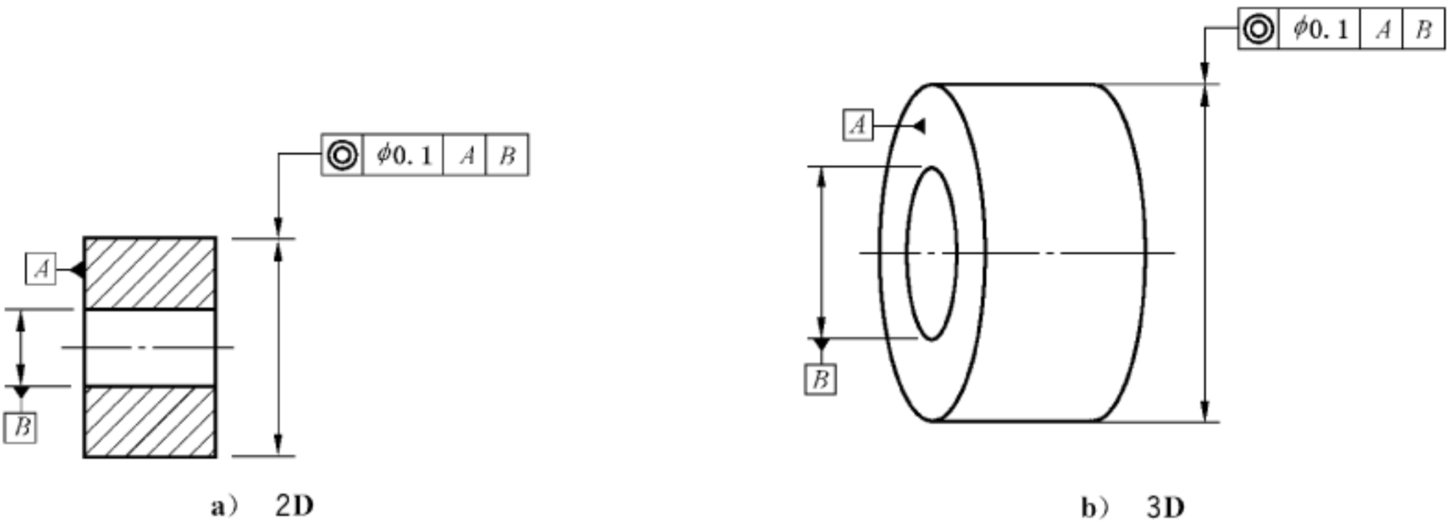
图 167 同轴度标注
