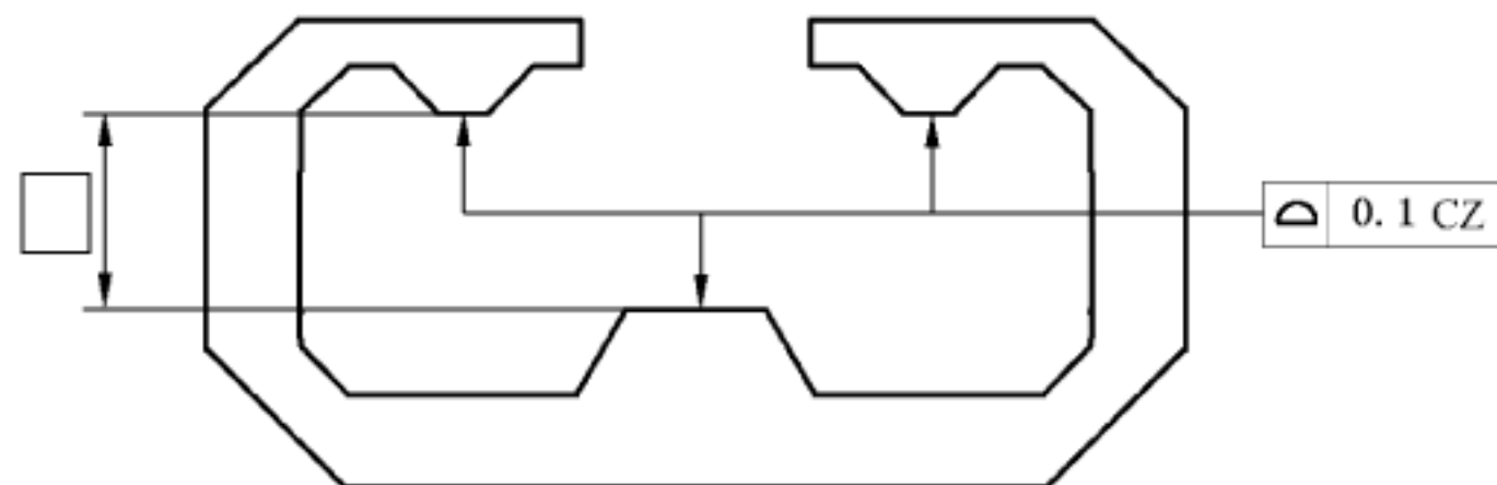
图 19 适用于多个要素的组合公差带规范
