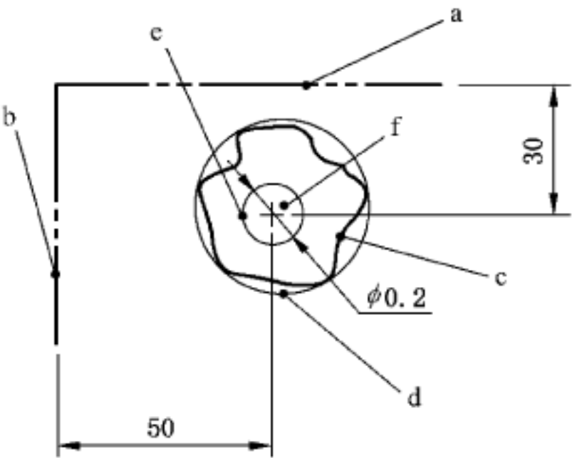
图 29 最小外接拟合被测要素——图样标注
