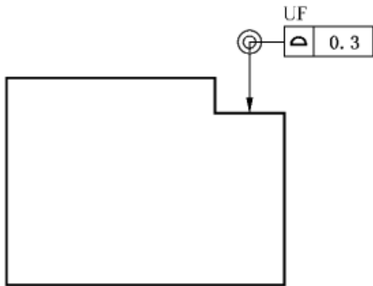
注：图样未标注完整。轮廓的公称几何形状未定义。
