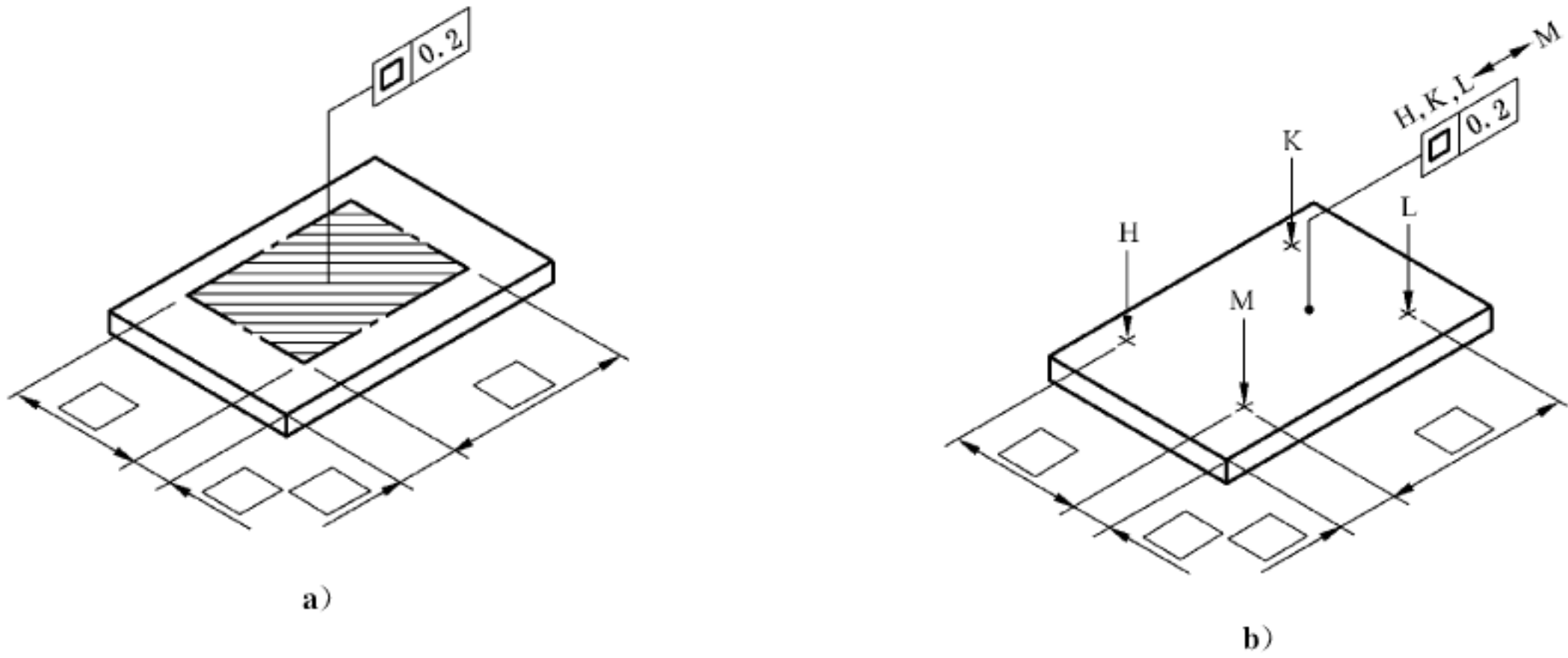
图 57 局部区域标注
