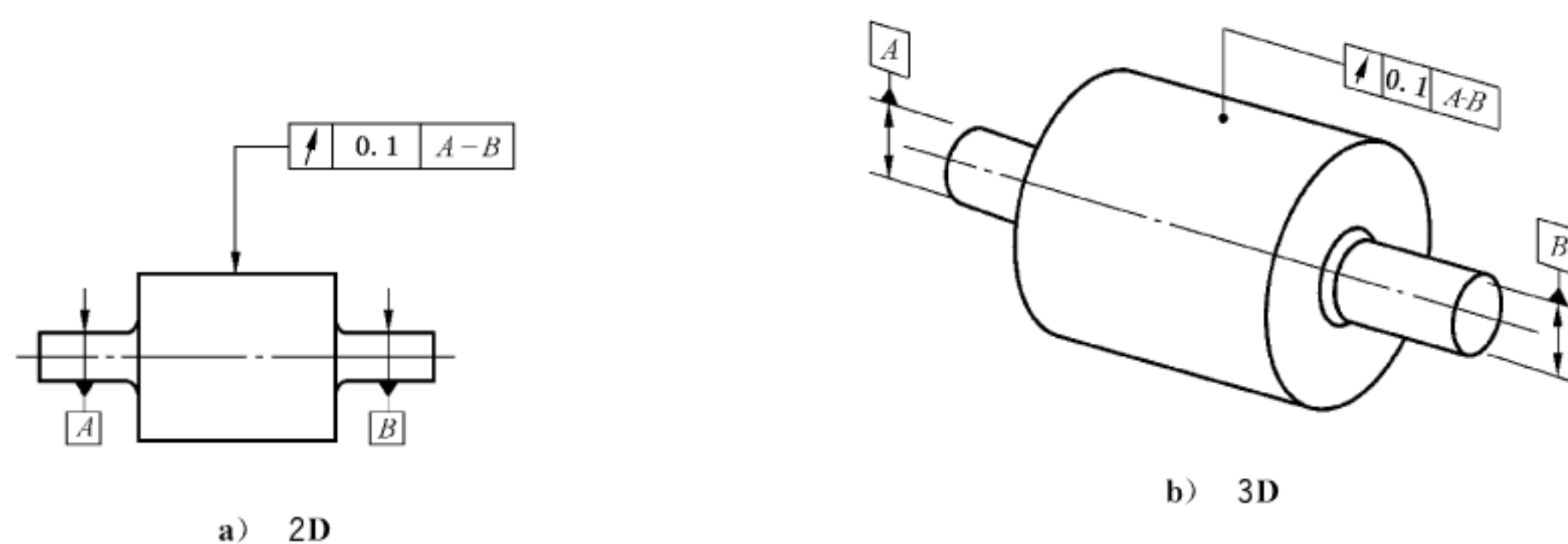
图 174 圆跳动标注
