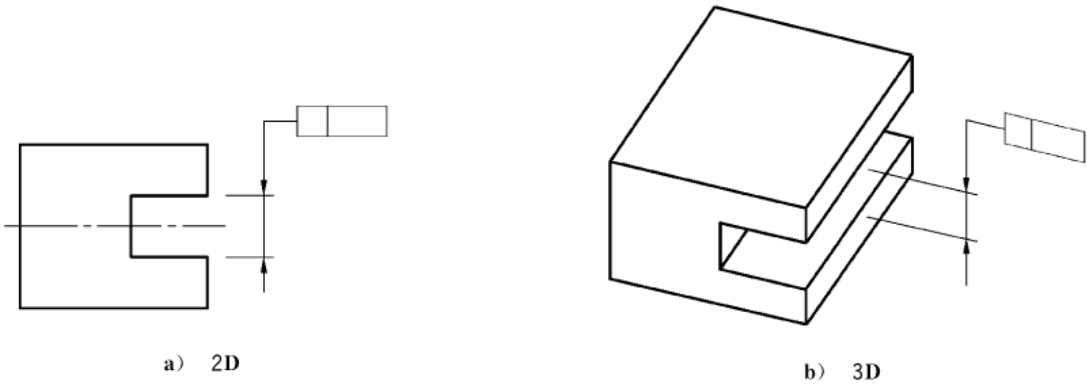
图 6 导出要素的标注
