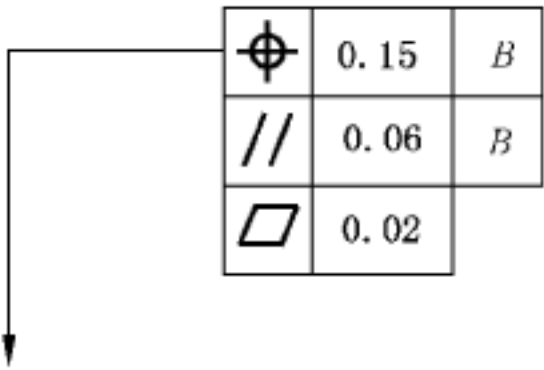
图 50 多层公差标注
