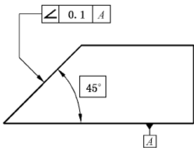
图 65 角度 TED 的标注
