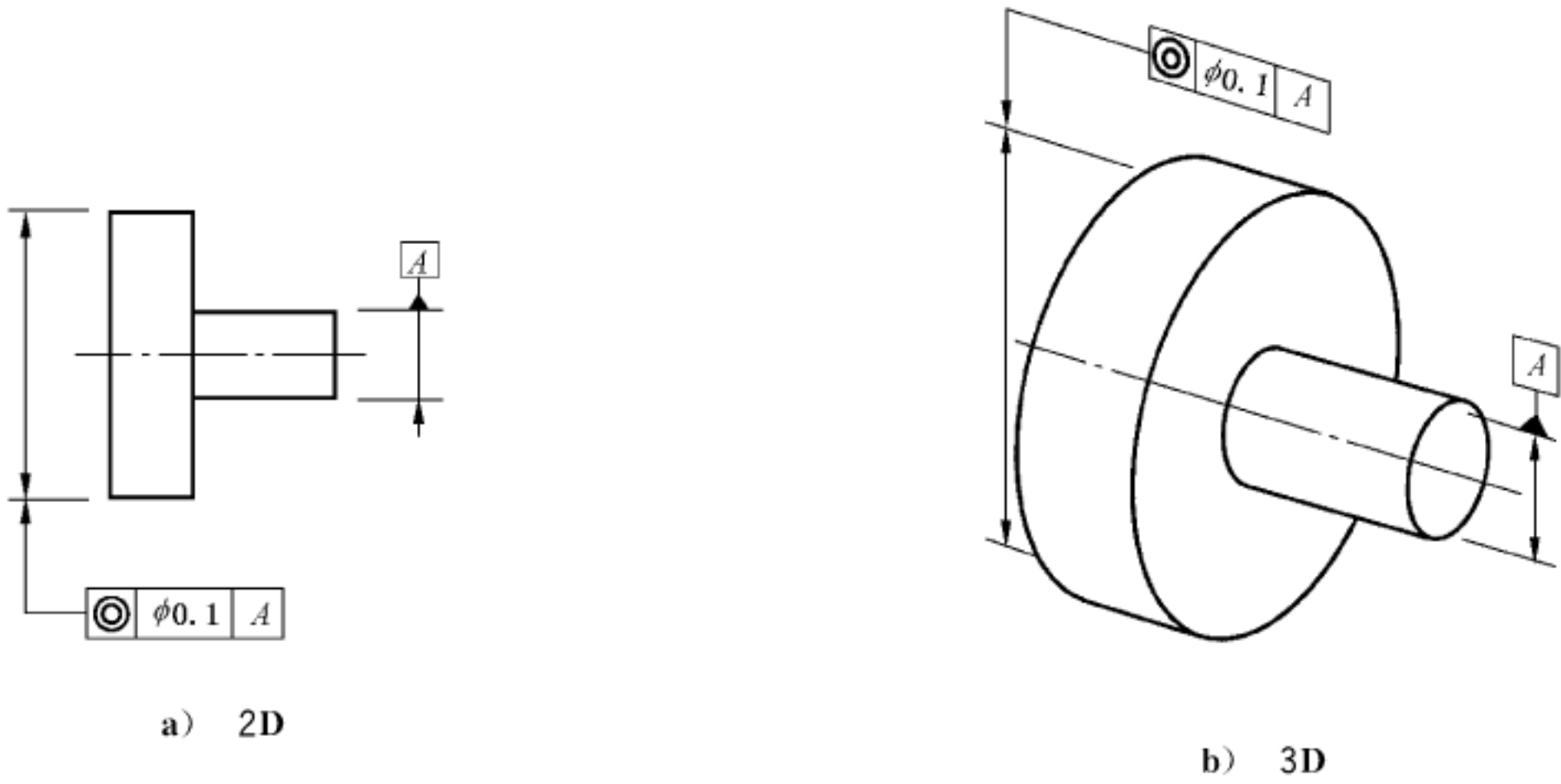
图 166 同轴度标注
