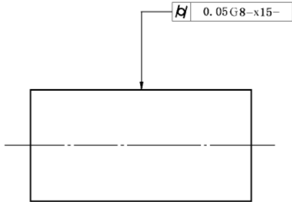
图 E.16 圆度公差示例——高斯滤波器
