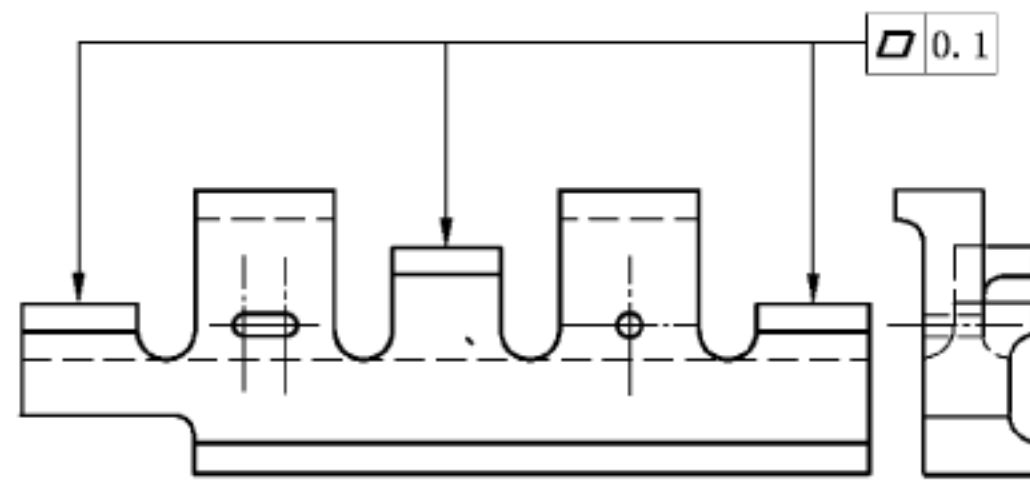
图 17 适用于多个单独要素的规范
