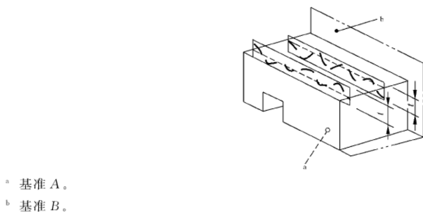
图 123 平行度公差带的定义
