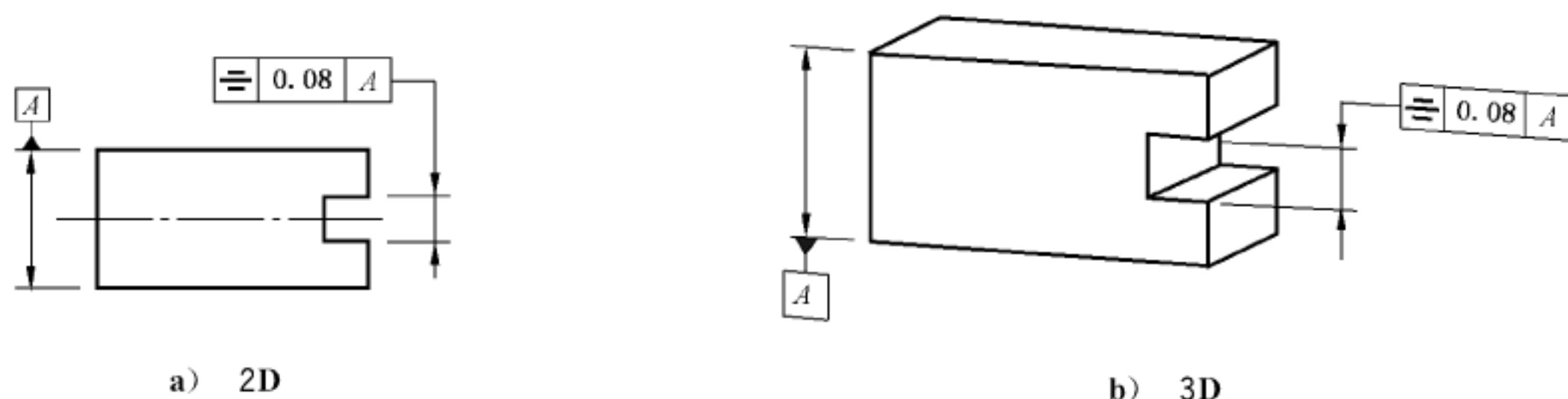
图 169 对称度标注
