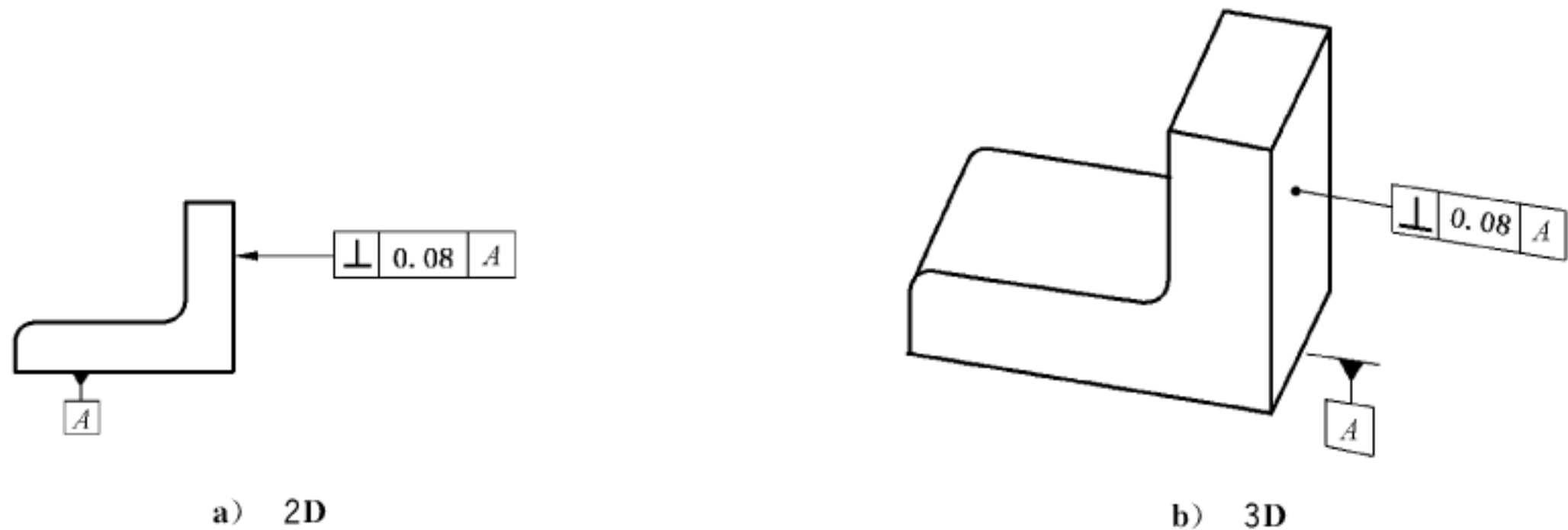
图 138 垂直度标注
