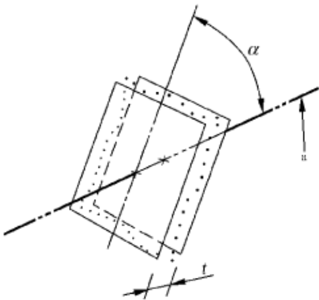
图 147 倾斜度公差带的定义
