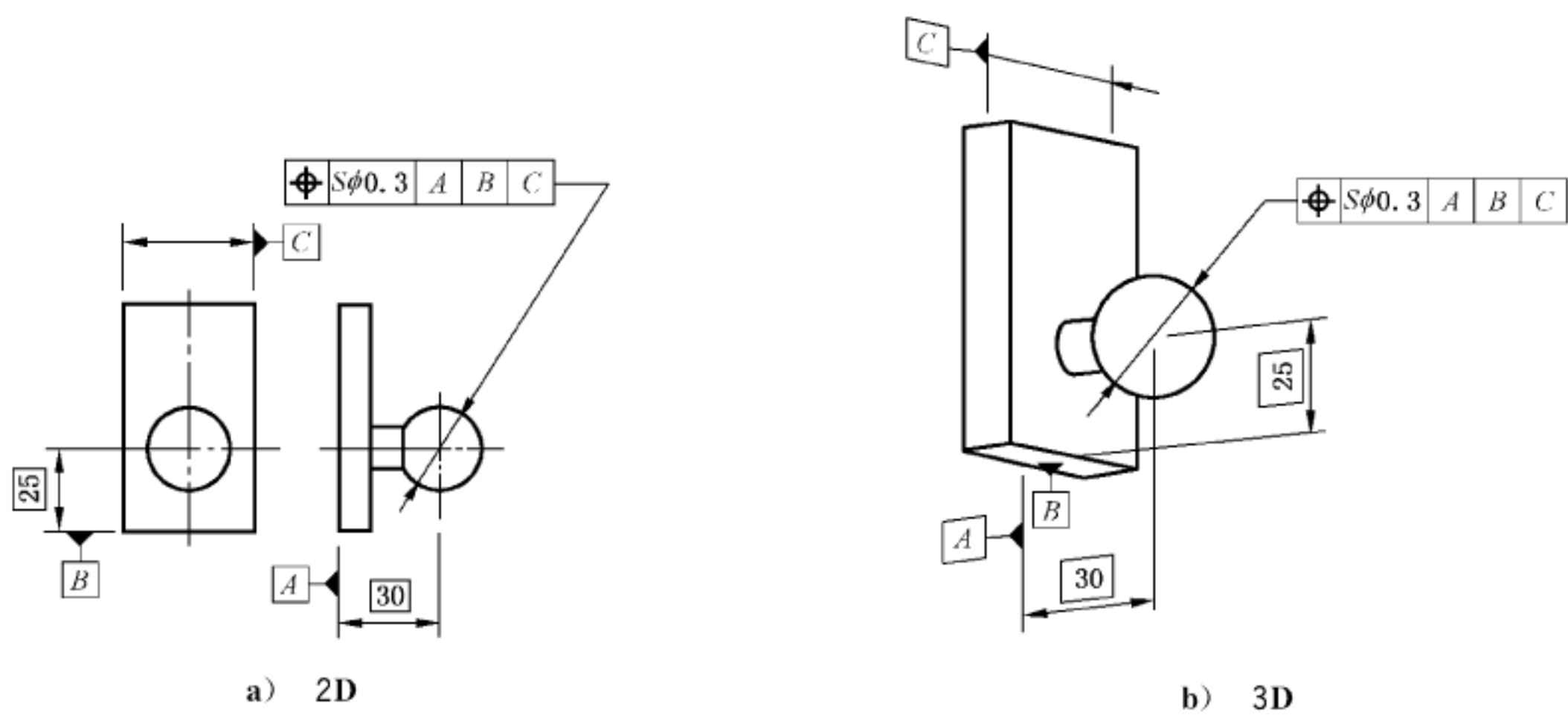
图 150 位置度标注
