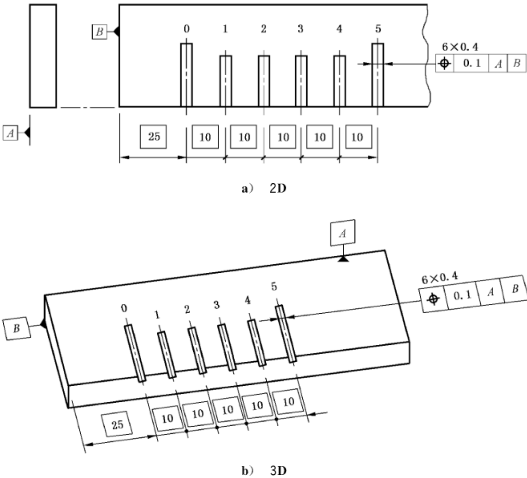
图 157 位置度标注
