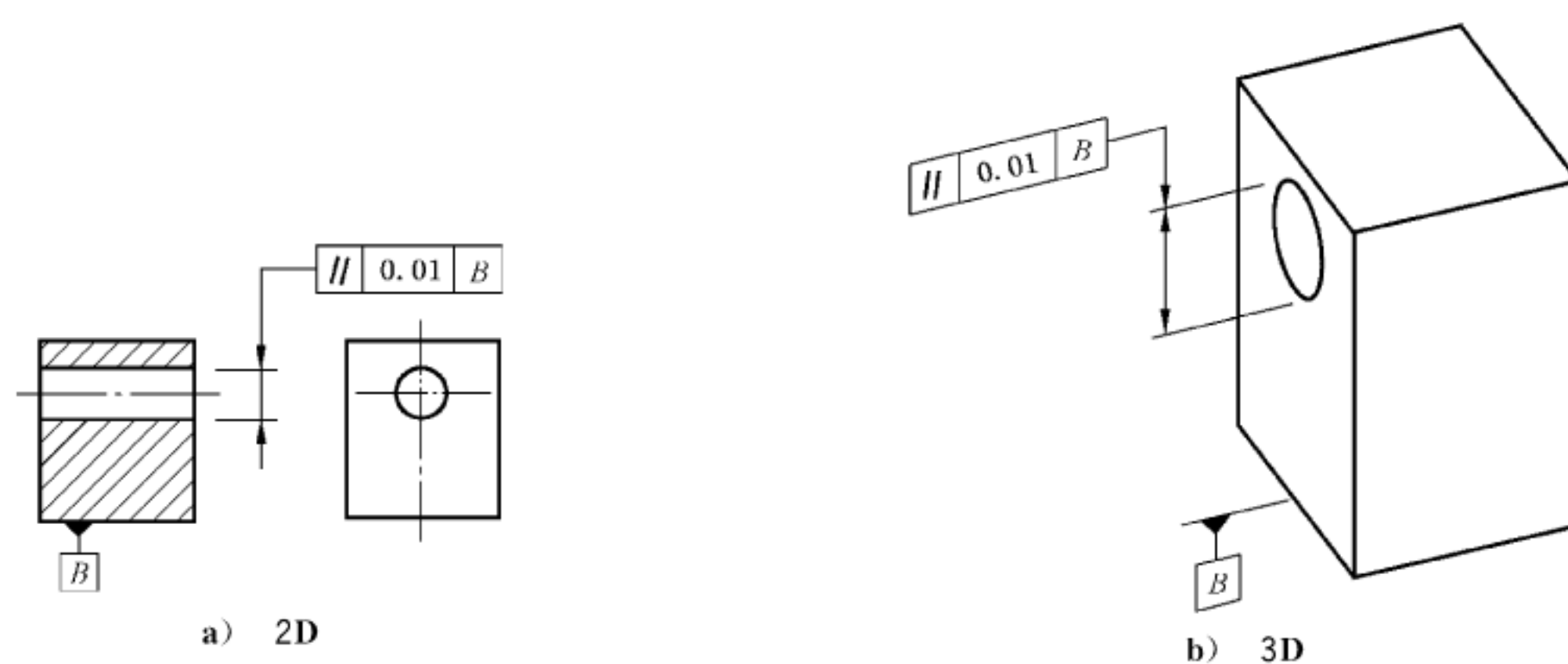
图 120 平行度标注
