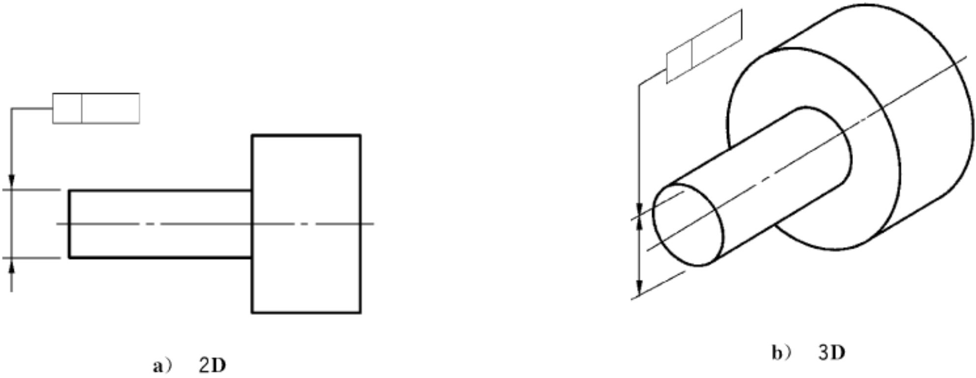
图 5 导出要素的标注
