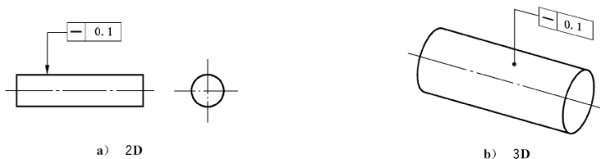
图 92 直线度标注
