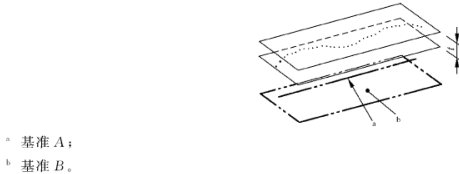
图 113 平行度公差带的定义
