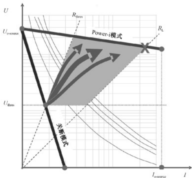
图 A.3 在负载连接期间 Power-i 电源的特性曲线输出设置示例
