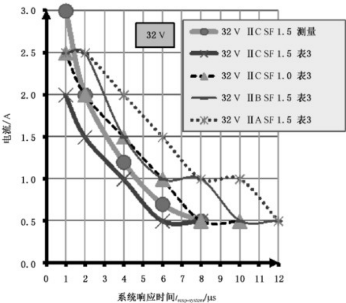
图 A.9 电压级别 32 V(32 VDC)的 Power-i 点燃曲线
