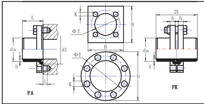
尺寸参数
