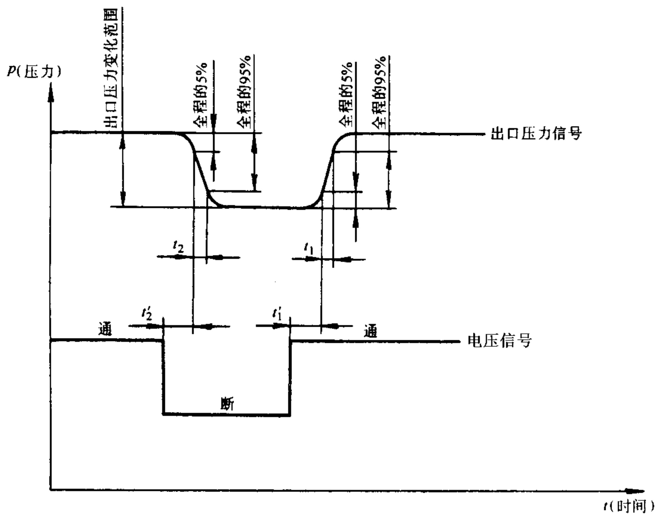
图 A.7 出口压力—时间瞬态响应曲线
