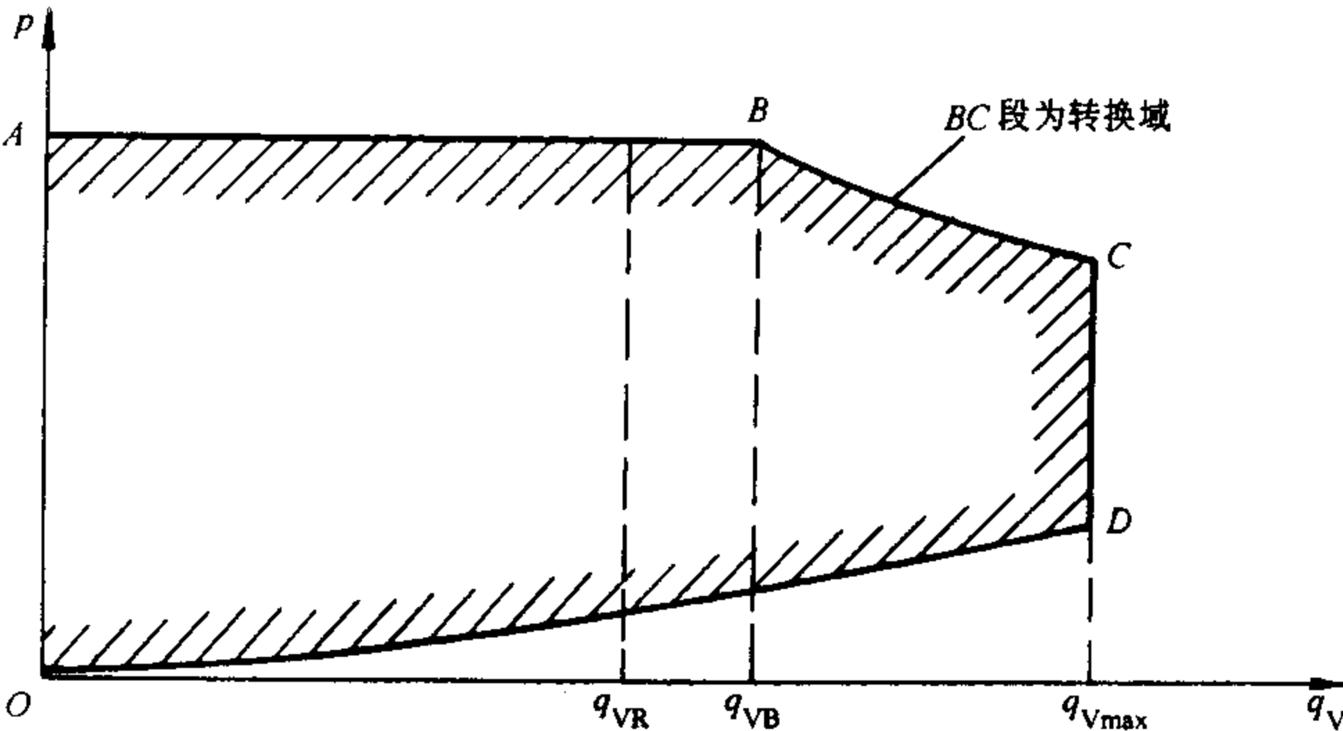
图 A.4 工作范围图
