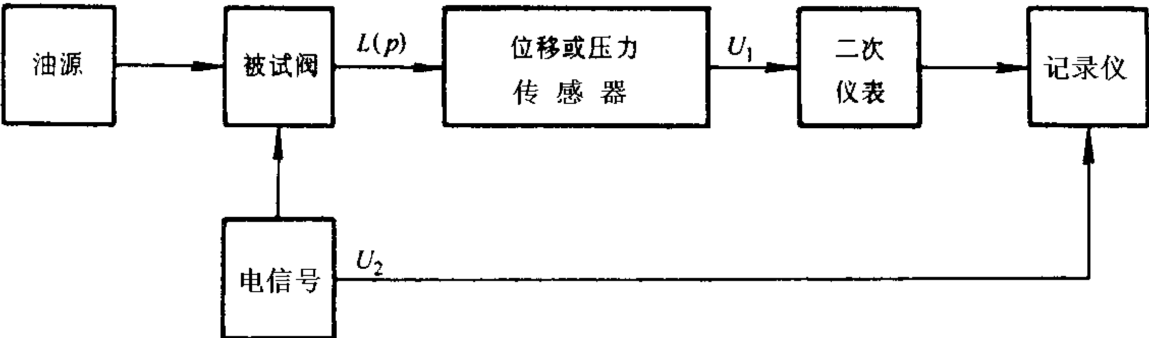
图 A.5 测试系统方框图
