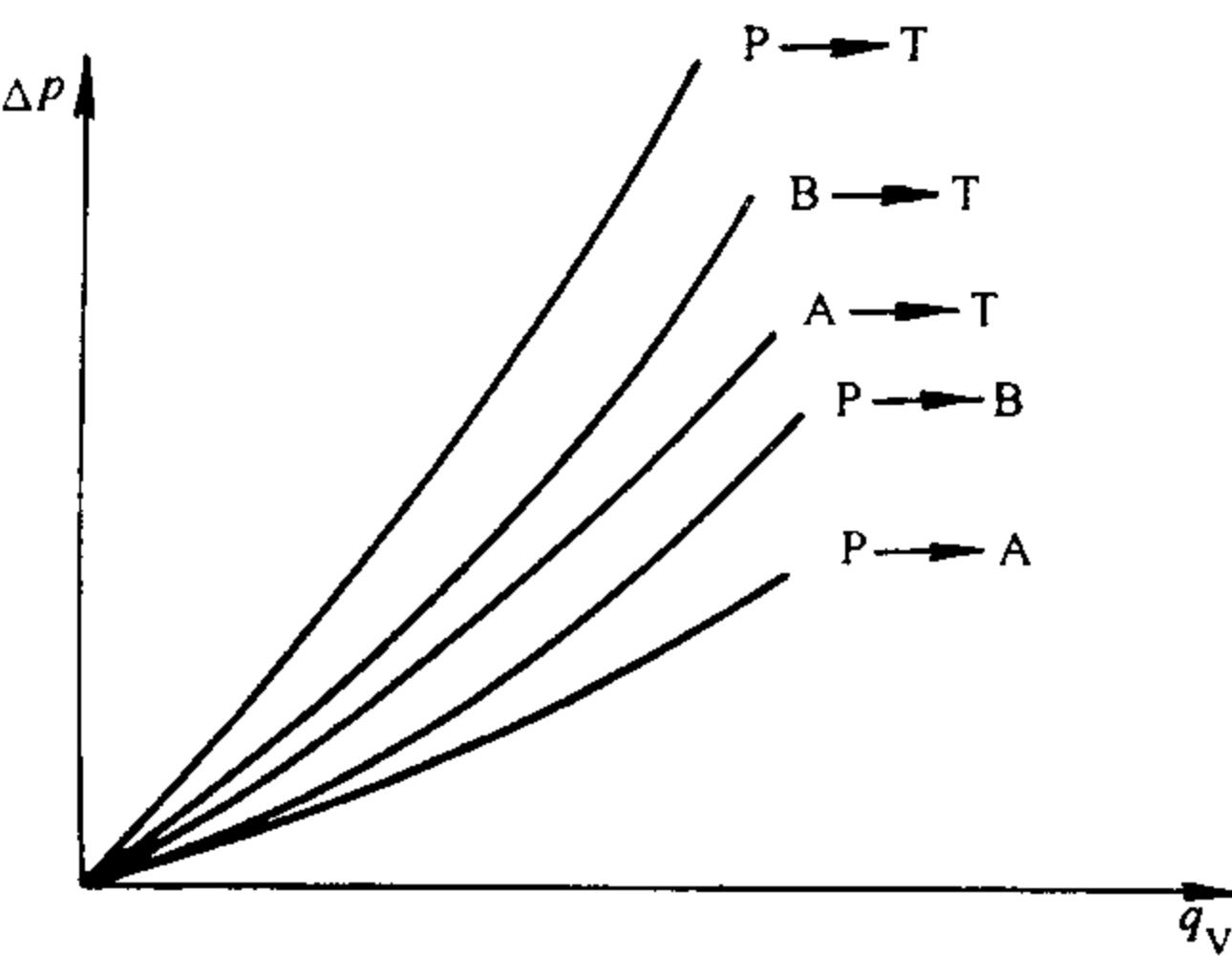
图 A.2 流量—压力损失曲线
