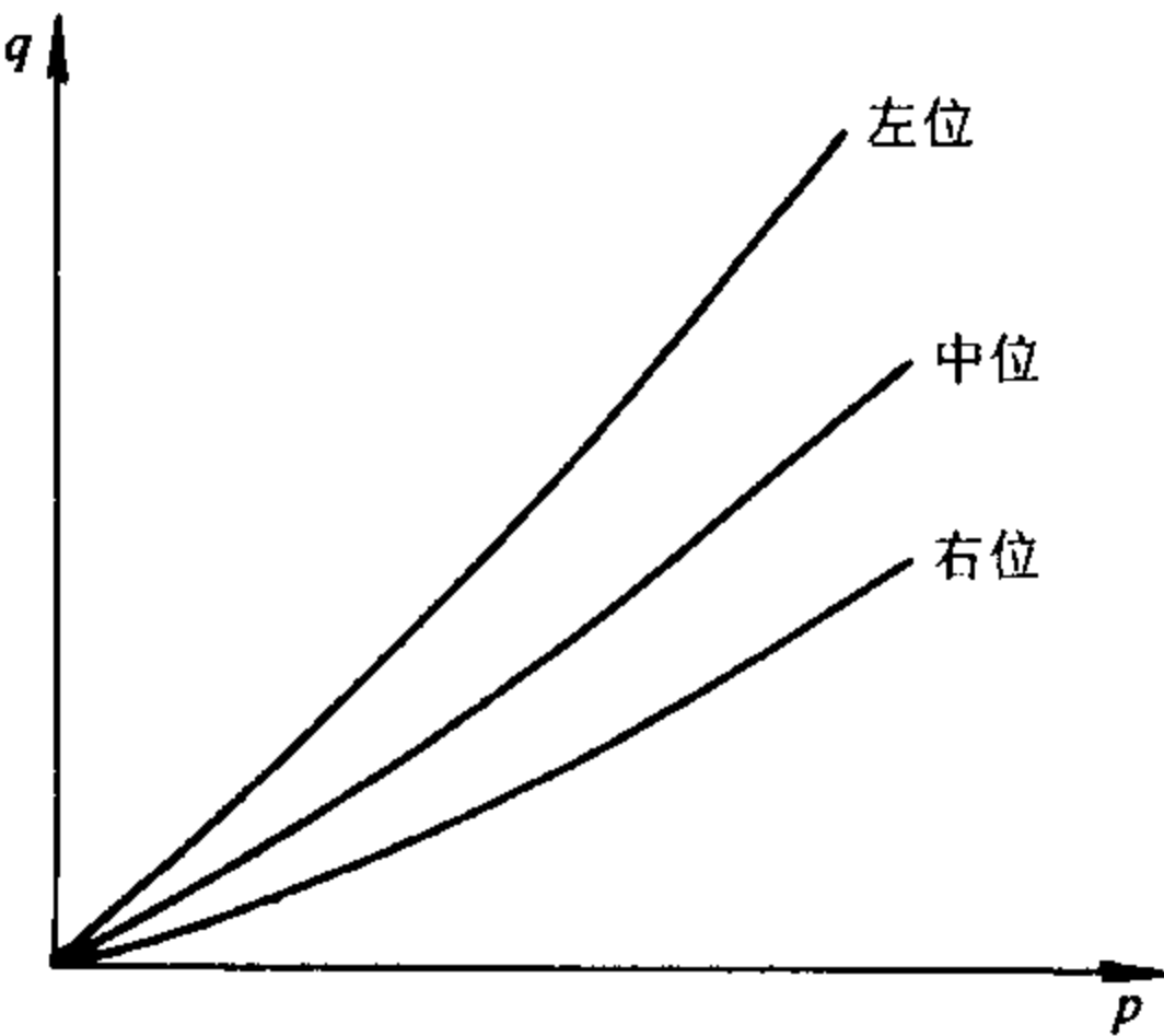
图 A.3 压力—内泄漏量曲线
