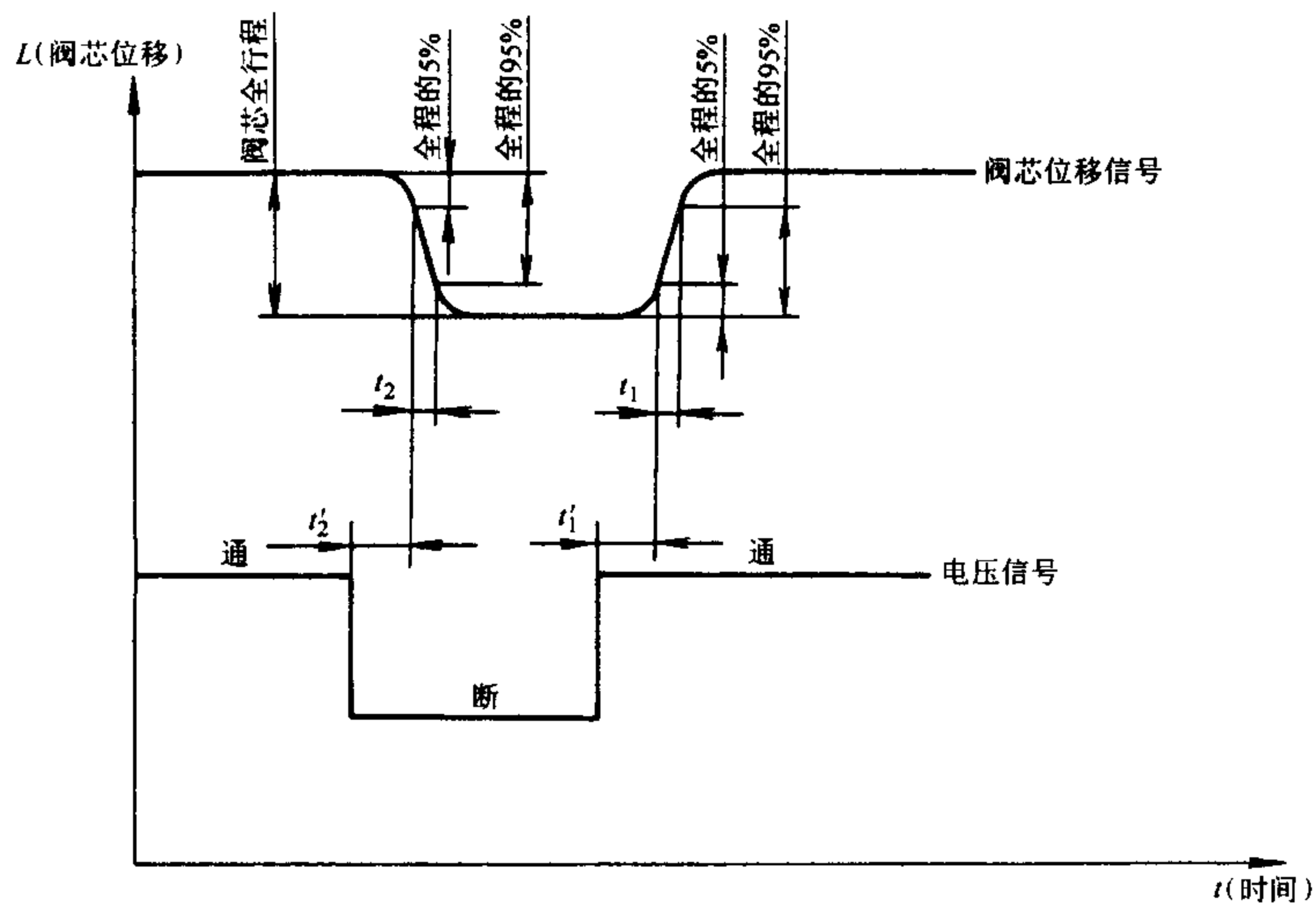
图 A.6 阀芯位移—时间瞬态响应曲线
