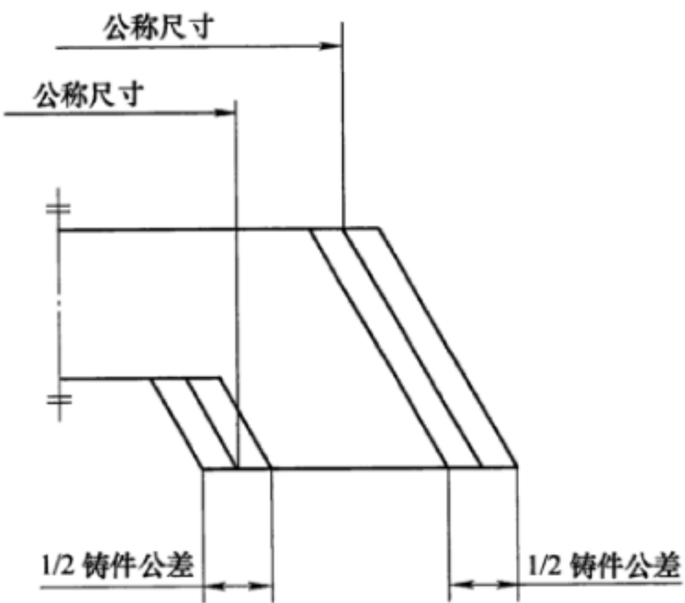
图 2 沿倾斜面对称布置的公差带
