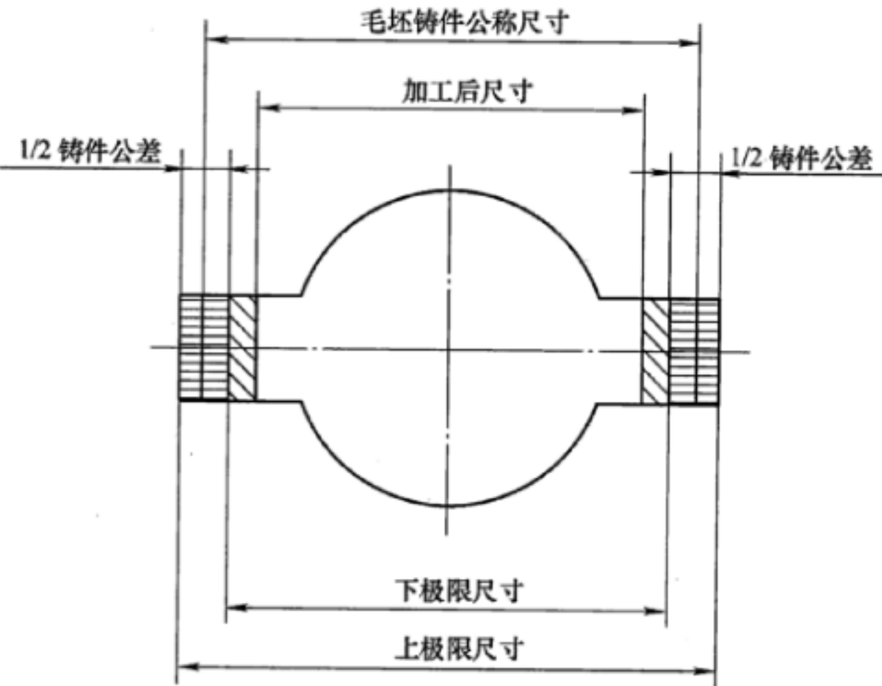
图 1 对称布置公差带
