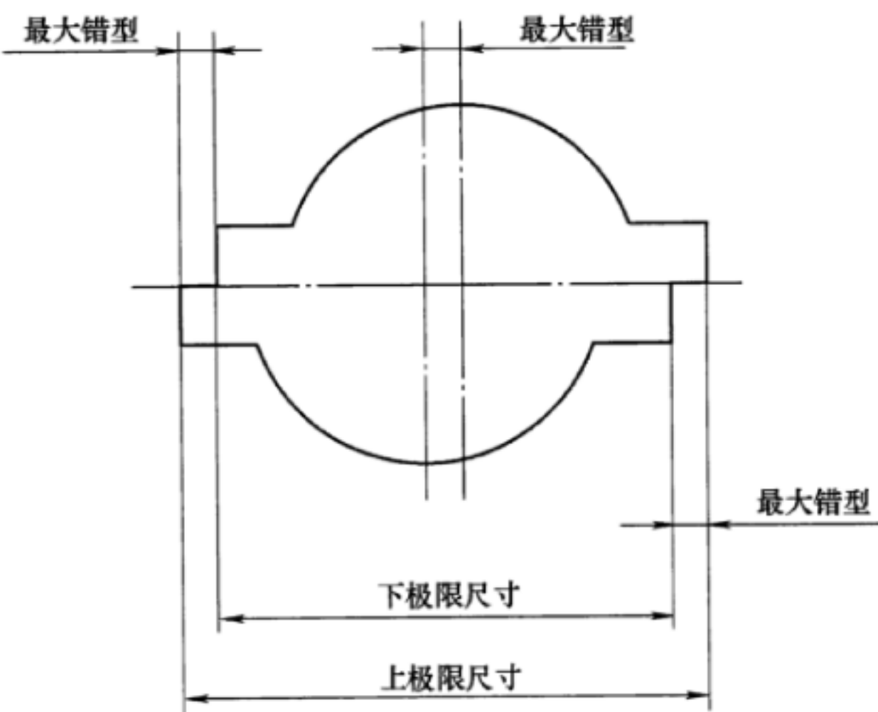
图 3 铸件允许的最大错型值
