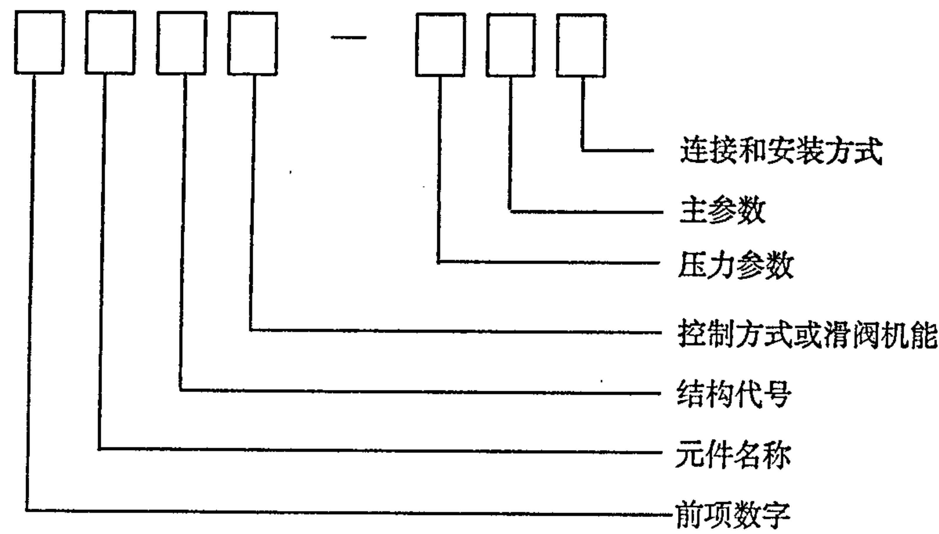
图 1 液压元件型号的基本组成
