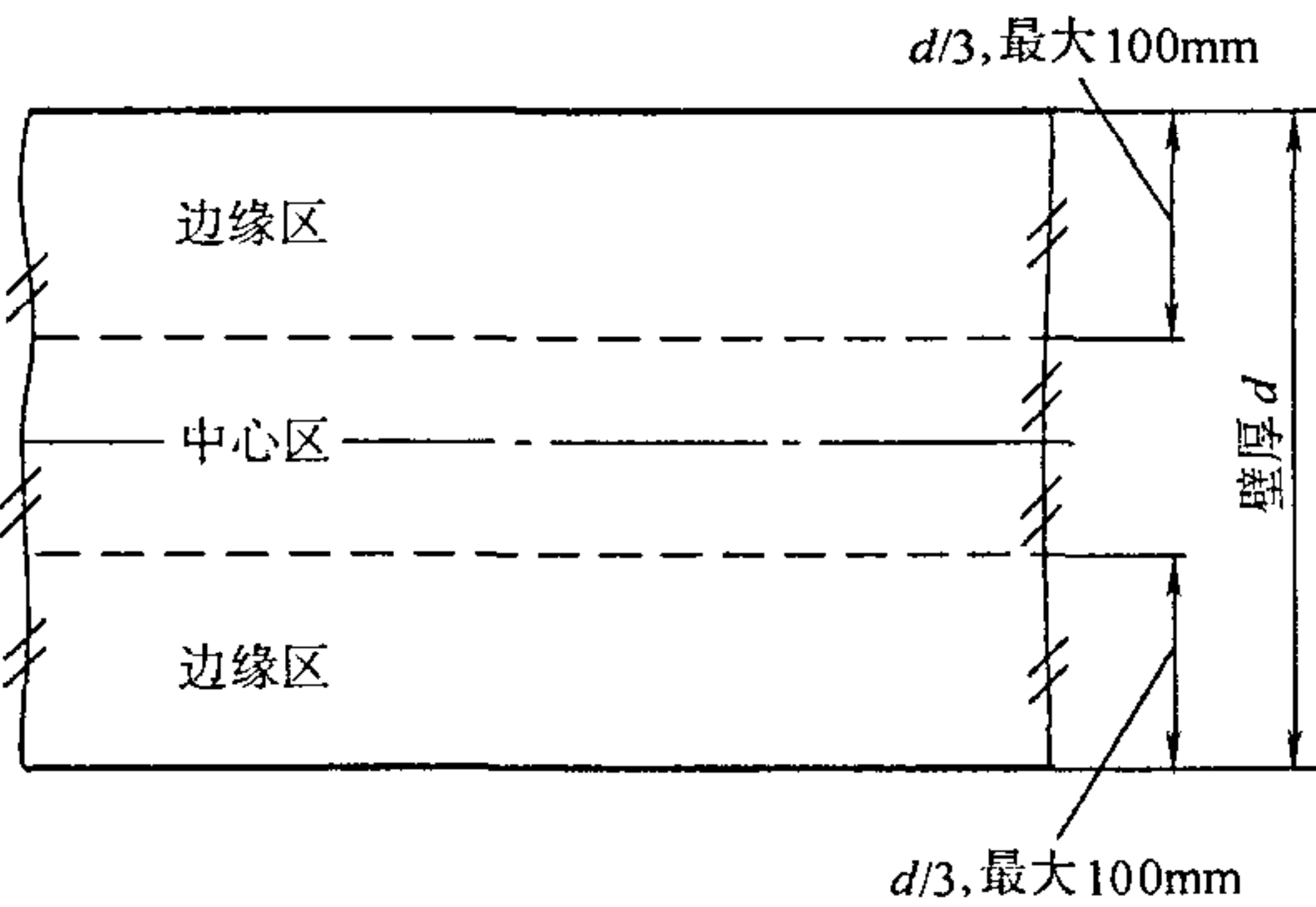
图 1 铸件壁厚区域划分 （壁厚区域的划分以铸件加工后的尺寸为基准）
