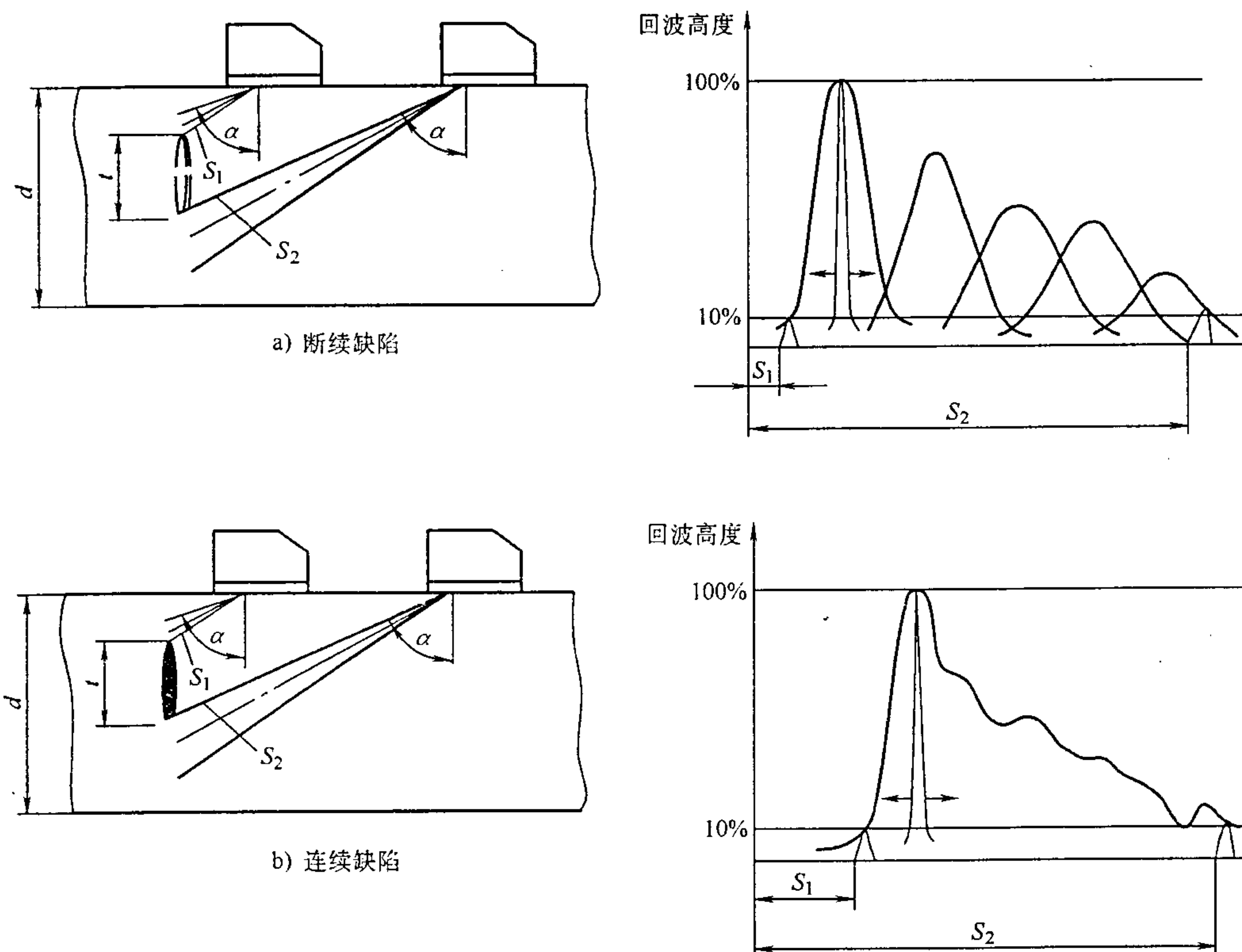
图 C.3 斜探头测定垂直于受检面的延伸性缺陷的延伸尺寸和回波动态
