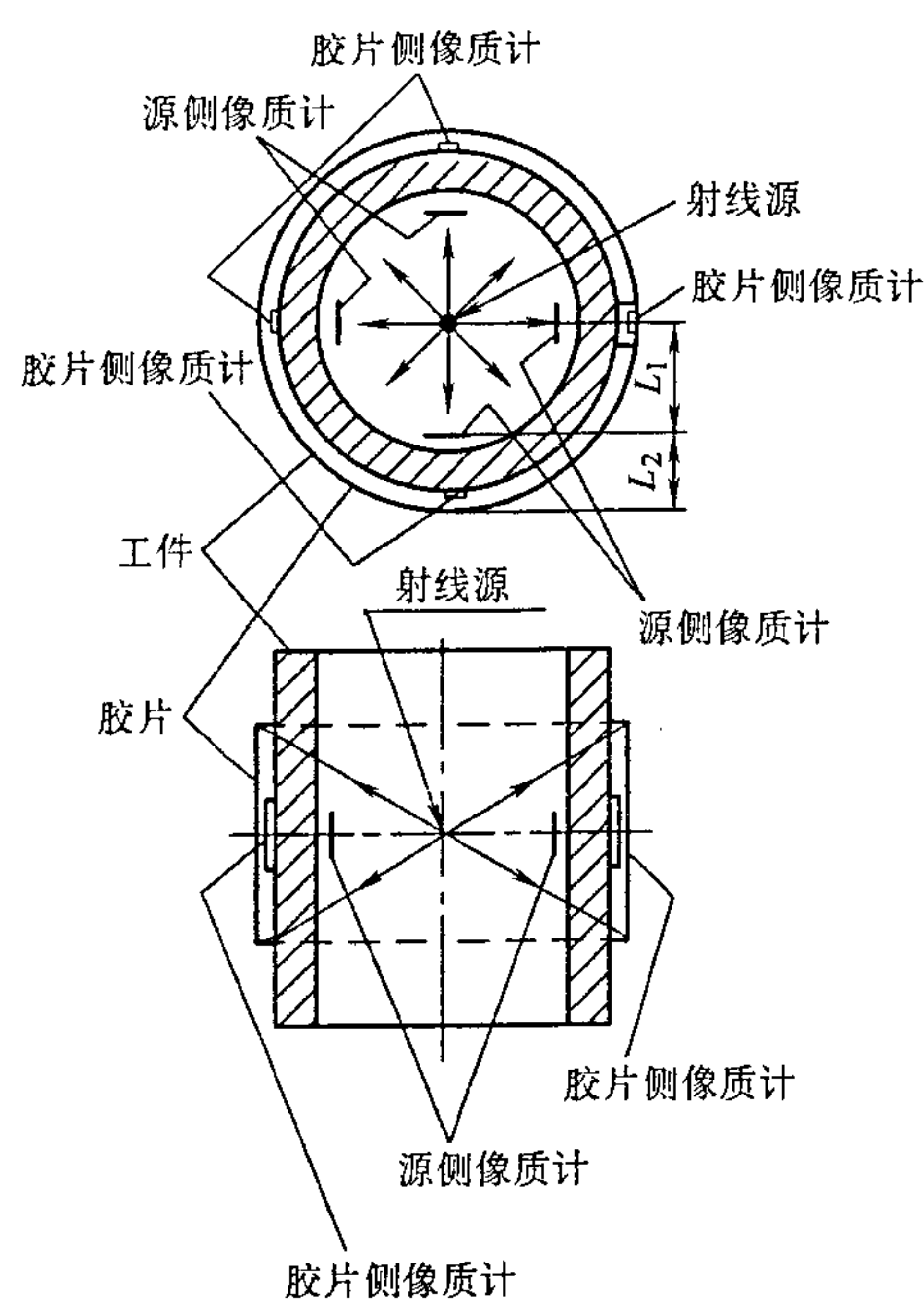
图 D.2 筒形工件照相布置（内透法）
