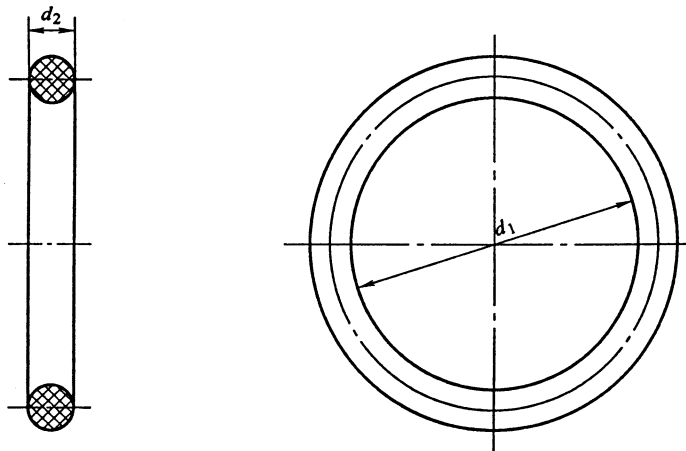
图 1 O 形橡胶密封圈
