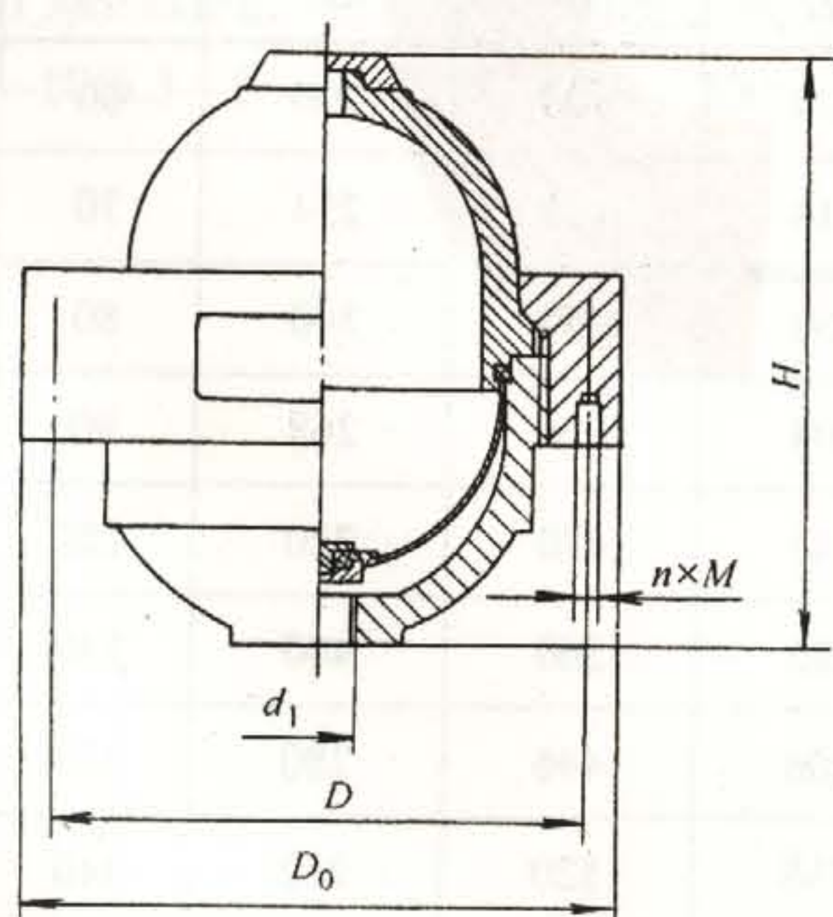
图1 A型蓄能器
