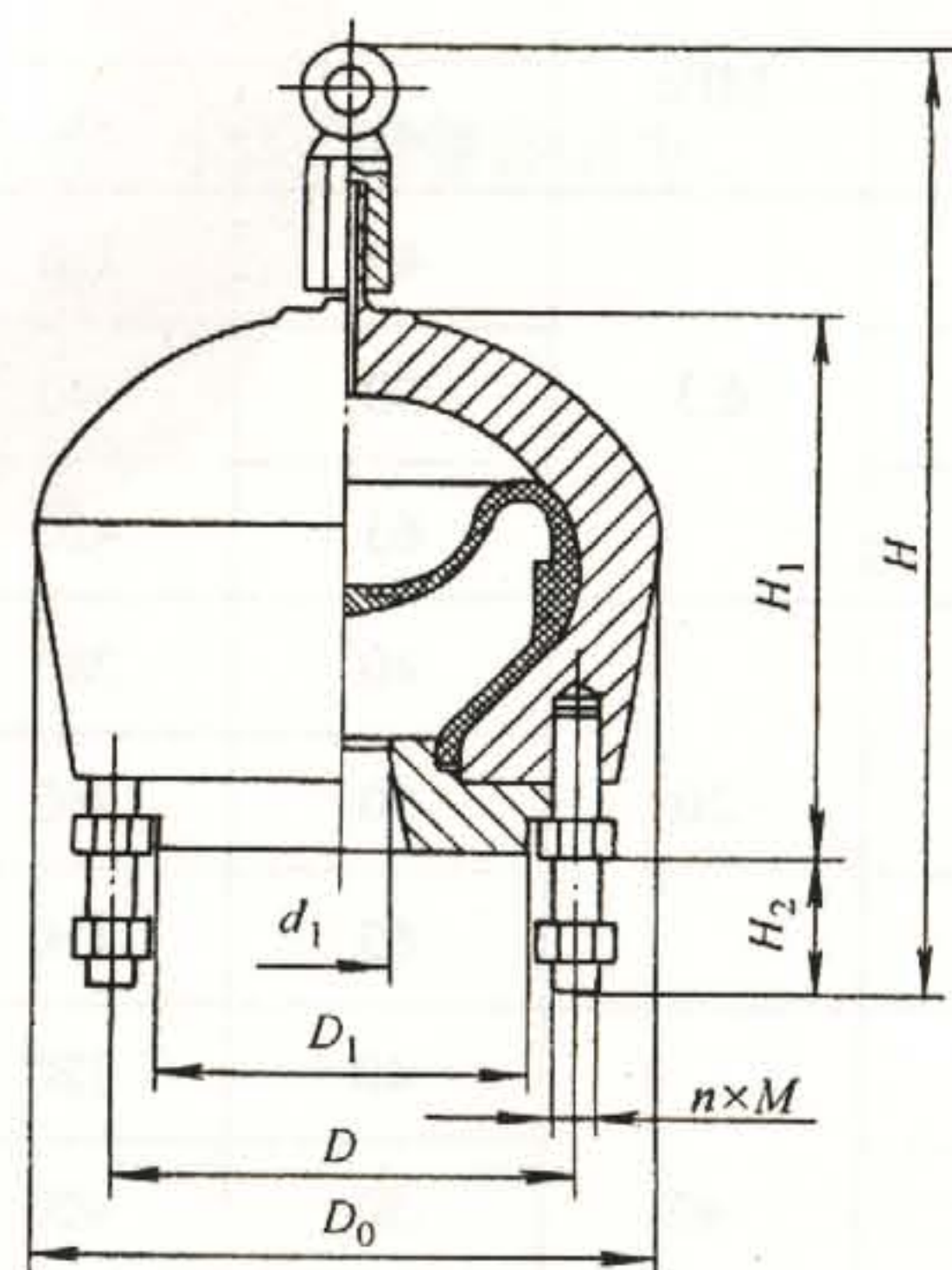
图2 B型蓄能器
