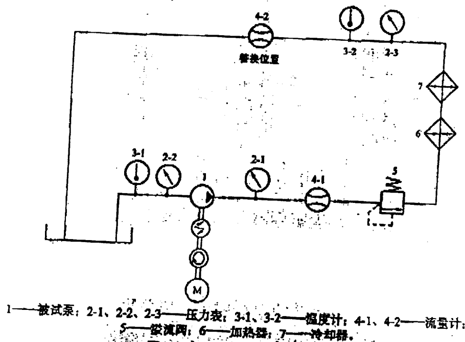
图 A.1 开式试验回路原理图
