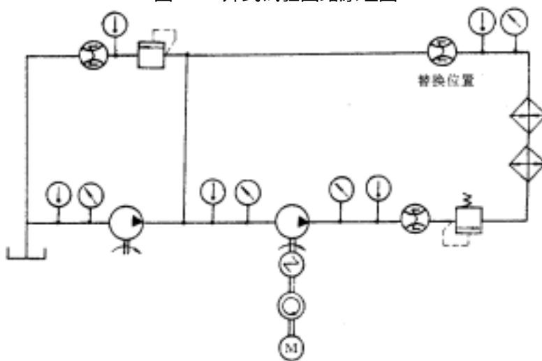
图 A2 闭式试验回路原理图
