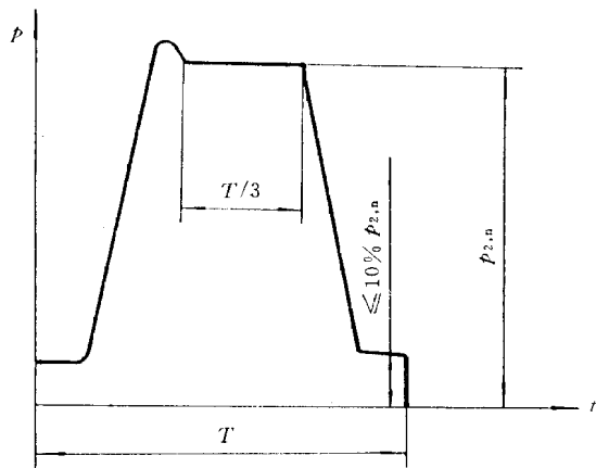
图 A7 冲击波形
