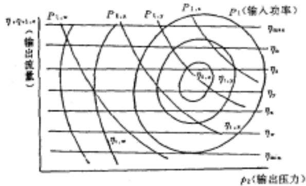
图 A3 容积效率等效率曲线
