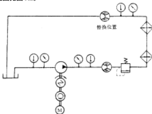
图 A1 开式试验回路原理图
