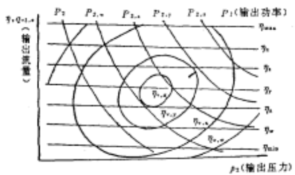
图 A4 总效率等效率曲线
