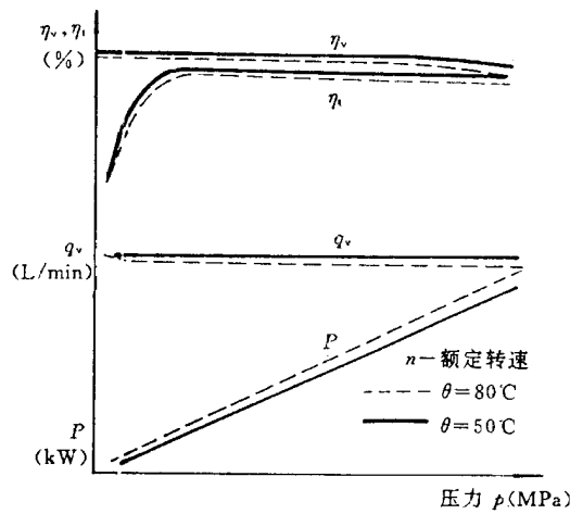
图 A6 功率、流量、效率随压力变化曲线
