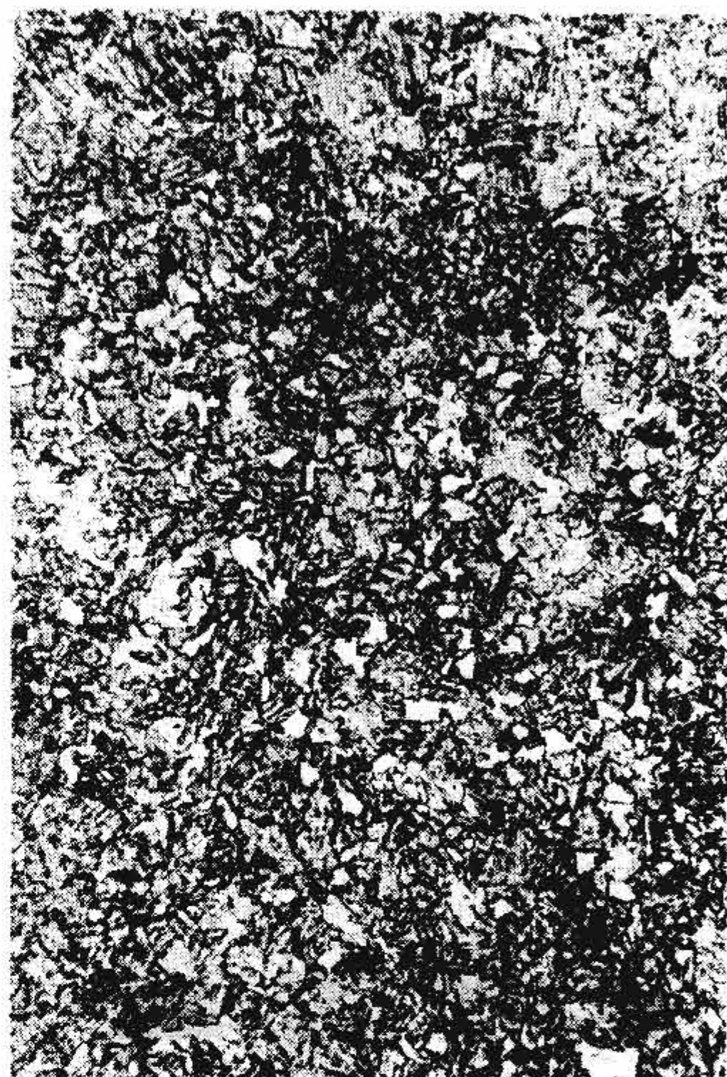
第 6 级 (较多量的块状及条状游离铁素体)
