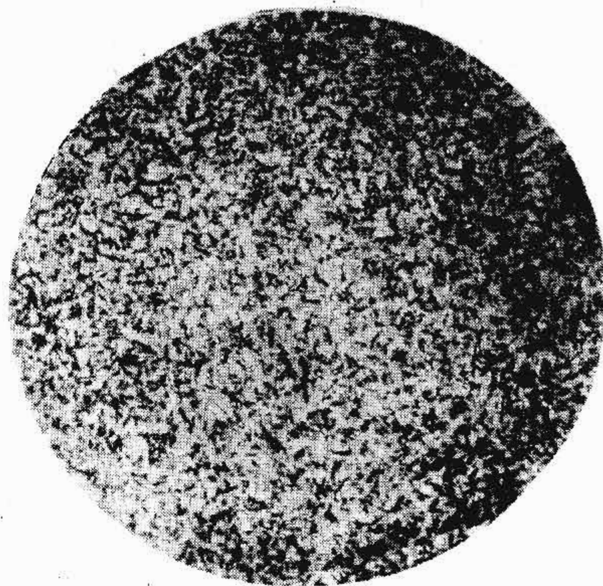
第 2 级 (细针状马氏体, 针的长度 > 1.5 mm)
