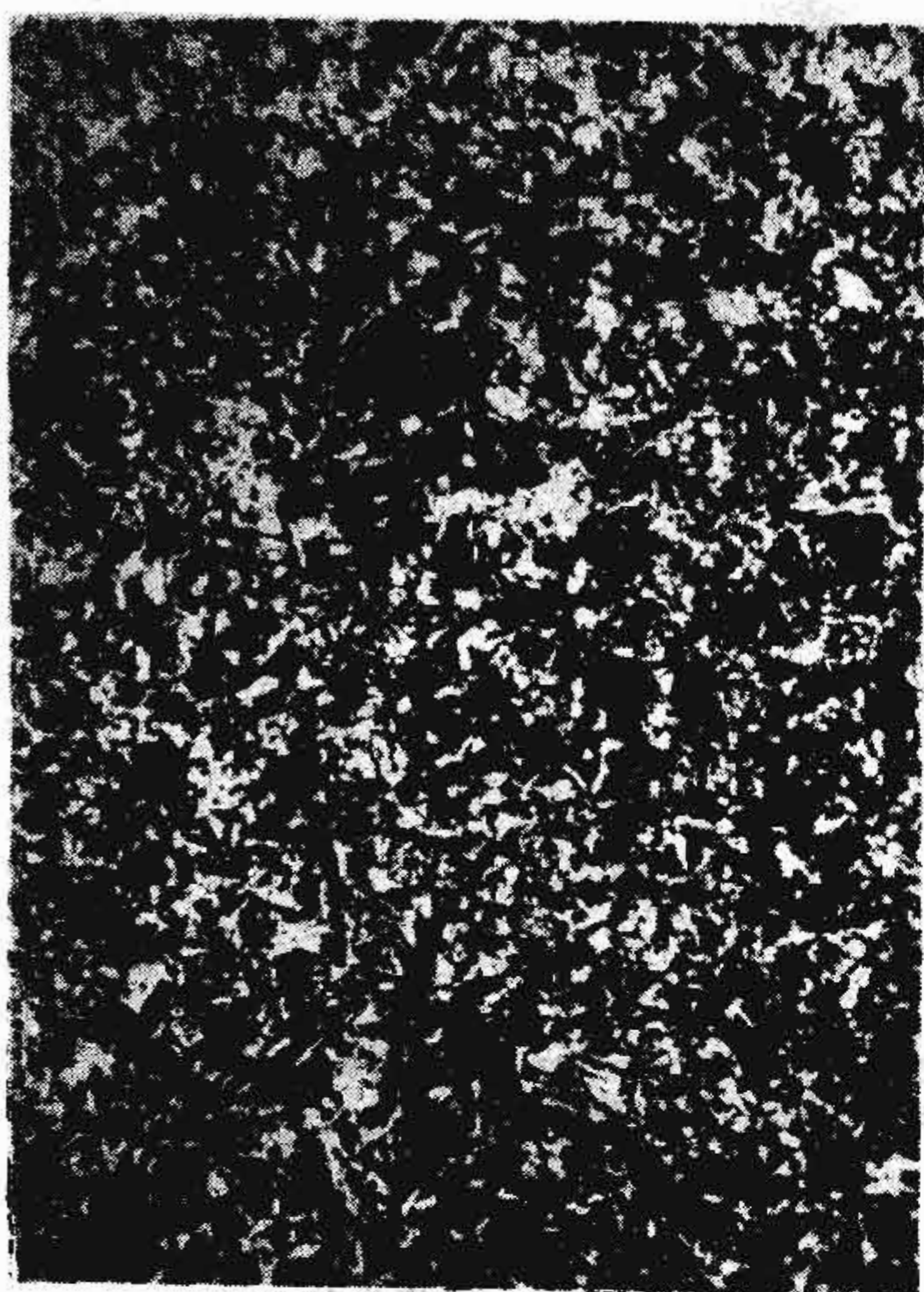
第 3 级 (少量细条状及小块状游离铁素体)
