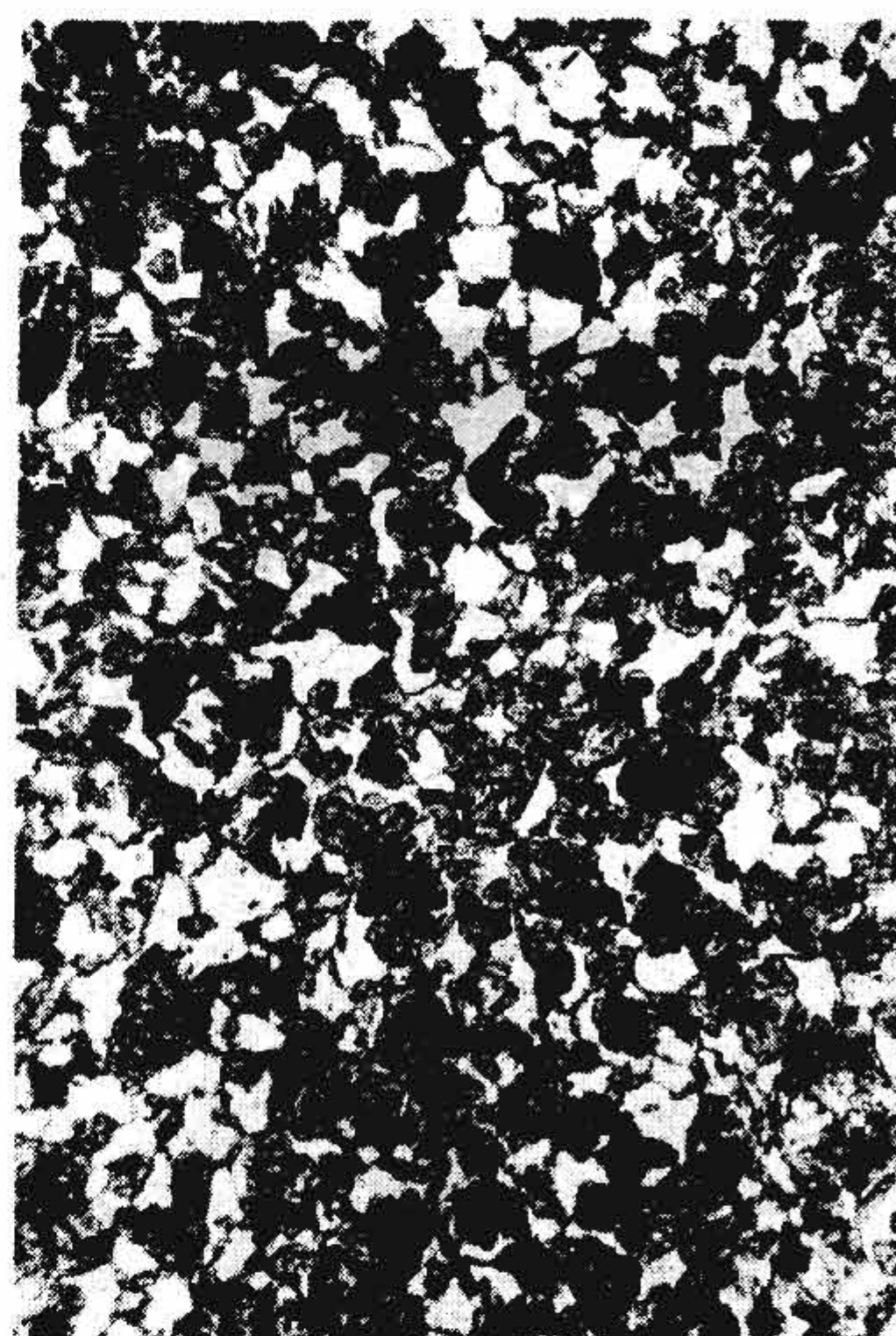
第 8 级 (大量的块状铁素体)
