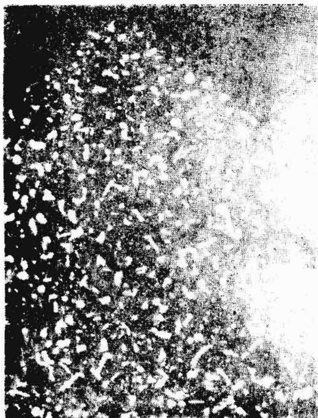
第 5 级 (碳化物呈较大块状、个别处呈断续网状分布)
