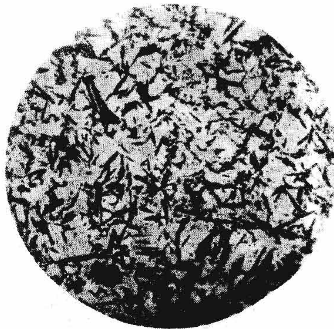
第 6 级 (粗针状马氏体, 针的长度 >8\sim 12\text{ mm} )
