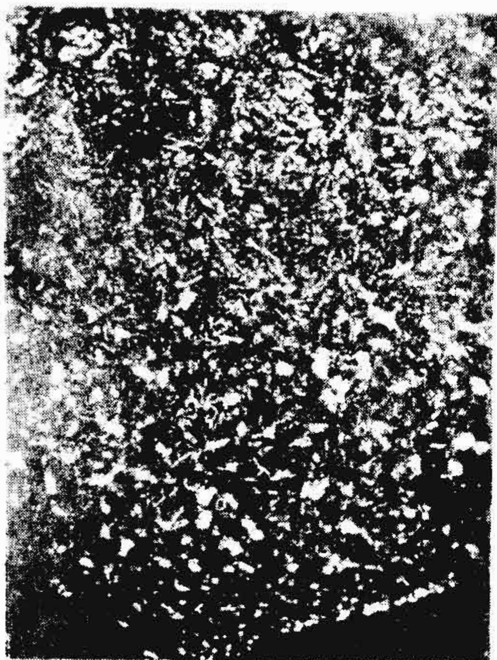
第 3 级 (碳化物呈细小块状、均匀分布)
