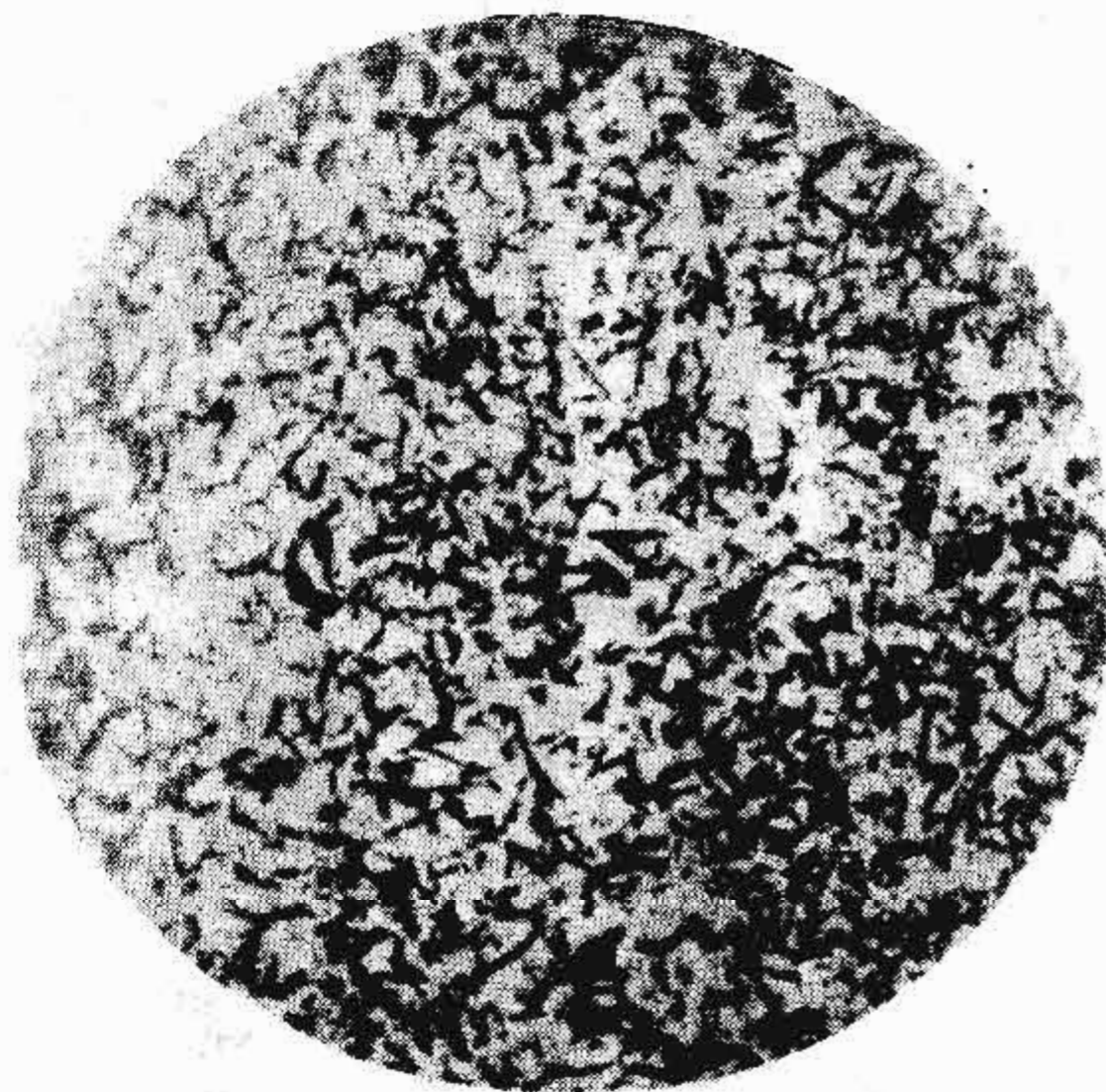
第 4 级 (针状马氏体, 针的长度 > 4 \sim 6 mm)
