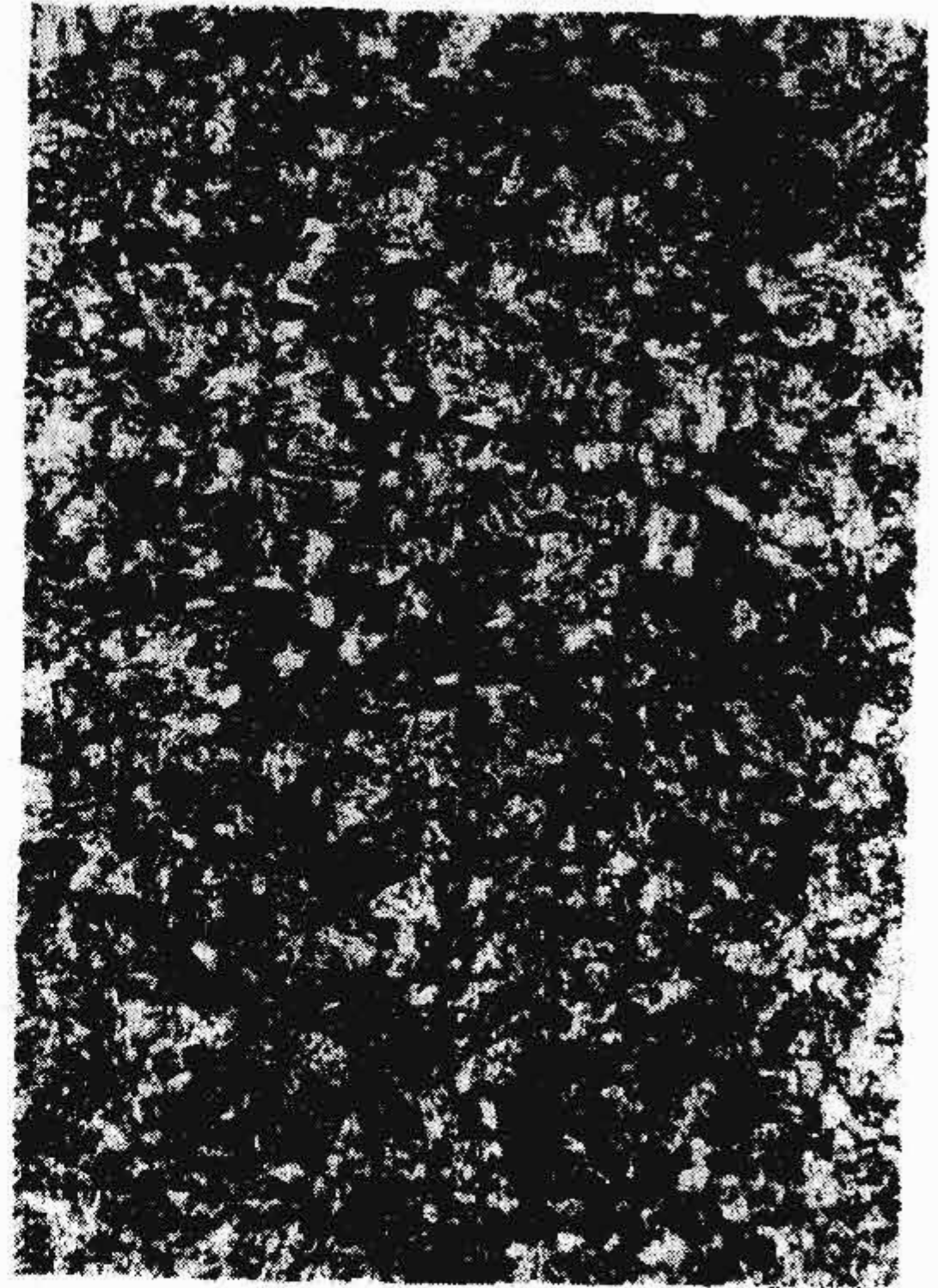
第 2 级 (微量游离铁素体)
