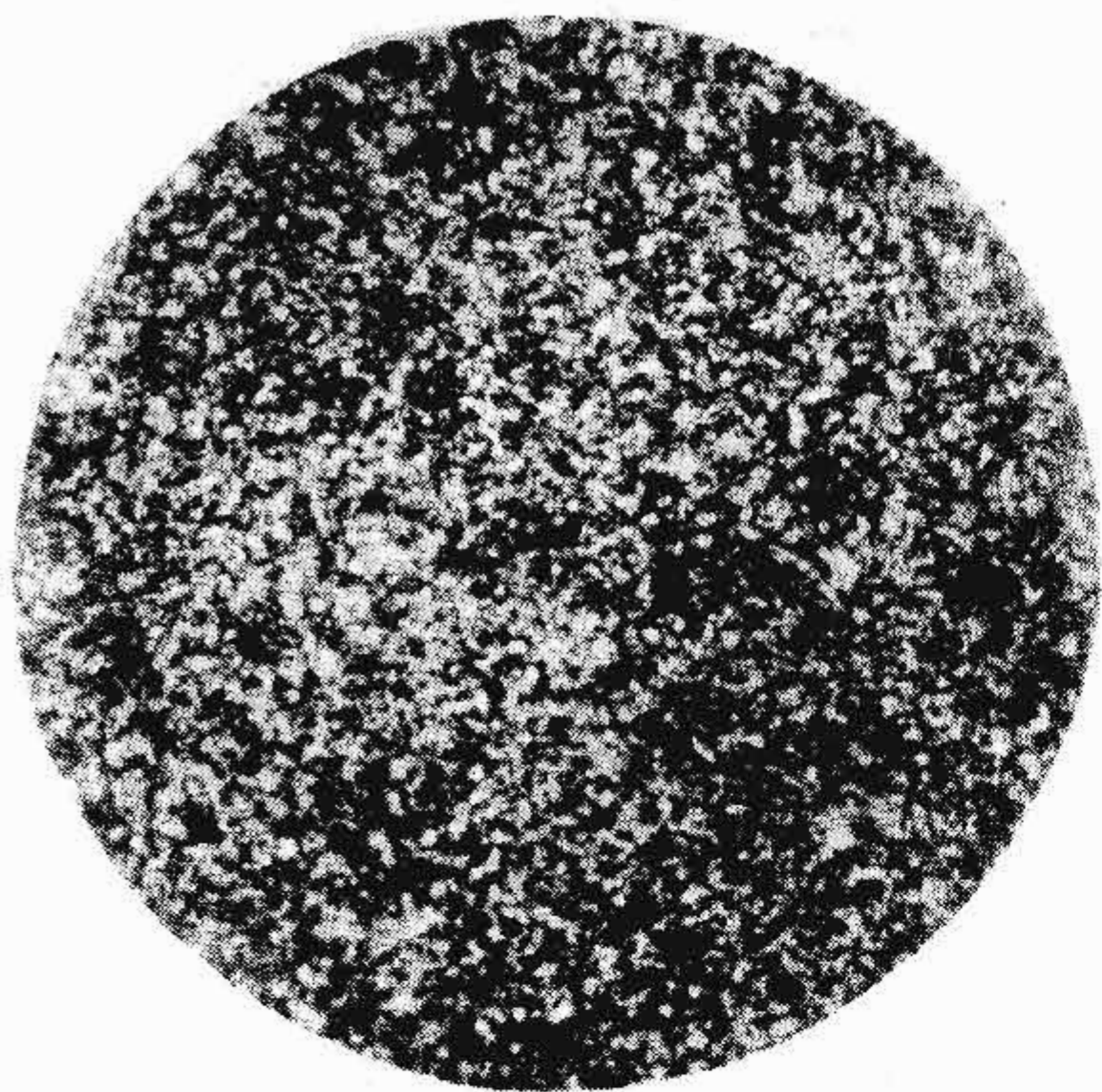
第 1 级 (细针状马氏体, 针的长度 \leq 1.5 mm)
