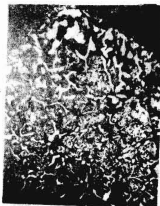
第 8 级 (碳化物呈粗大网状分布)
