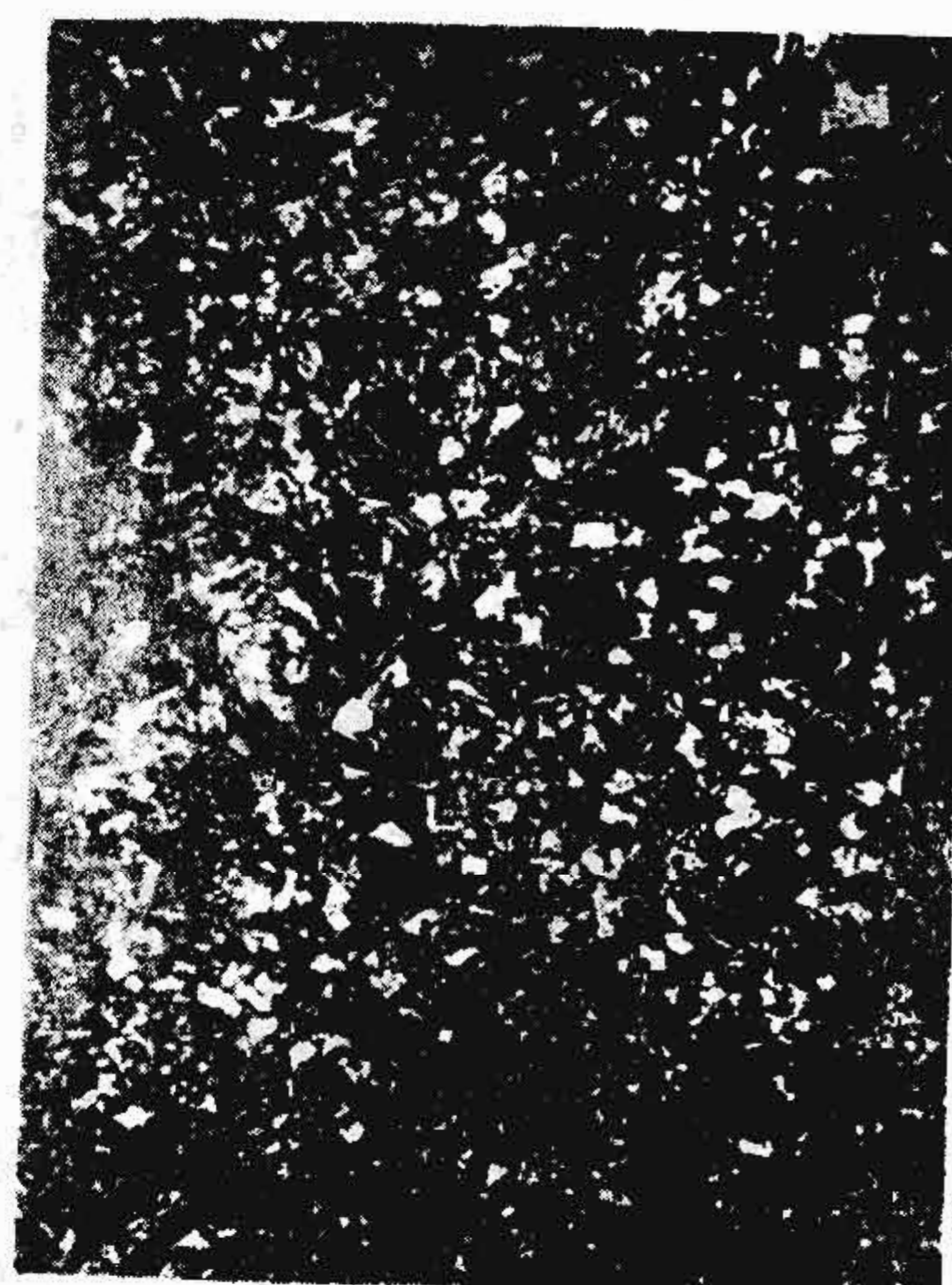
第 6 级 (较多数量的块状及条状游离铁素体)
