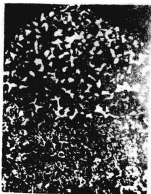
第 7 级 (碳化物呈连续网状分布)
