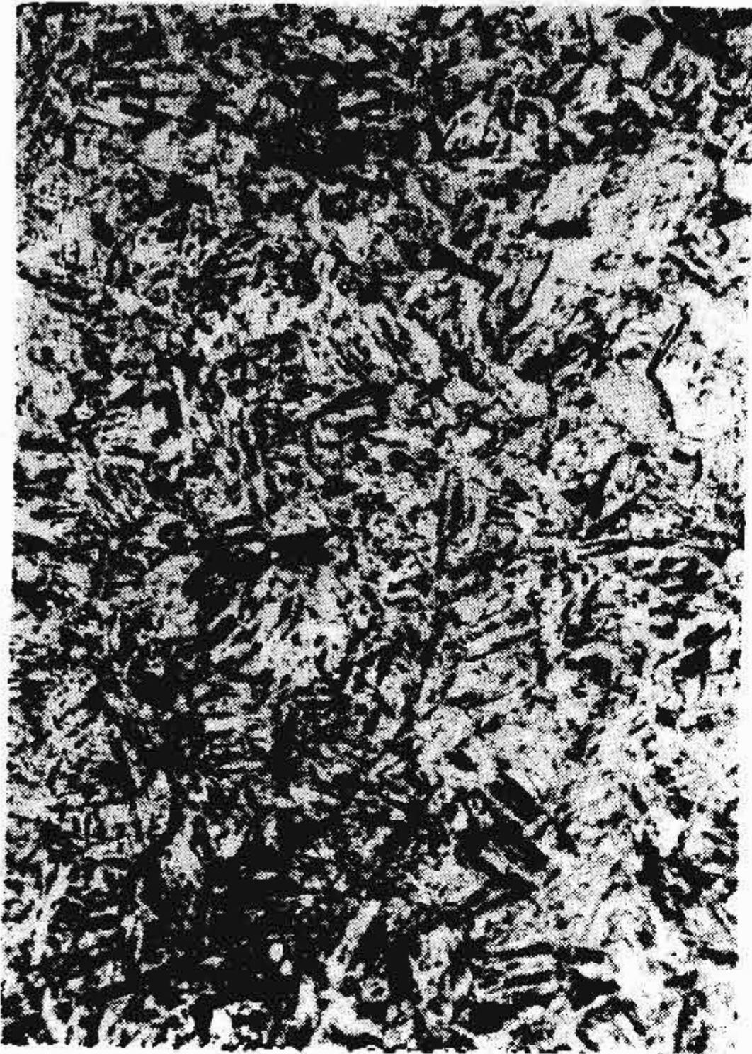
第 1 级 (无明显游离铁素体)
