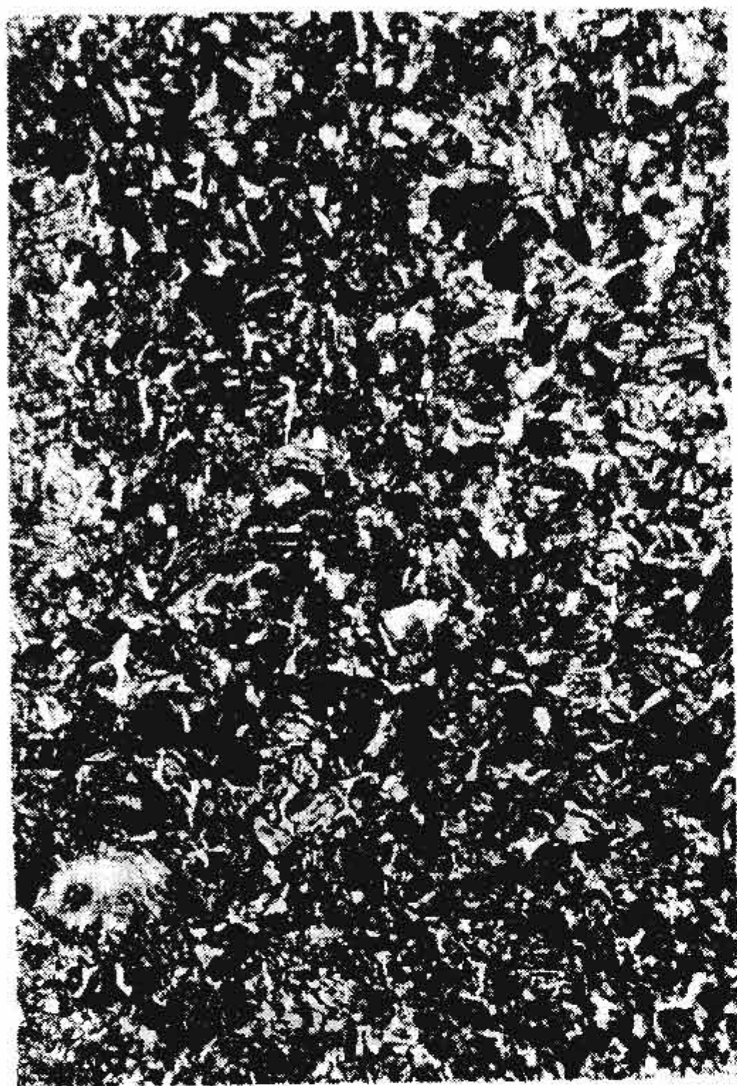
第 5 级 (条状及块状游离铁素体)
