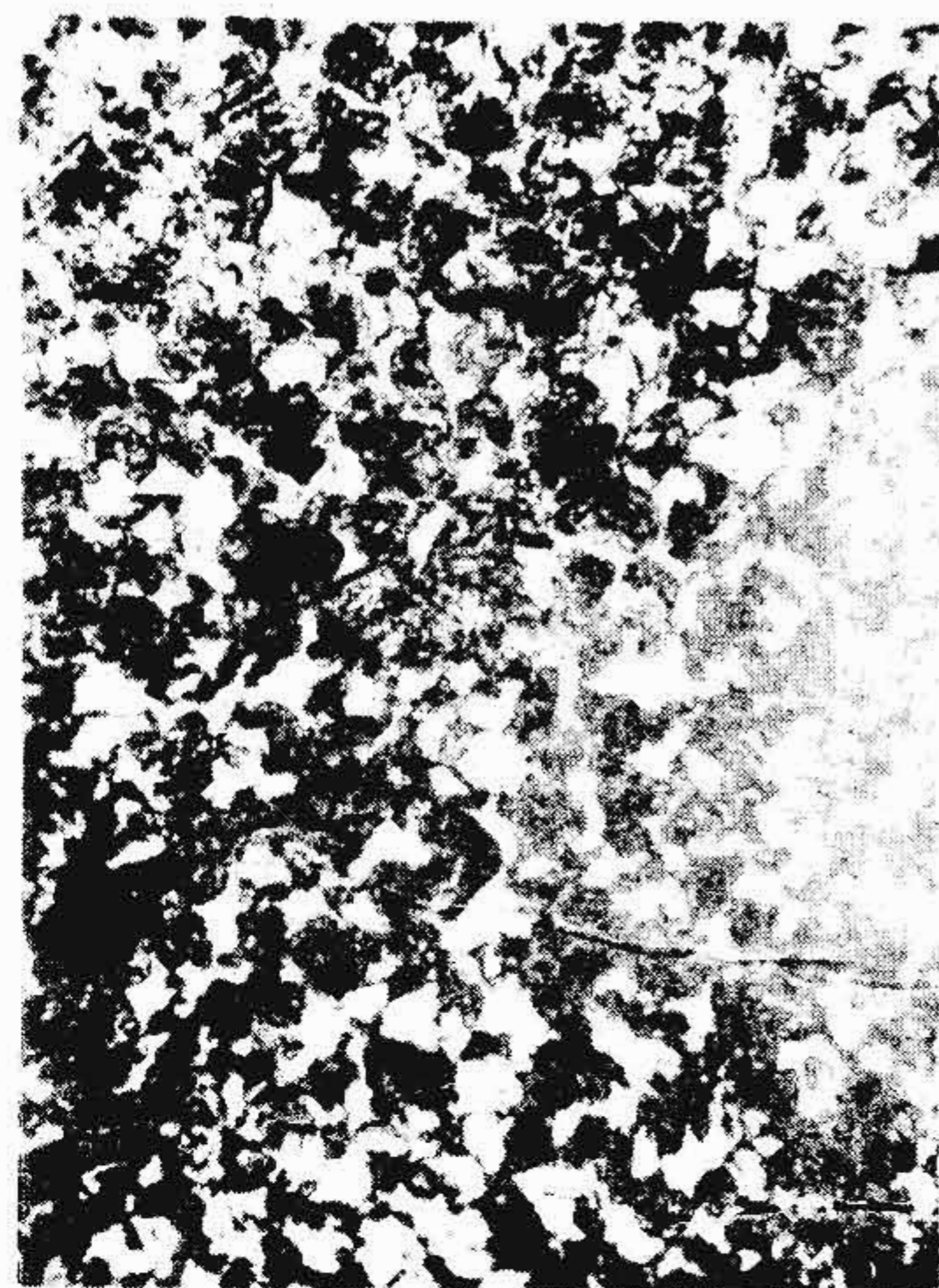
第 8 级 (大量的块状铁素体)
