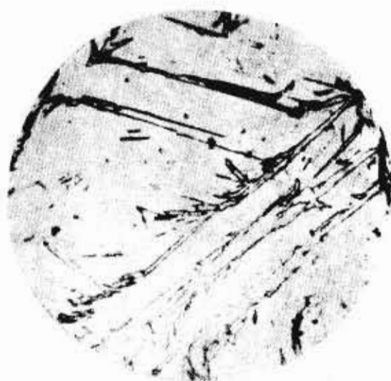
第 10 级 (粗针马氏体, 针的长度 >50 \text{ mm} )
