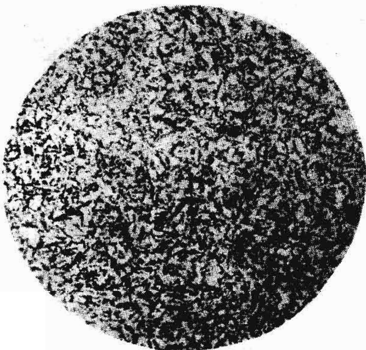
第 3 级 (针状马氏体, 针的长度 > 2.5 \sim 4 mm)
