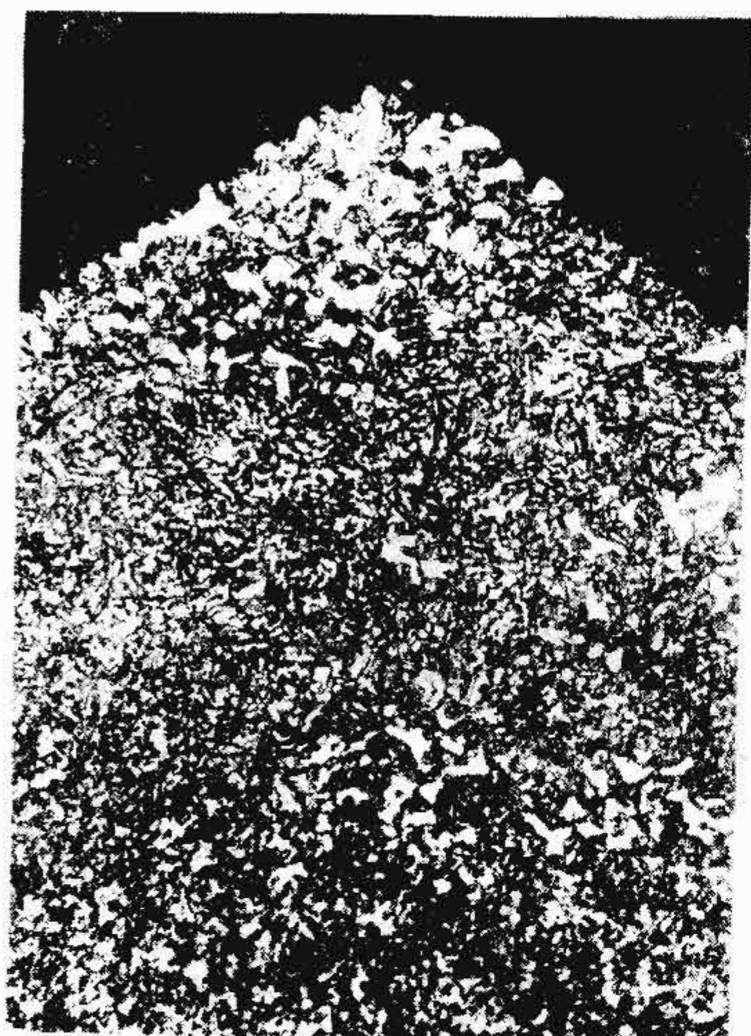
第 5 级 (块状碳氮化合物, 较偏析分布)
