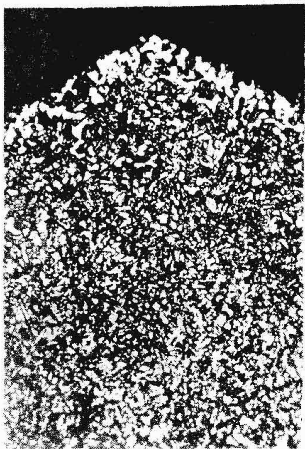
第 5 级 (块状碳氮化合物, 较集中分布)
