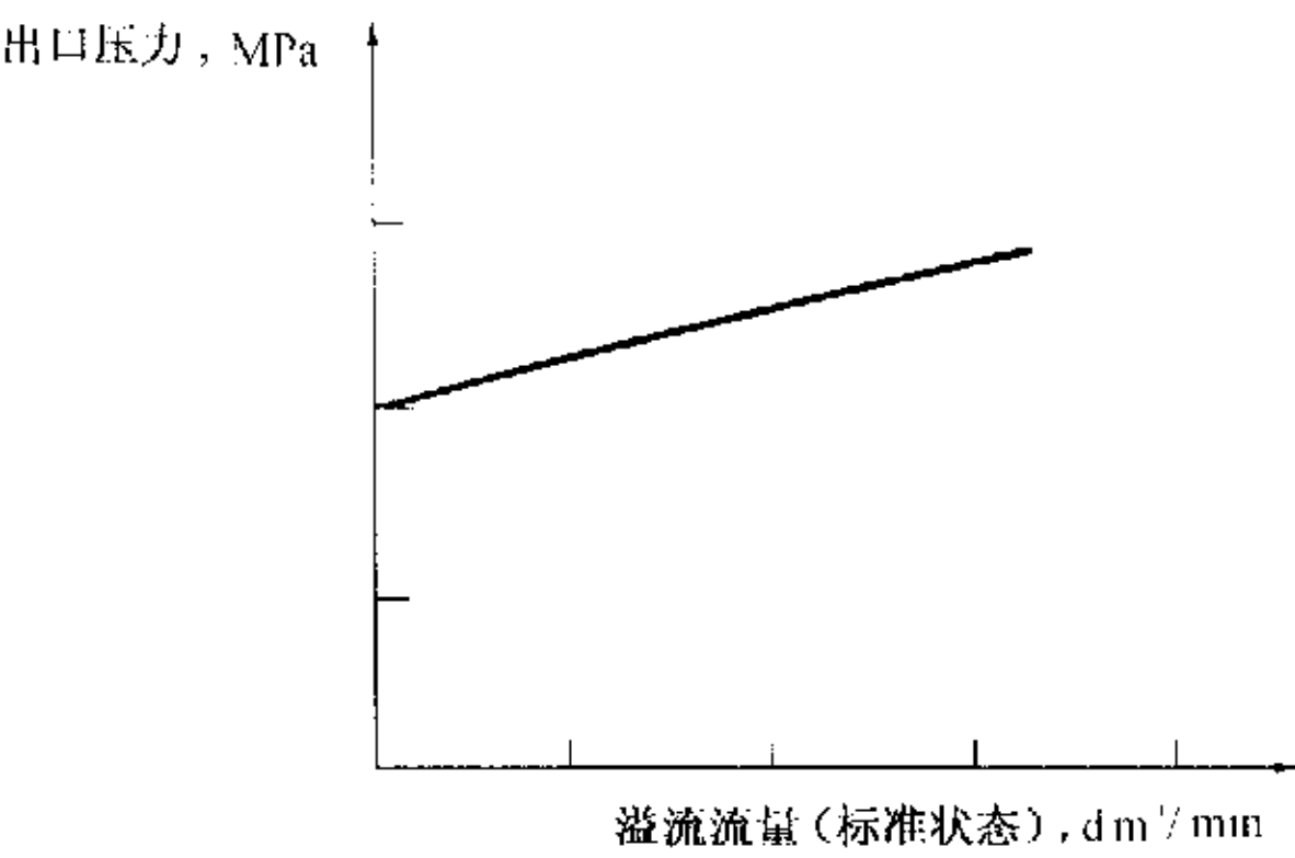
图 3 溢流特性曲线
