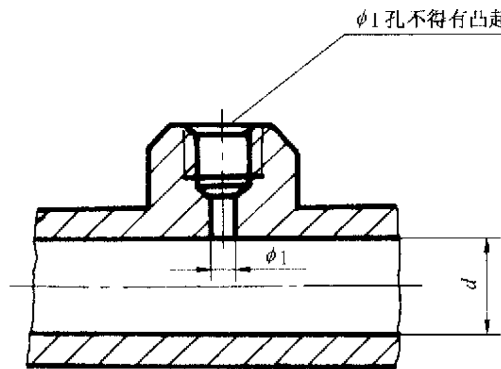
图 5 取压孔结构图
