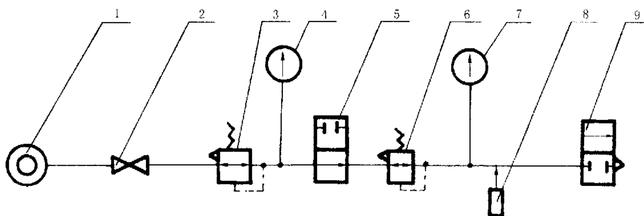
1—气源;2—截止阀;3—空气减压阀;4、7—压力表; 5、9—二位三通阀(可用机、电、气控);6—被测空气减压阀;8—计数器
