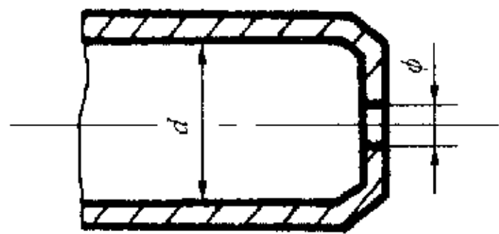
图 6 恒节流孔结构
